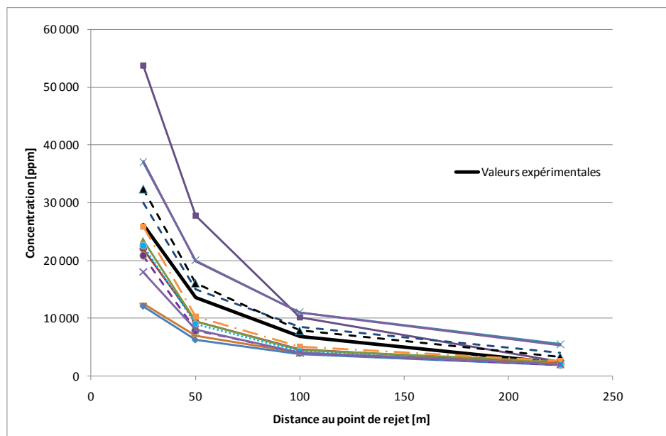
Figure 17 : Evolution de la concentration en CO_2 en fonction de la distance dans l'axe du rejet.
