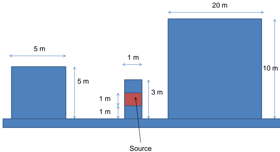
Figure 35 : Coupe A-A.
