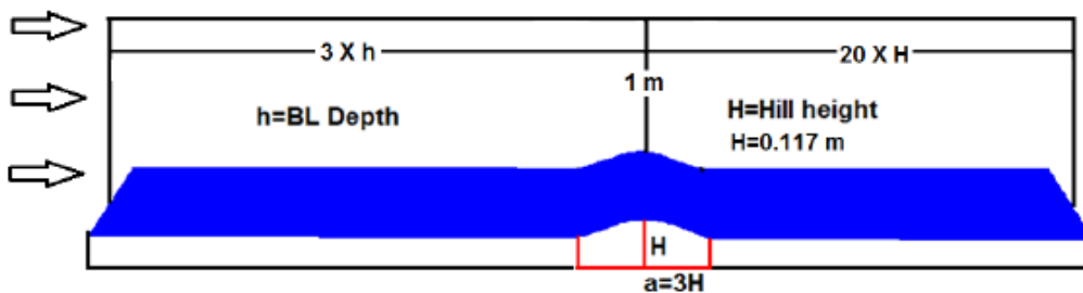
Figure 54 : Vue schématique de l'expérience de Khurshudyan [99].
