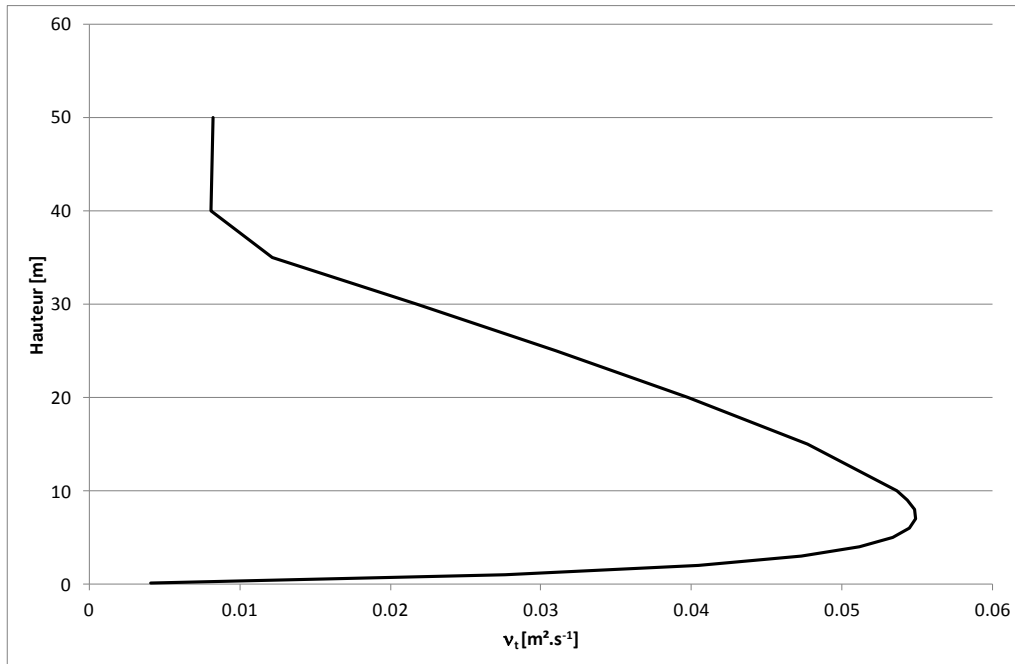
Figure 21 : Exemple de forme de viscosité turbulente.
