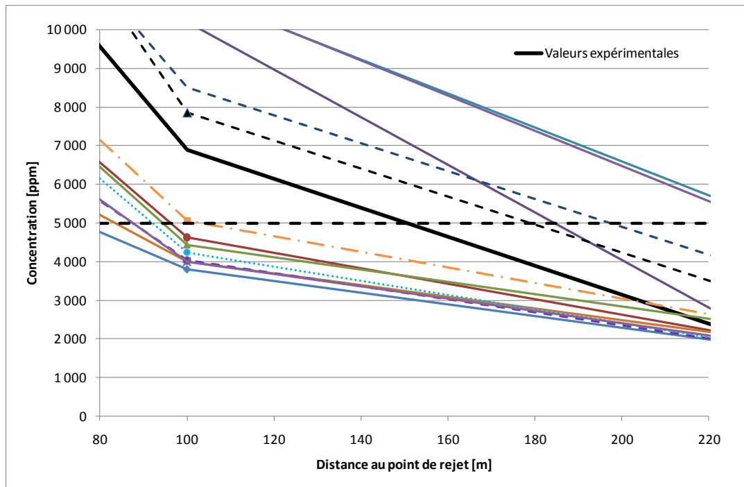
Figure 18 : Relation concentration, distance d'effets, zoom sur la courbe de la Figure 17 pour des valeurs de concentration de 5 000 ppm.
