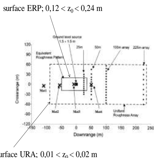
Figure 15 : Vue générale schématique de la configuration expérimentale. ERP : Equivalent Roughness Panel, zone de rugosité de 0,12 à 0,24 m - URA : Uniform Roughness Area, zone de rugosité de 0,01 à 0,02 m.
