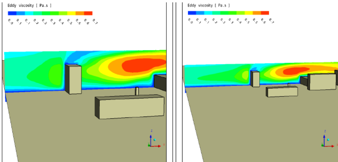
Figure 46 : Champ de viscosité turbulente dans un plan horizontal sans (gauche) et avec (droite) extrusion du maillage.
