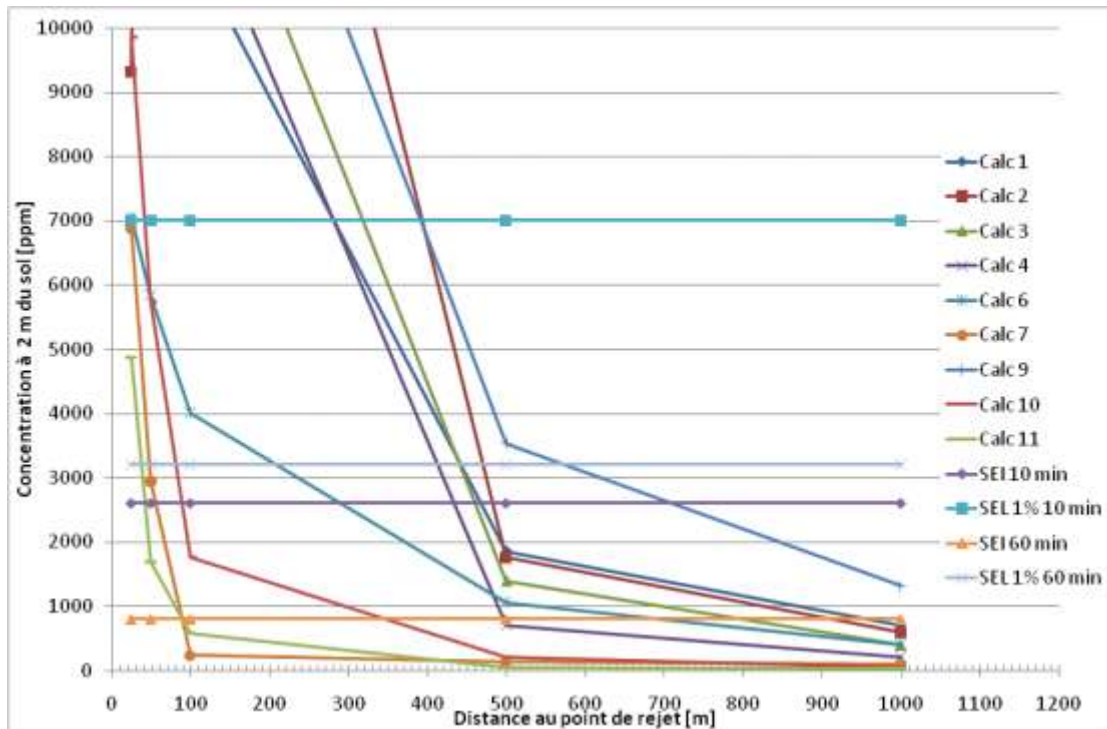
Figure 13 : Distances d'effet obtenues par les différentes modélisations.
