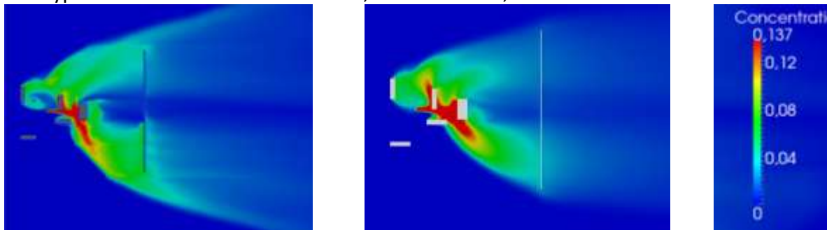
Figure 41 : Résultats obtenus sans (gauche) et avec (droite) modélisation de la physique de l'atmosphère, champ de concentration en C_3H_8 .
