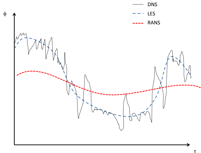
Figure 8 : Représentation schématique de l'évolution d'une grandeur physique au cours du temps selon les différentes modélisations de la turbulence.
