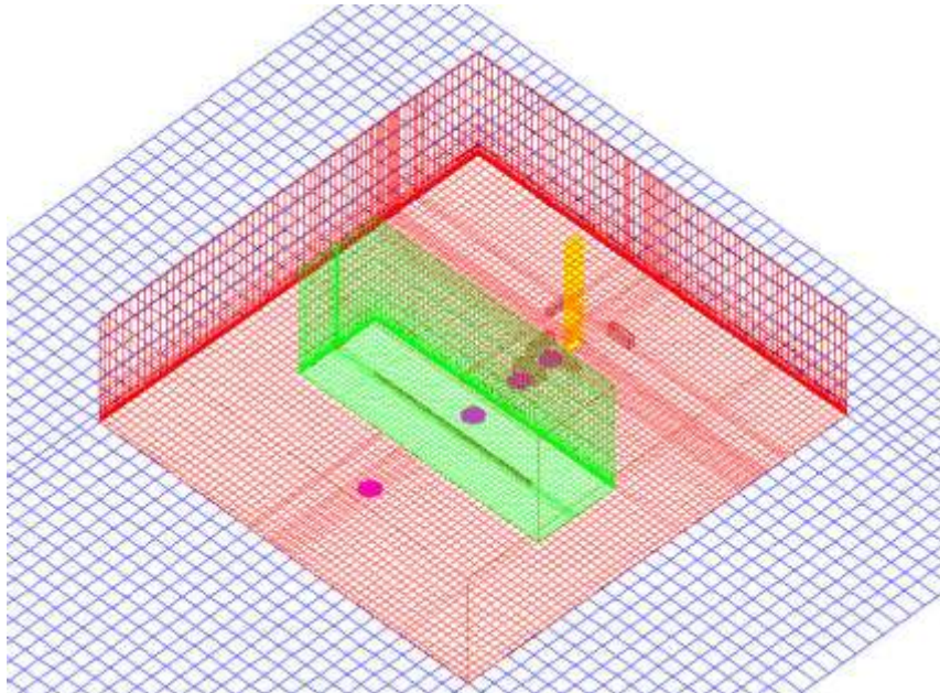
Figure 30 : Exemple de maillages imbriqués.
