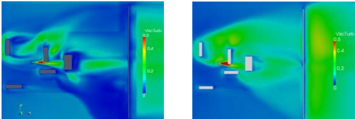
Figure 40 : Résultats obtenus sans (gauche) et avec (droite) modélisation de la physique de l'atmosphère, champ de viscosité turbulente.
