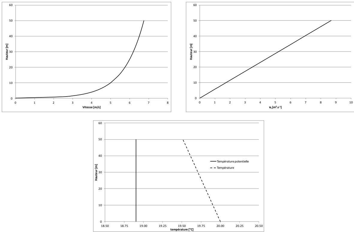
Figure 23 : Profils de vitesses, viscosité turbulente et température obtenus pour une classe de vent D5.
