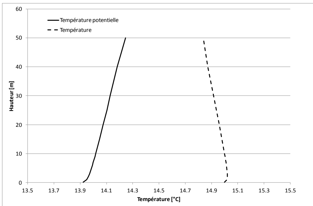
Figure 22 : Profils de température et température potentielle pour une classe de vent F3.
