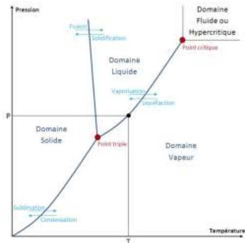
Figure 26 : Diagramme de phase d'un corps pur
