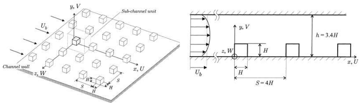
Figure 53 : Configuration étudiée par Meinders [96].
