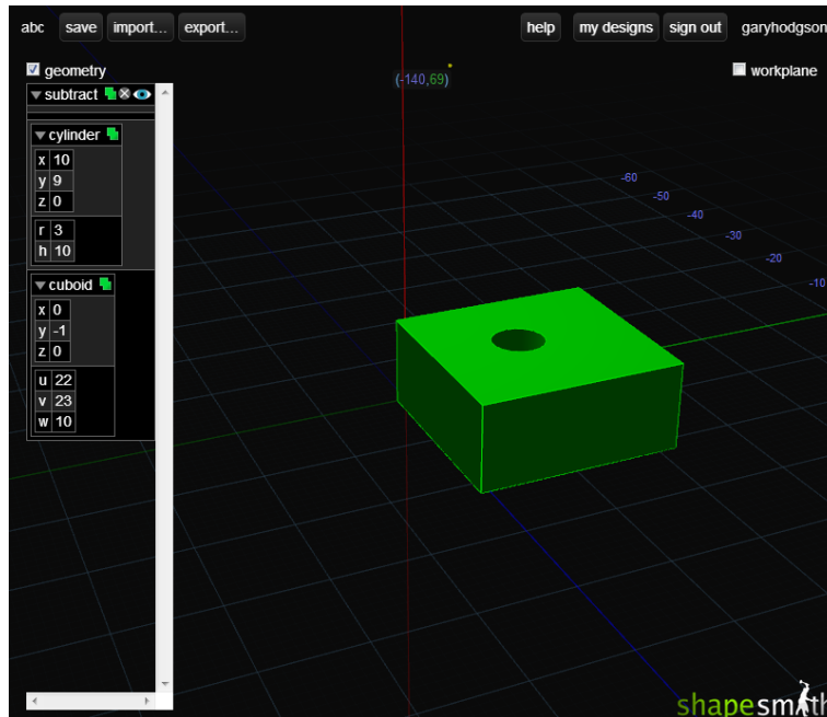
FIGURE 3.9 : Outil de CAO en ligne Shapsmith.
