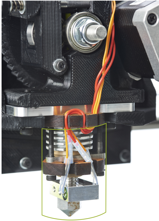
FIGURE 8.2 : Le cylindre de dégagement autour de l'extrudeuse.
