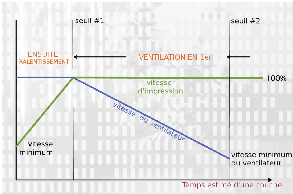
FIGURE 5.15 : Stratégie de refroidissement.
