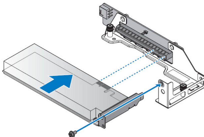
Figure 133. Installation de la carte NPIO dans un support
