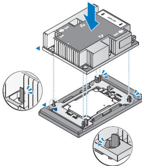
Figure 19. Insertion du dissipateur de chaleur dans un assemblage de plateau de processeur
