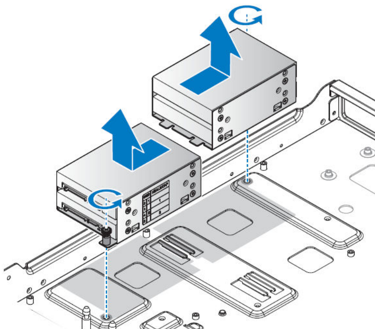
Figure 28. Retrait de l'assemblage de disque dur de 2,5 pouces
