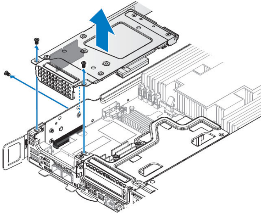
Figure 66. Retrait de l'assemblage mini-PERC
