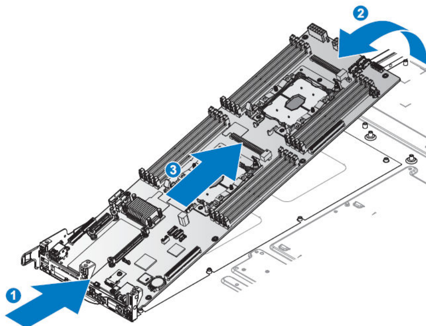
Figure 43. Retrait de la carte serveur
