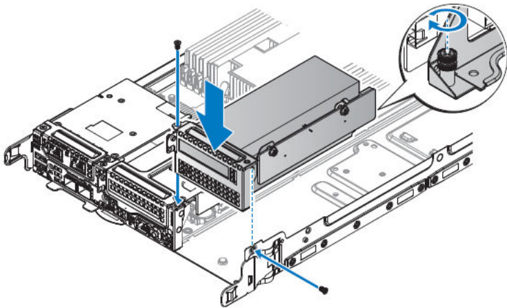
Figure 141. Installation de l'assemblage de la carte NPIO
