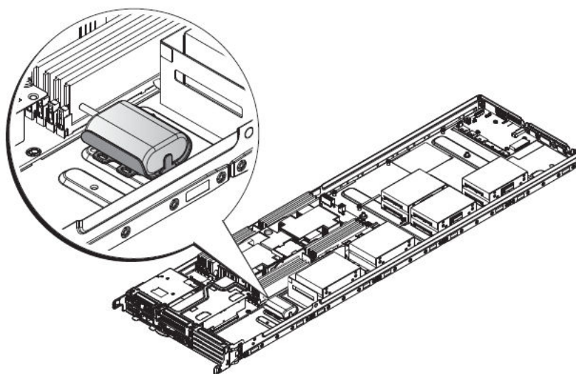
Figure 52. Localisation du supercondensateur
