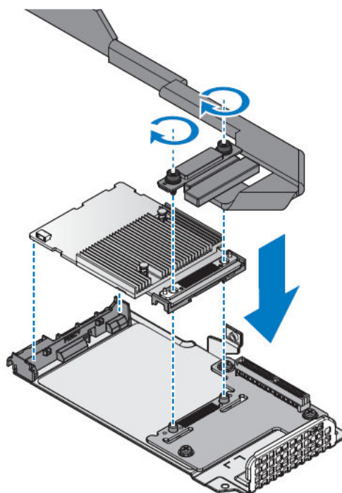
Figure 71. Assemblage de la carte de mini-adaptateur PERC et du câble sur le support
