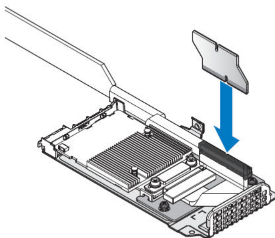
Figure 72. Installation de la carte-pont sur l'assemblage du mini-adaptateur PERC
