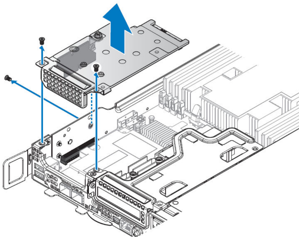
Figure 82. Retrait de l'assemblage SATA M.2
