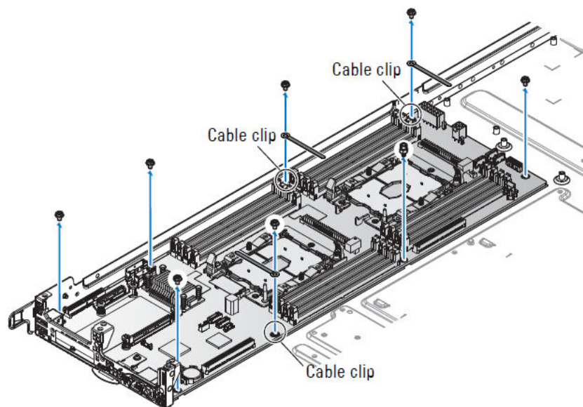
Figure 42. Retrait des vis de fixation de la carte serveur
