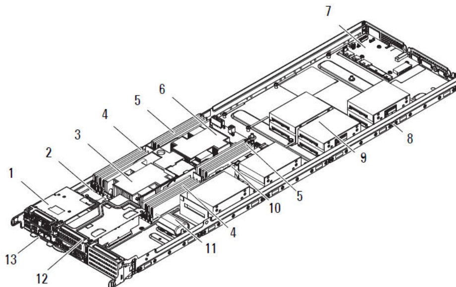
Figure 1. Serveur DSS 9620 2,5 pouces demi-largeur
