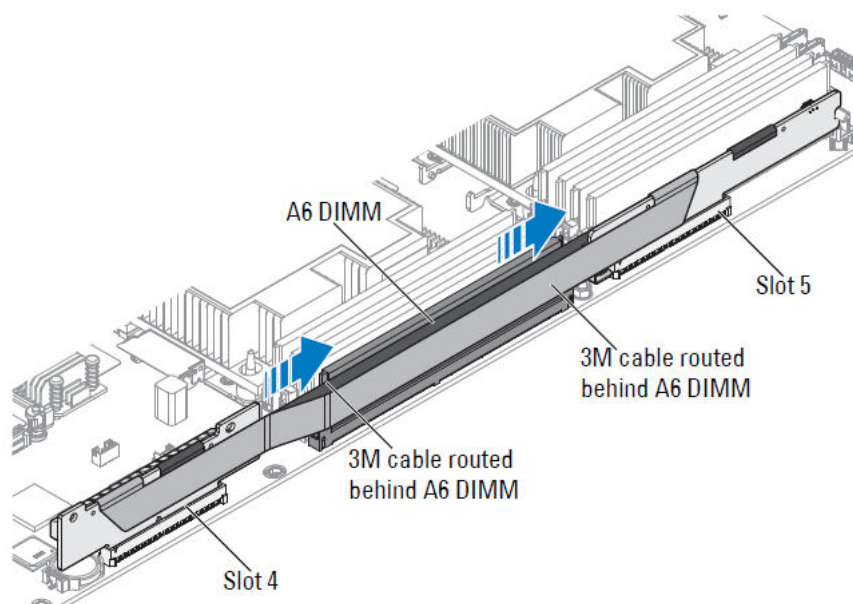
Figure 124. Présentation de l'acheminement des câbles
