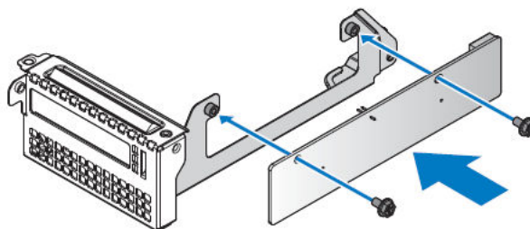
Figure 139. Installation de la carte de montage sur un support
