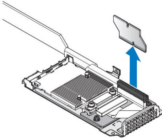
Figure 67. Retrait de la carte-pont de l'assemblage mini-PERC.
