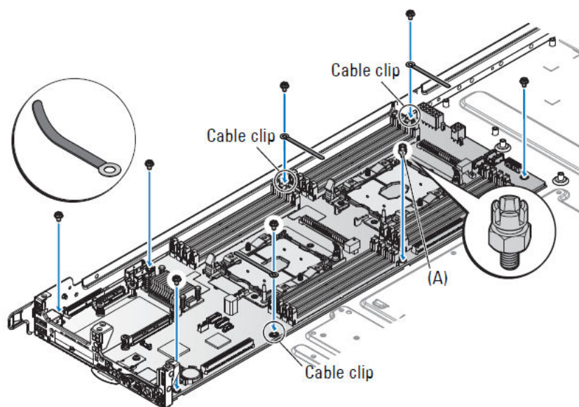
Figure 45. Fixation de la carte serveur
