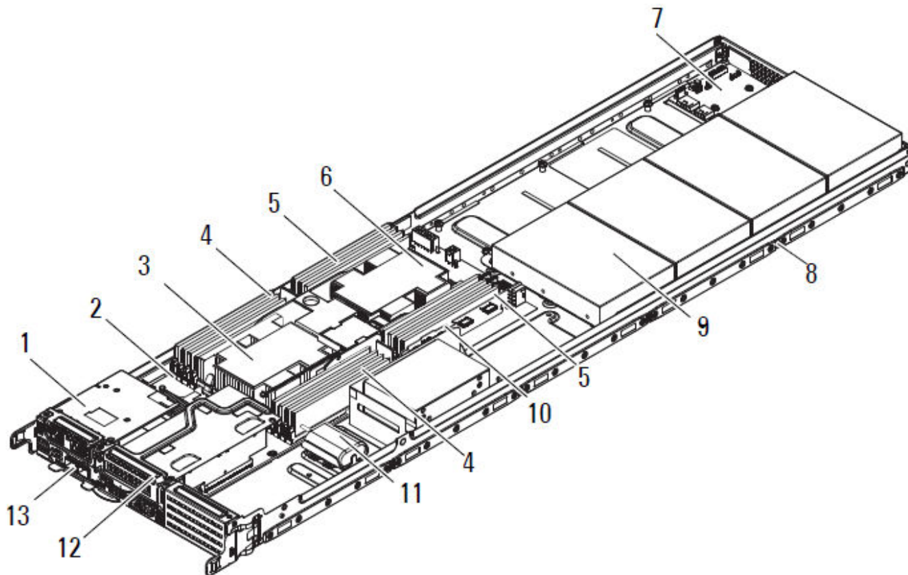
Figure 2. Serveur DSS 9620 3,5 pouces demi-largeur
