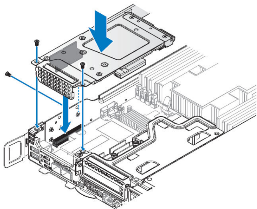
Figure 73. Installation de l'assemblage du mini-adaptateur PERC
