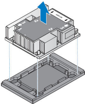
Figure 20. Retrait de l'assemblage du processeur du plateau de processeur
