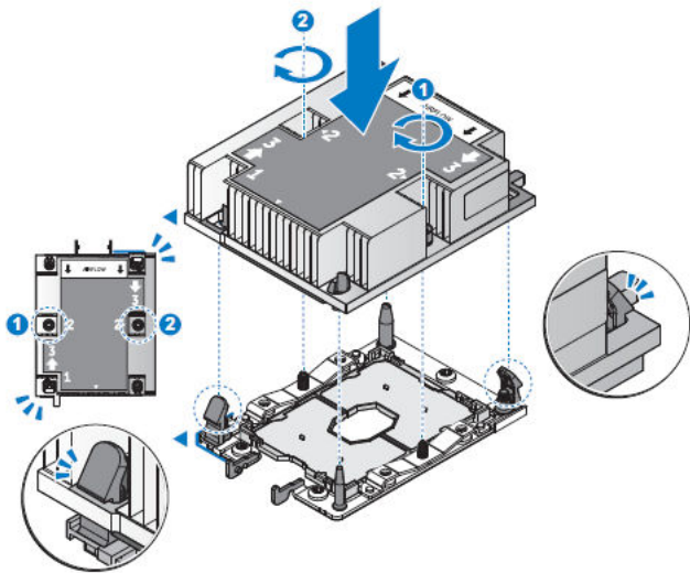
Figure 21. Installation de l'assemblage du processeur
