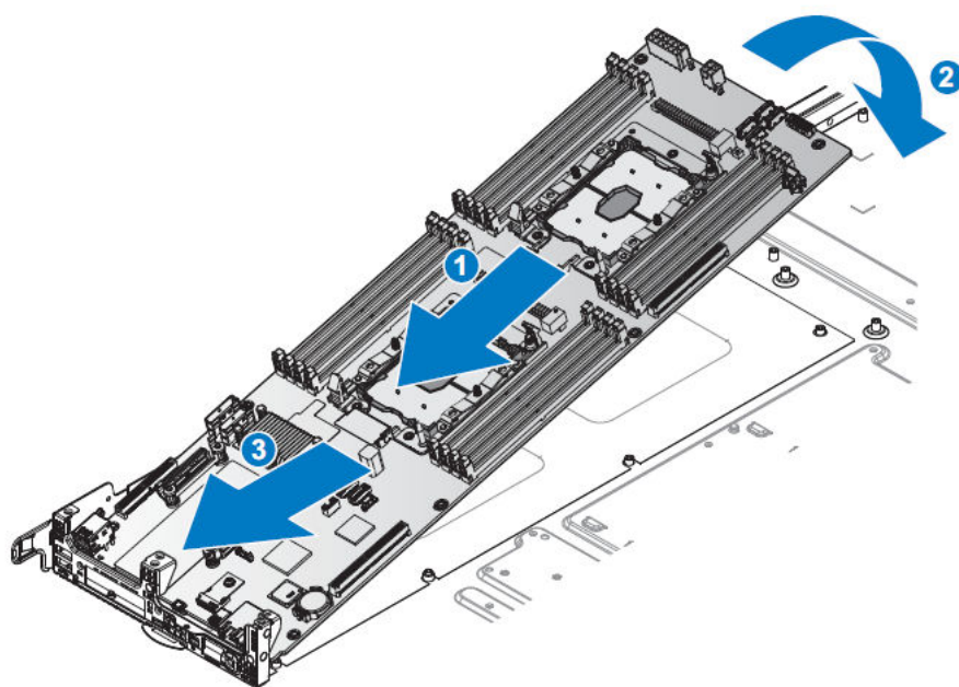
Figure 44. Installation de la carte serveur
