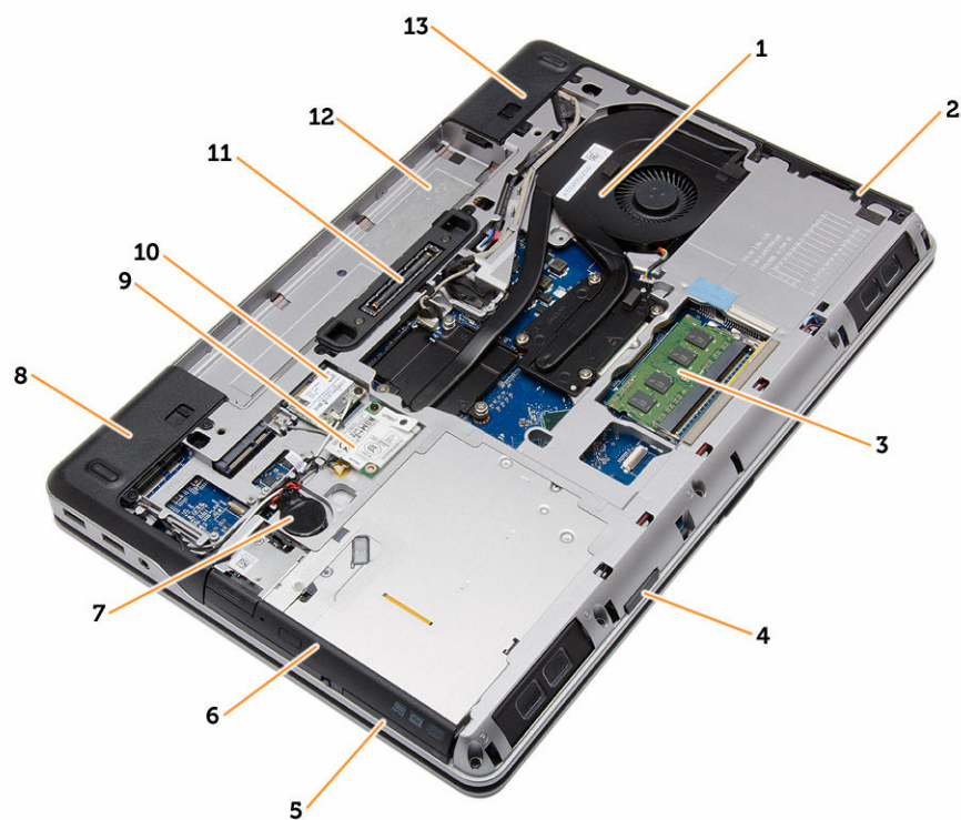
Figure 1. Vue arrière - Capot arrière retiré
