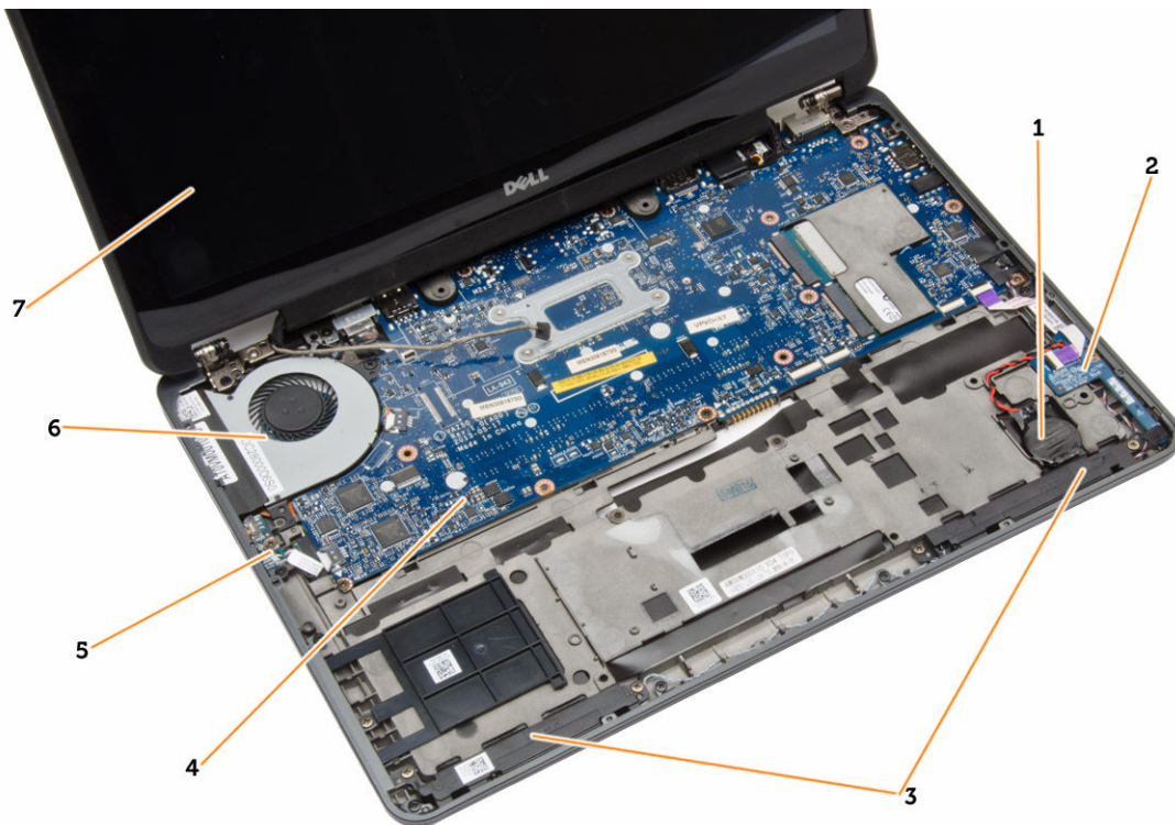
Figure 2. Vue interne – Avant
