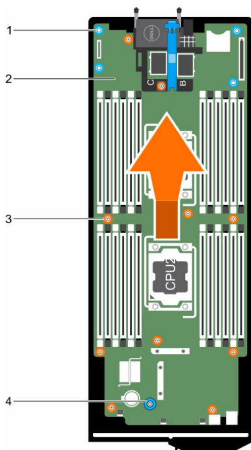
Figure 60. Retrait de la carte système
