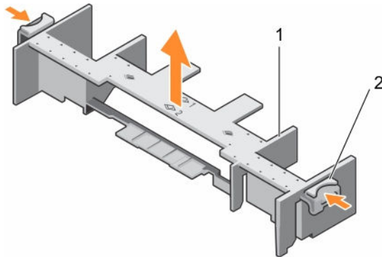
Figure 11. Retrait d'un carénage de refroidissement
