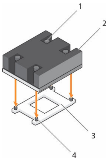
Figure 34. Installation d'un dissipateur de chaleur
