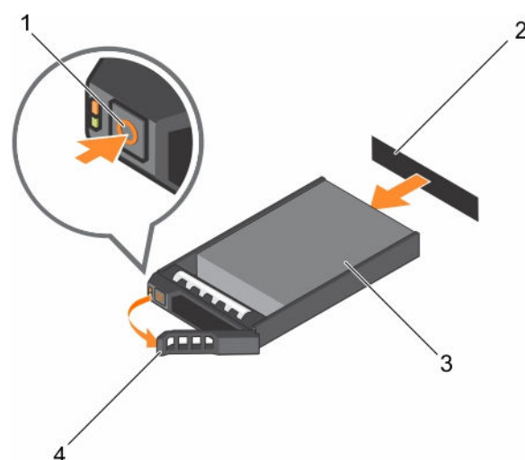
Figure 38. Retrait d'un disque dur
