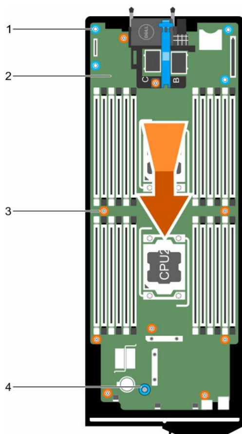
Figure 61. Installation de la carte système
