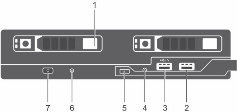
Figure 2. Fonctions du panneau avant (système de disque dur/SSD de 2,5 pouces)
