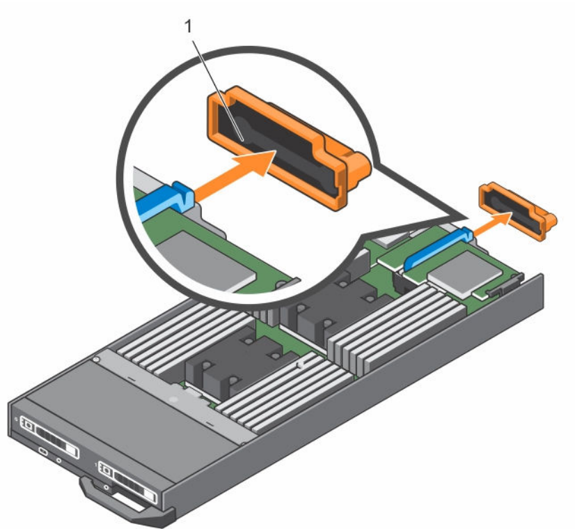
Figure 7. Retrait du capot des connecteurs d'E/S
