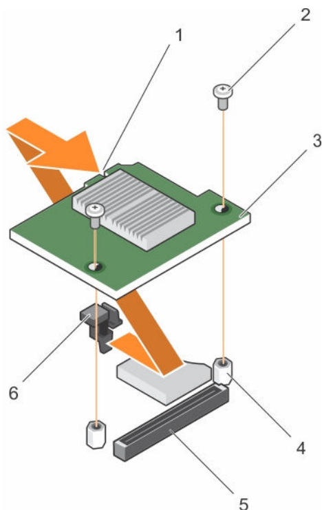
Figure 29. Retrait de la carte fille réseau
