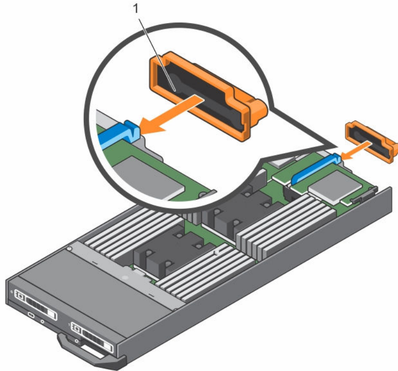
Figure 9. Installation du traîneau
