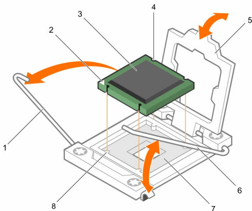
Figure 33. Installation et retrait d'un processeur
