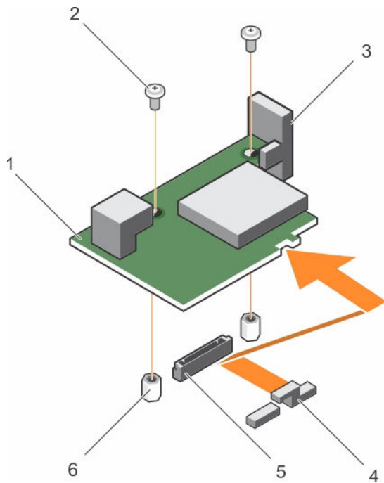
Figure 23. Retrait de la carte IDSDM en option
