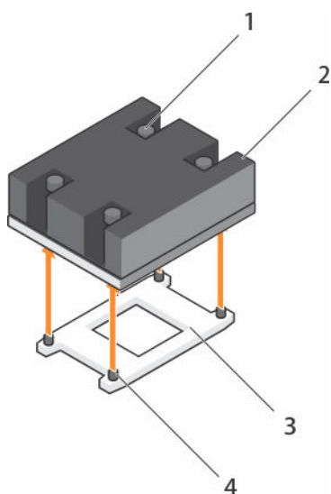
Figure 31. Retrait d'un dissipateur de chaleur
