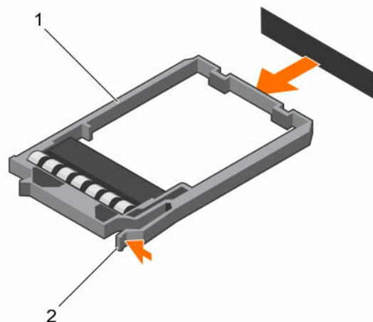
Figure 43. Retrait d'un cache de SSD de 1,8 pouce
