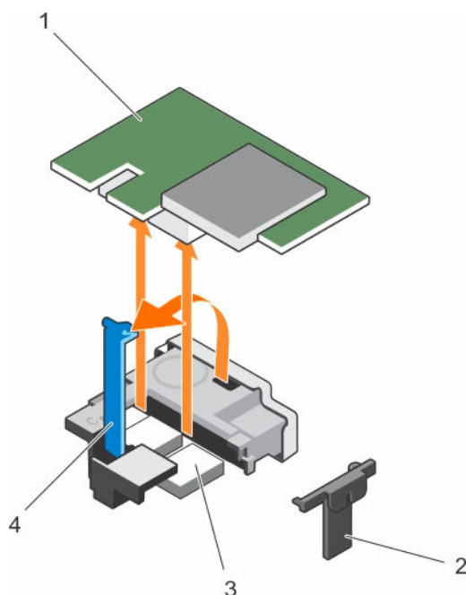
Figure 18. Retrait d'une carte mezzanine PCIe
