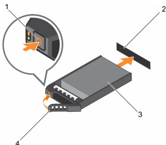
Figure 40. Installation d'un disque dur
