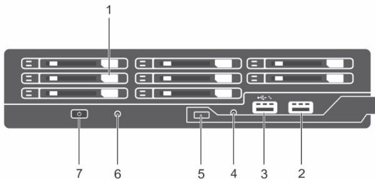
Figure 3. Fonctions du panneau avant : système SSD de 1,8 pouce
