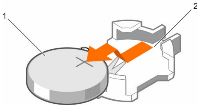
Figure 58. Retrait de la pile de secours de la NVRAM
