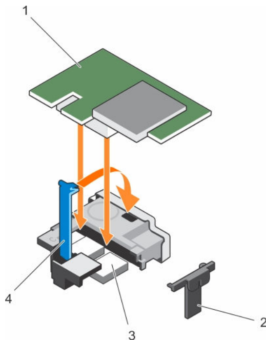
Figure 19. Installation d'une carte mezzanine PCIe
