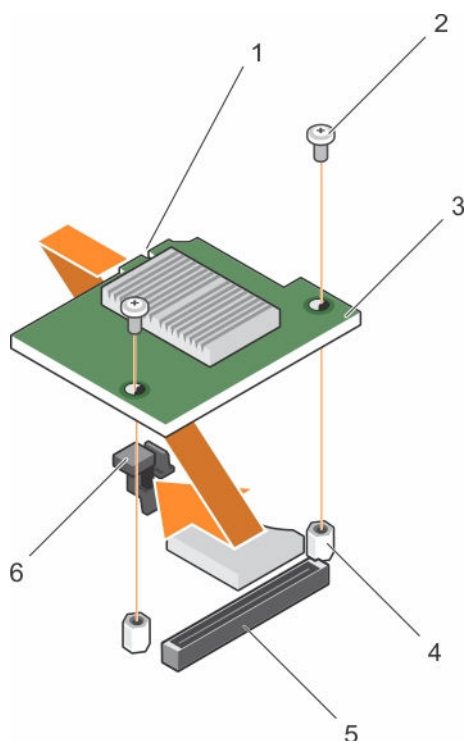
Figure 30. Installation de la carte fille réseau
