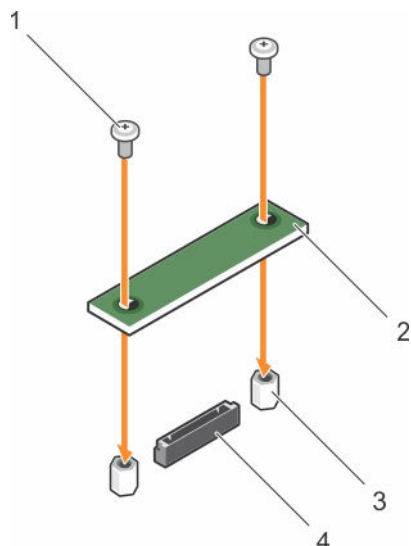
Figure 26. Installation de la carte rSPI en option
