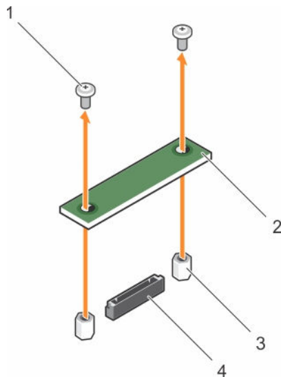
Figure 25. Retrait de la carte sSPI en option
