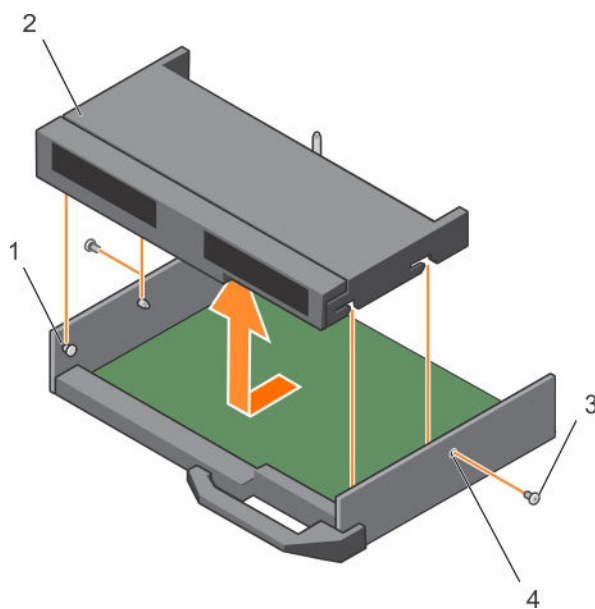
Figure 50. Retrait d'un bâti de disque dur/SSD
