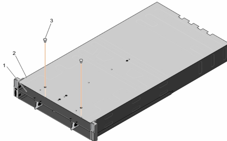
Figure 54. Retrait et installation des vis fixant le module intercalaire supérieur à la plaque du milieu
