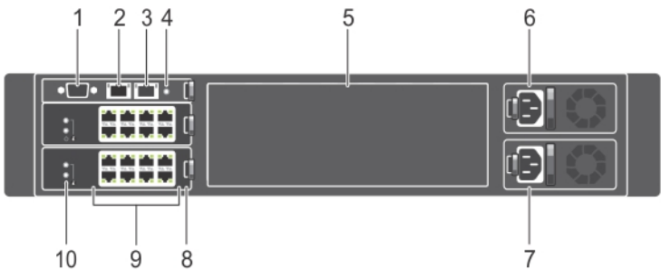
Figure 8. Voyants et caractéristiques du panneau arrière – PowerEdge FX2
