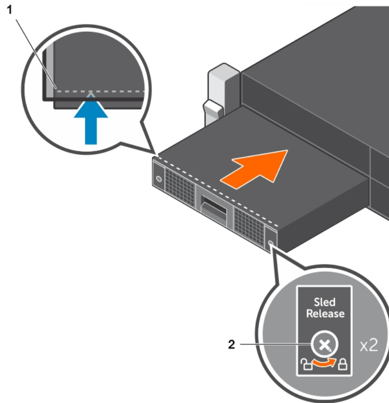
Figure 35. Installation d'un traîneau de stockage
