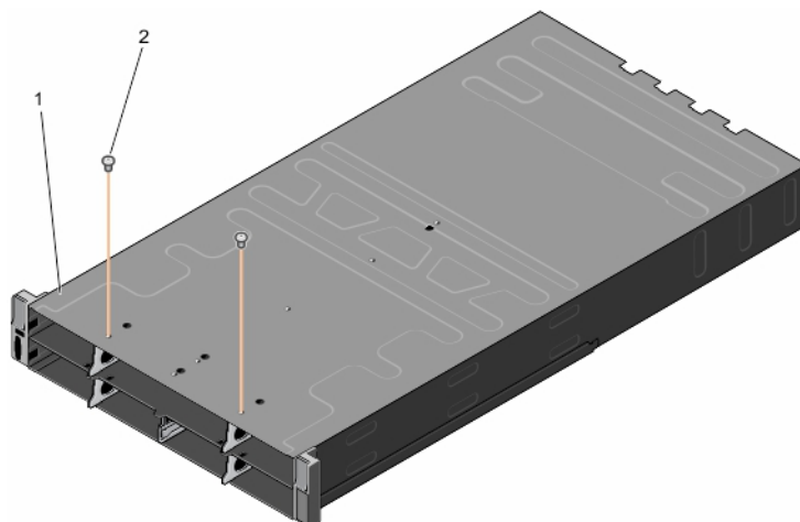
Figure 50. Retrait et installation des vis fixant le module intercalaire inférieur
