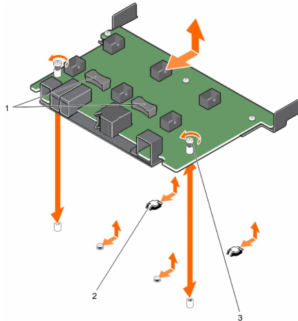
Figure 47. Retrait et installation de la carte d'interface des ventilateurs
