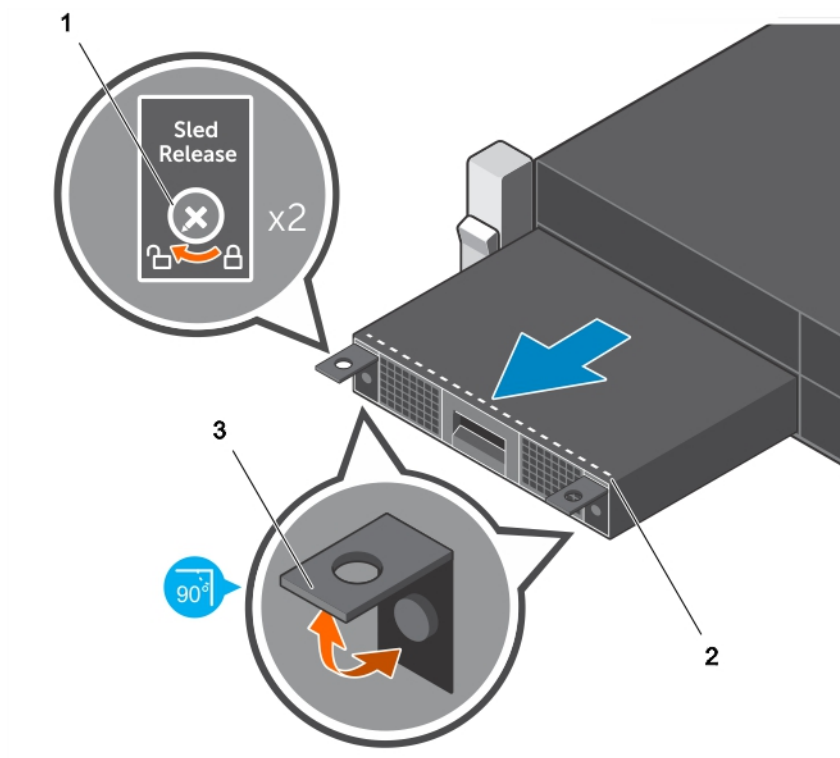
Figure 33. Retrait d'un traîneau de stockage
