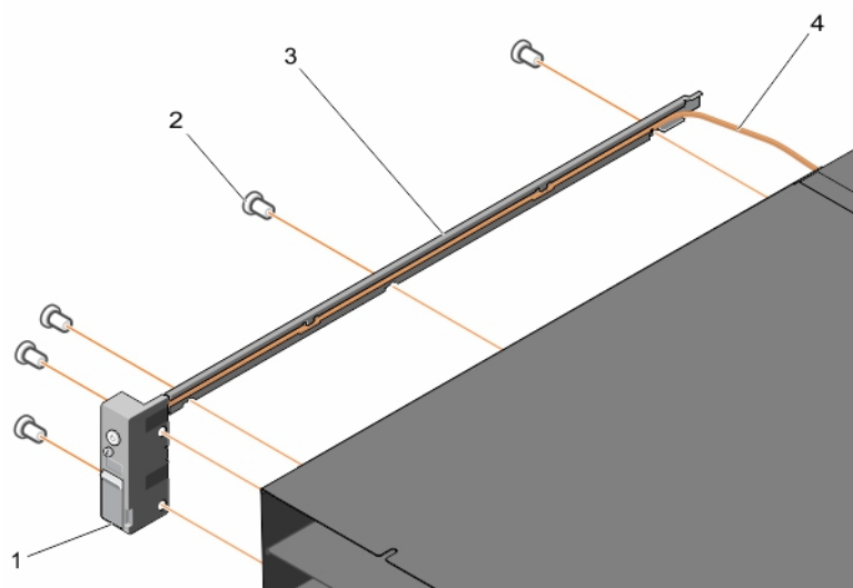
Figure 62. Retrait et installation de la gaine du câble
