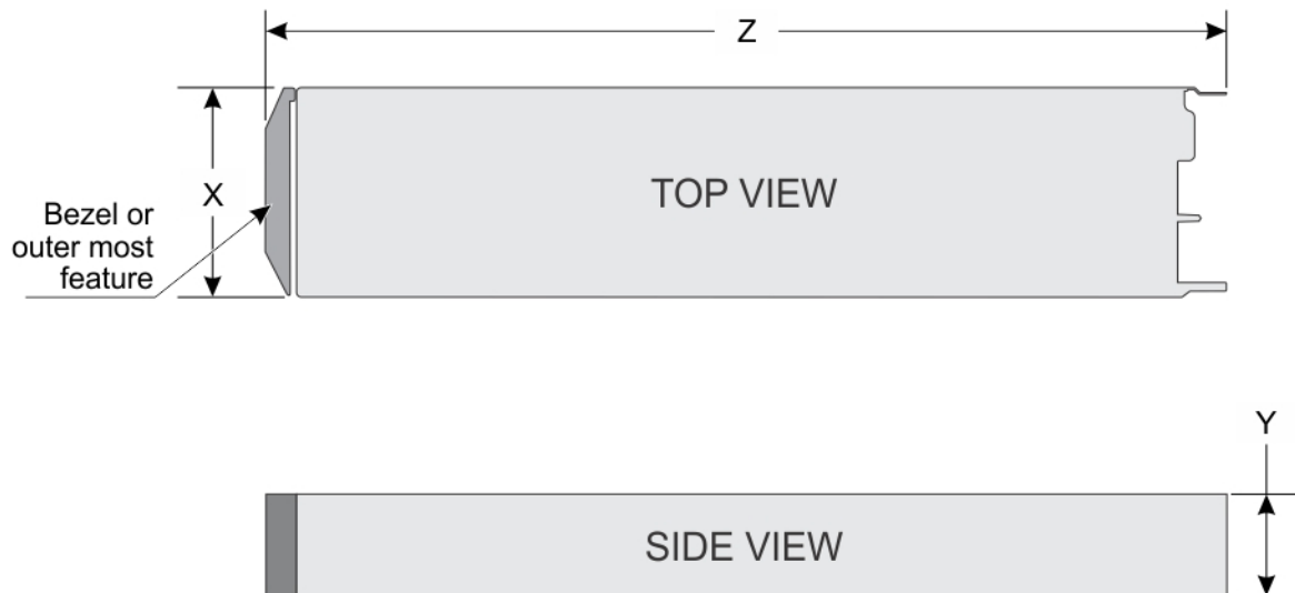
Figure 6. Dimensions du système
