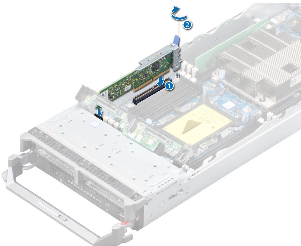
Figure 49. Installation du module IDSDM facultatif
