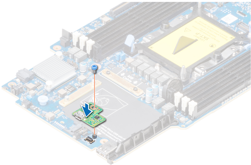
Figure 55. Installation de la carte rSPI
