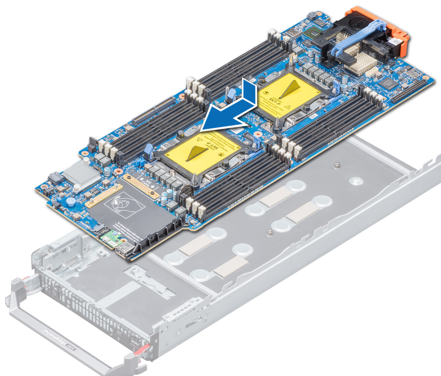
Figure 52. Installation de la carte système
