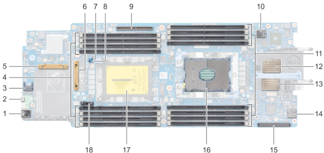
Figure 56. Connecteurs de carte système
