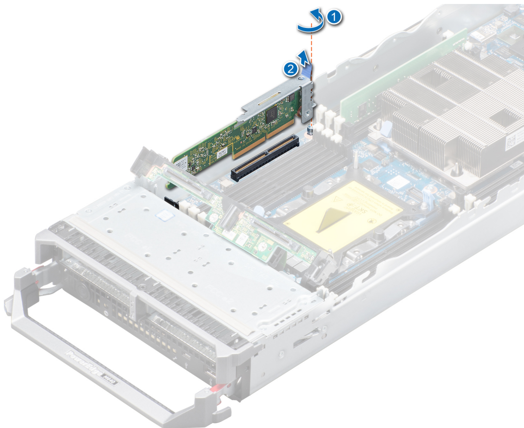
Figure 48. Retrait du module IDSDM optionnel
