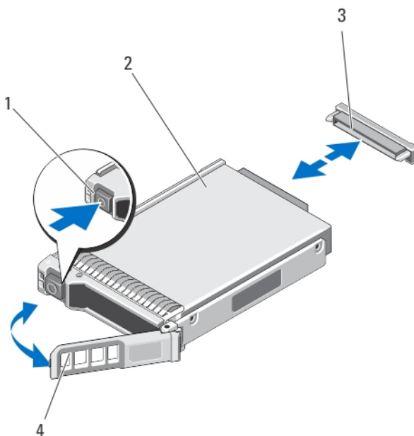
Figure 7. Retrait et installation d'un disque dur/SSD PCIe
