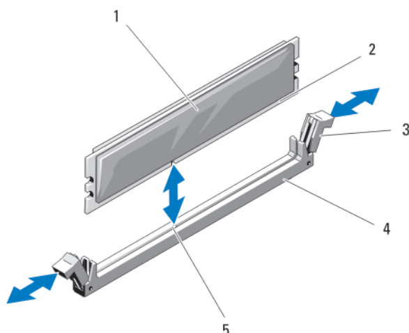
Figure 22. Installation et retrait d'une barrette de mémoire ou d'un cache
