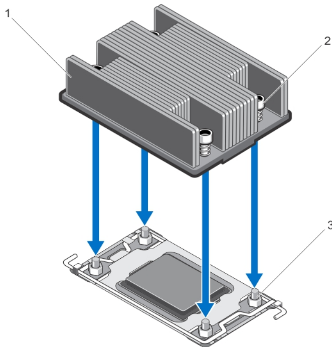
Figure 17. Retrait et installation du dissipateur de chaleur
