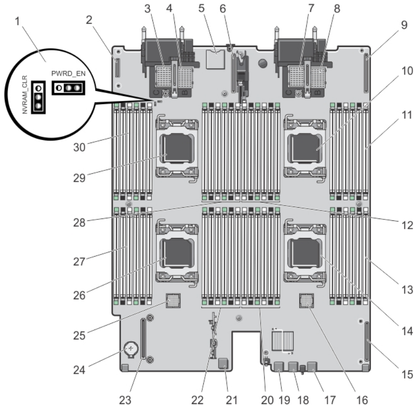
Figure 26. Connecteurs de la carte système
