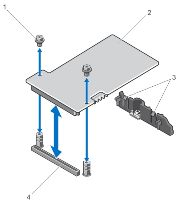
Figure 24. Retrait et installation de la carte contrôleur de stockage
