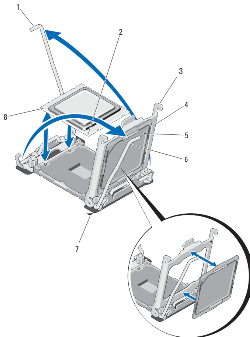
Figure 19. Retrait et installation d'un processeur
