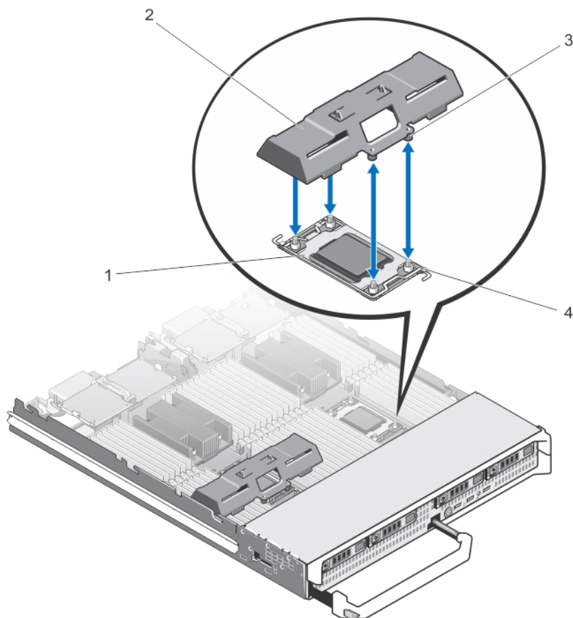
Figure 16. Retrait et installation d'un cache de processeur/de barrette de mémoire DIMM
