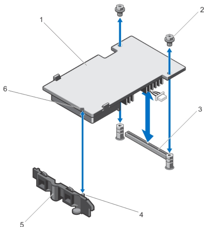
Figure 25. Retrait et installation d'une PCIe extender
