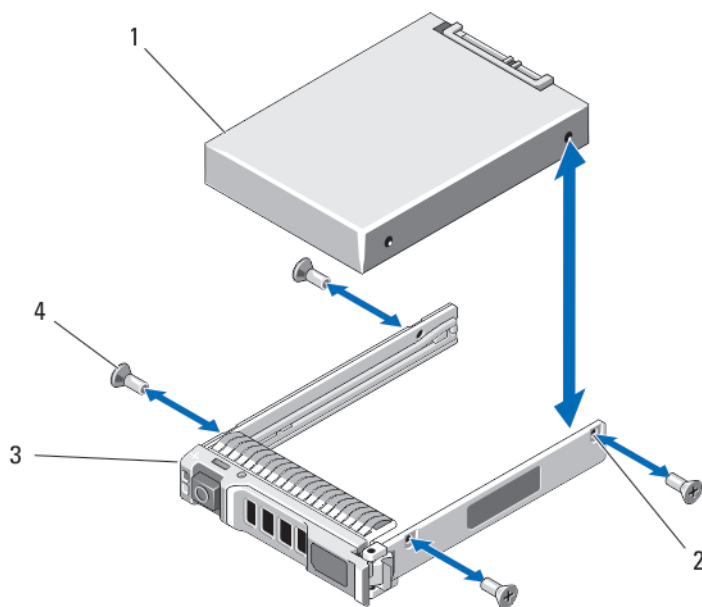
Figure 8. Retrait et installation d'un disque dur/SSD PCIe dans un support de disque dur
