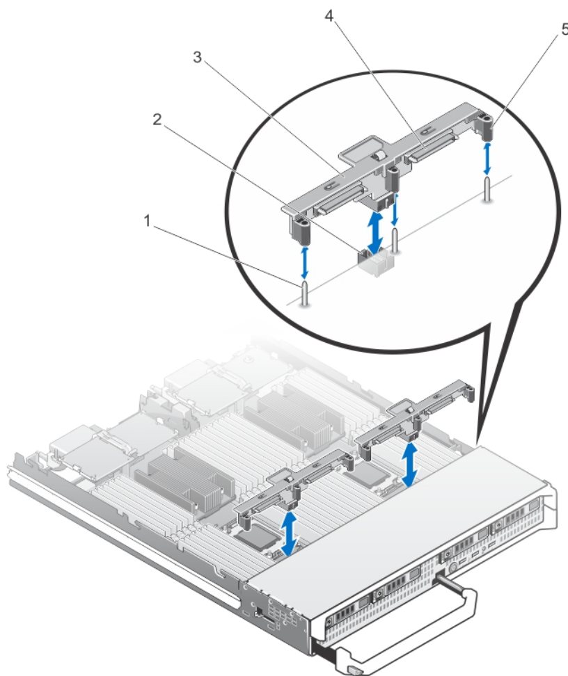
Figure 10. Retrait et installation du fond de panier de disque dur/SSD (mi-longueur)
