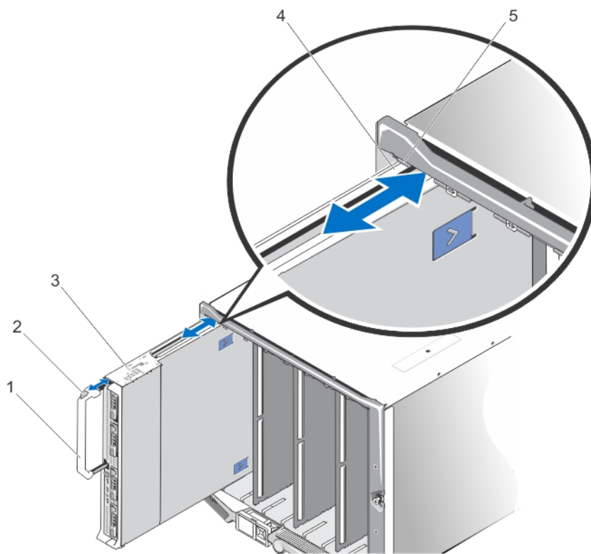
Figure 3. Retrait et installation du serveur lame
