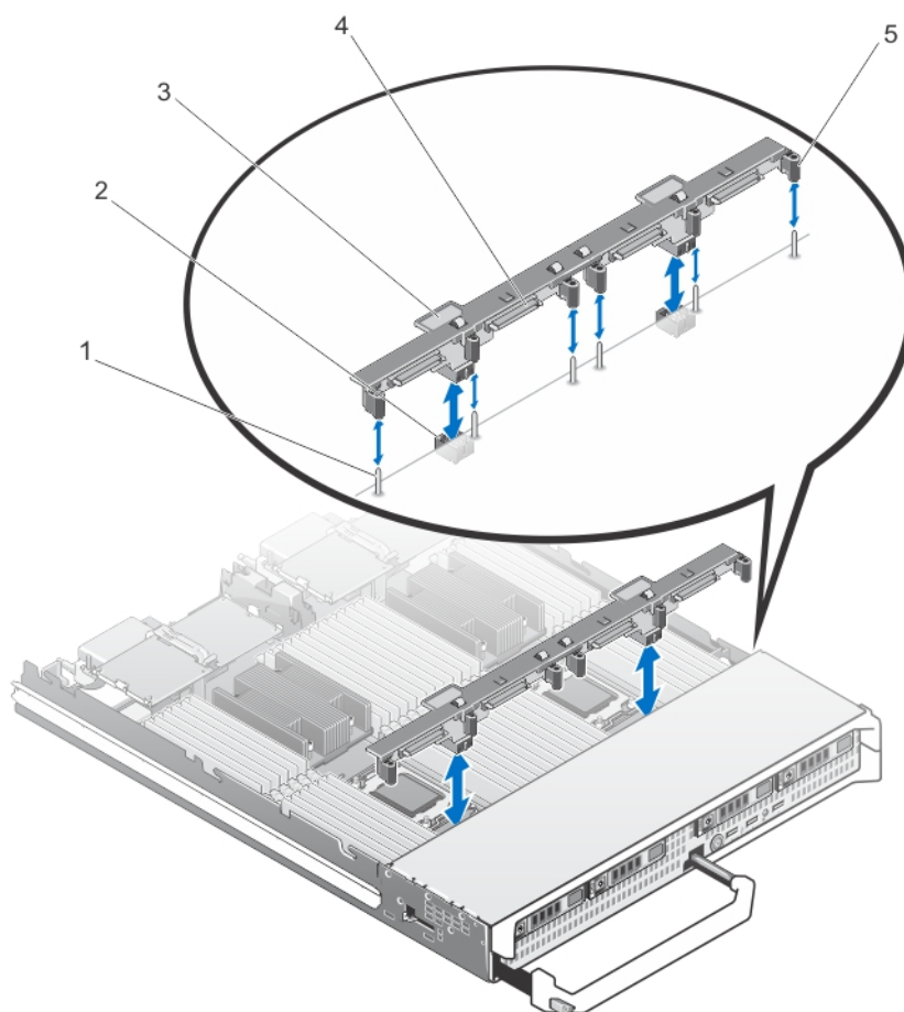
Figure 9. Retrait et installation du fond de panier de disque dur/SSD (pleine longueur)
