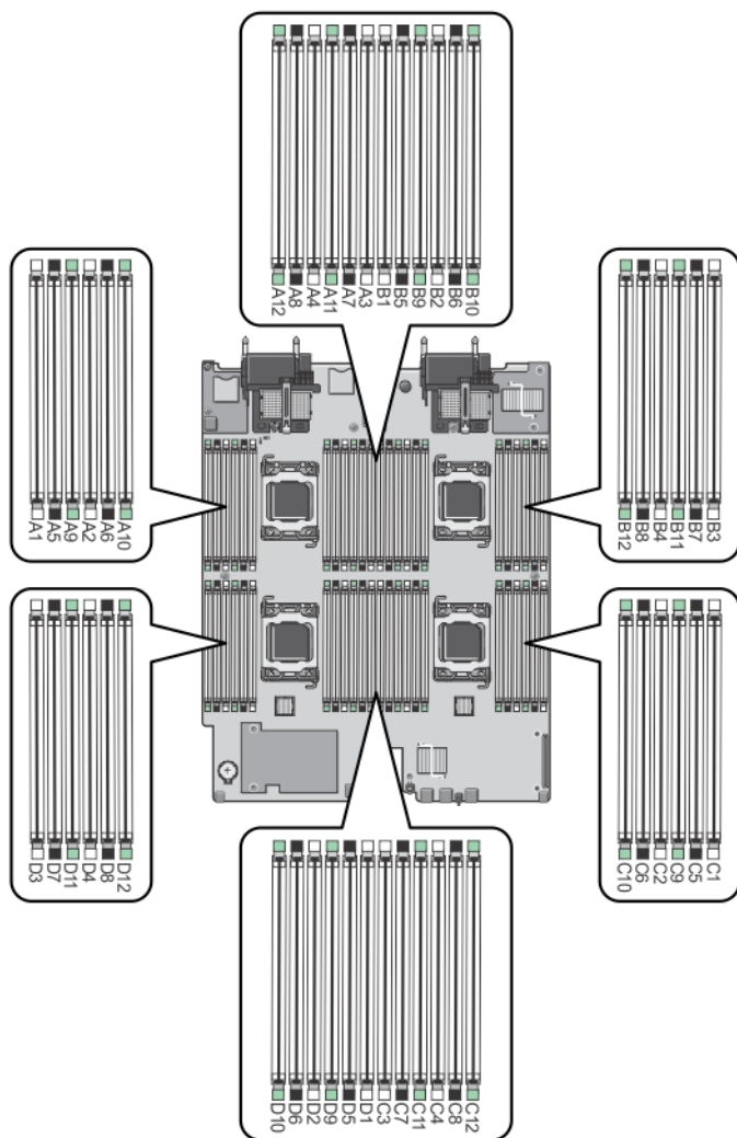
Figure 21. Emplacement des supports de mémoire
