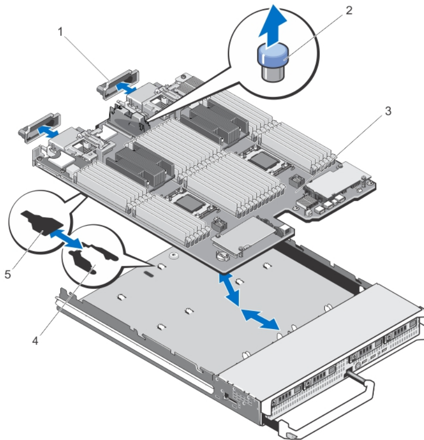
Figure 20. Retrait et installation de la carte système
