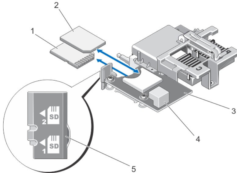
Figure 13. Remplacement de la carte SD
