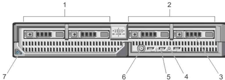
Figure 1. Voyants et fonctions du panneau avant
