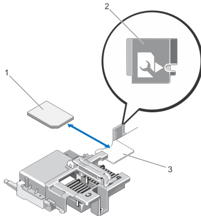
Figure 15. Remplacement de la carte SD vFlash
