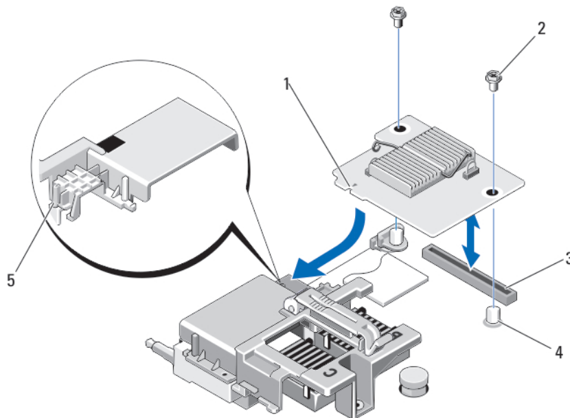
Figure 12. Retrait ou installation de la carte réseau fille/carte de montage LOM
