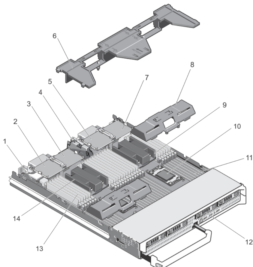
Figure 5. À l'intérieur du serveur lame
