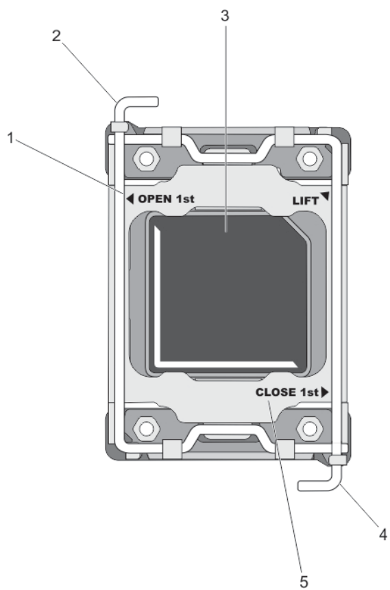
Figure 18. Séquence d'ouverture et de fermeture du levier du cadre de protection du processeur
