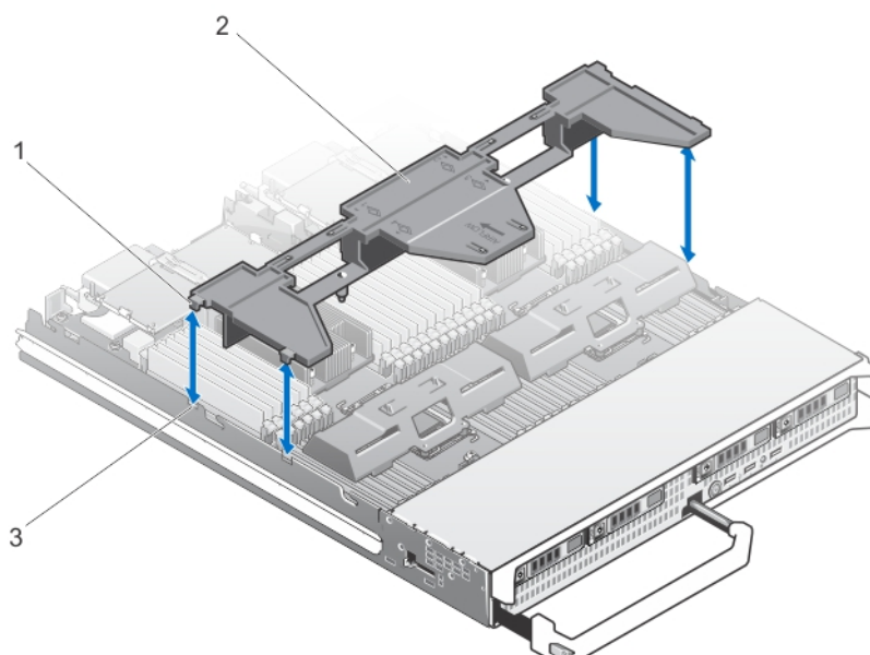
Figure 6. Retrait et installation d'un carénage de refroidissement
