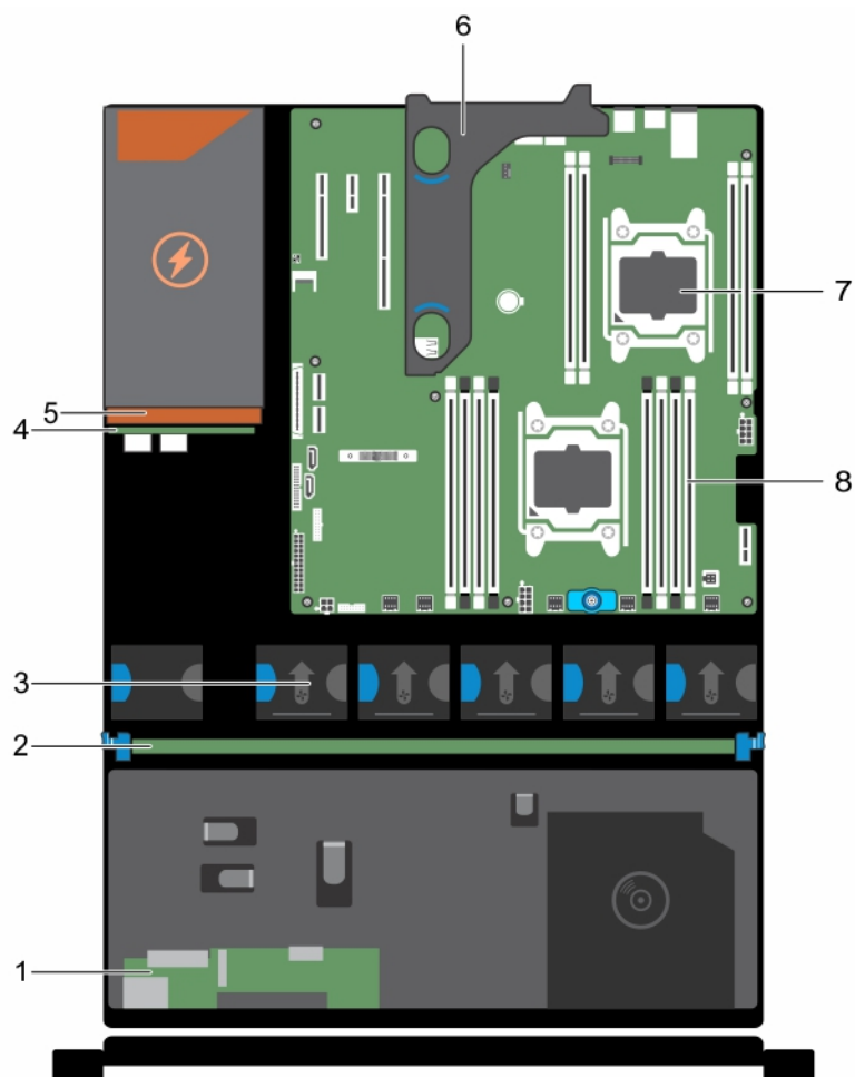
Figure 16. À l'intérieur du système - Châssis du bloc d'alimentation redondant
