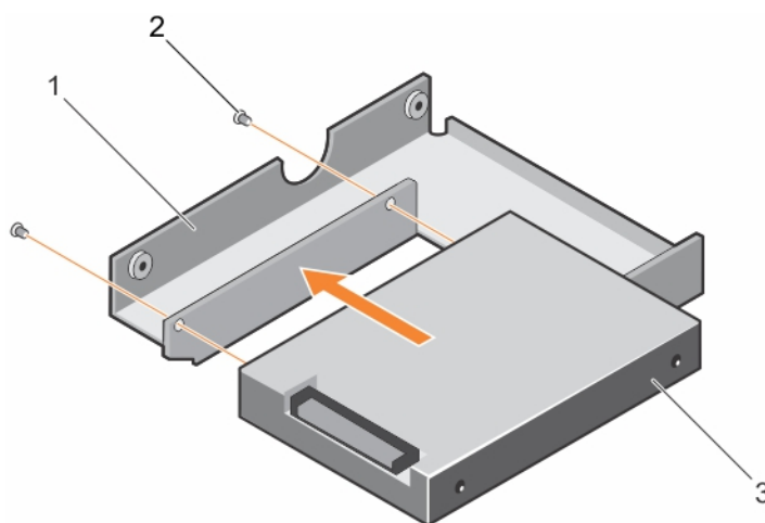
Figure 28. Installation d'un disque dur de 2,5 pouces remplaçable à chaud dans un adaptateur de disque dur de 3,5 pouces
