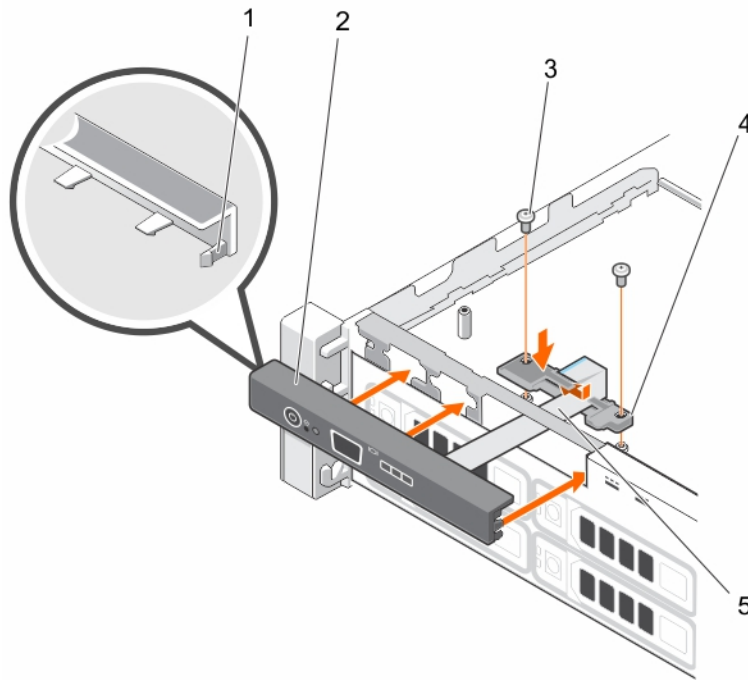
Figure 84. Installation du panneau de commande
