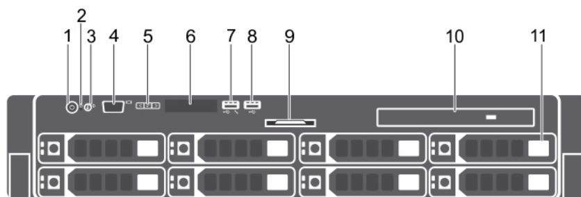
Figure 2. Disques durs de 3,5 ou 2,5 pouces échangeables à chaud (dans un support de disque hybride)
