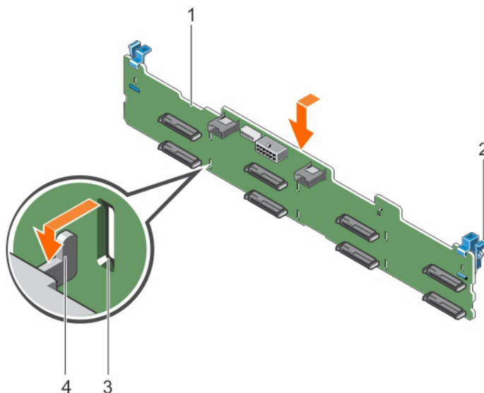
Figure 80. Installation du fond de panier de disque dur
