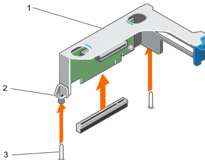
Figure 41. Retrait de la carte de montage pour carte d'extension
