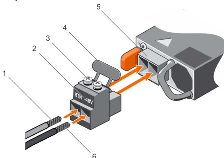
Figure 70. Assemblage des câbles d'alimentation d'entrée en CC
