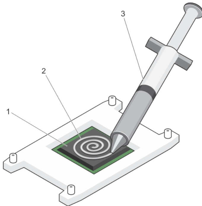
Figure 60. Application de graisse thermique sur la partie supérieure du processeur
