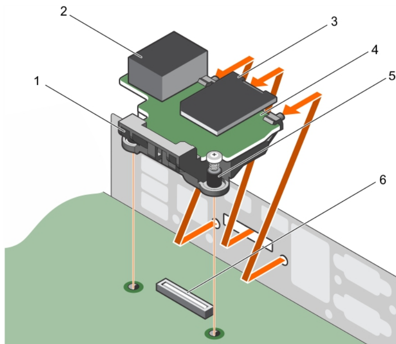
Figure 47. Retrait de la carte des ports iDRAC
