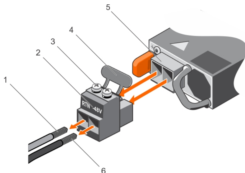
Figure 71. Retrait des câbles d'alimentation d'entrée en CC
