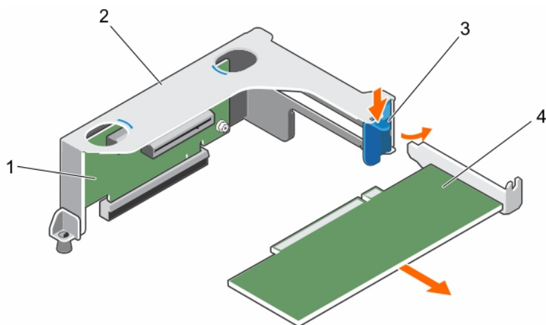
Figure 43. Retrait d'une carte d'extension de la carte de montage pour carte d'extension
