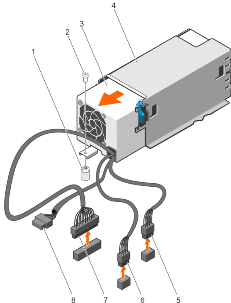
Figure 66. Retrait d'un bloc d'alimentation en CA non redondant (câblé)
