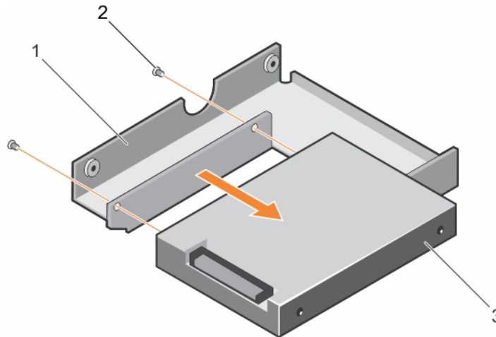
Figure 27. Retrait d'un disque dur de 2,5 pouces remplaçable à chaud dans un adaptateur de disque dur de 3,5 pouces
