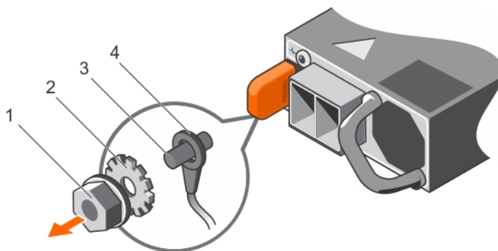
Figure 69. Retrait du câble de terre de sécurité
