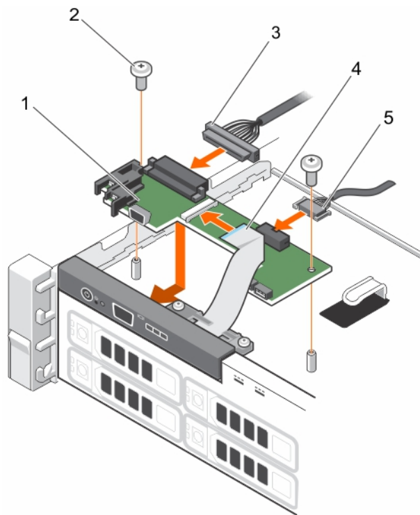
Figure 82. Installation de la carte du panneau de commande
