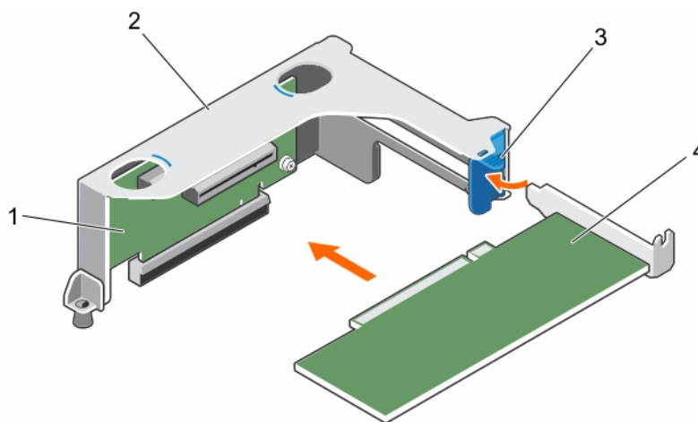
Figure 45. Installation d'une carte d'extension dans la carte de montage pour carte d'extension
