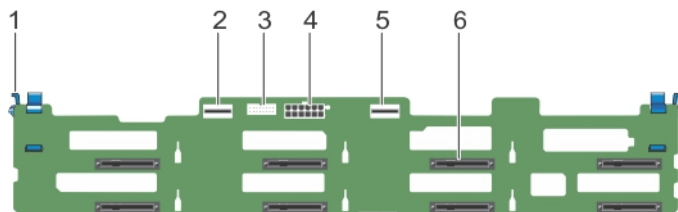
Figure 77. Retrait du fond de panier de disque dur
