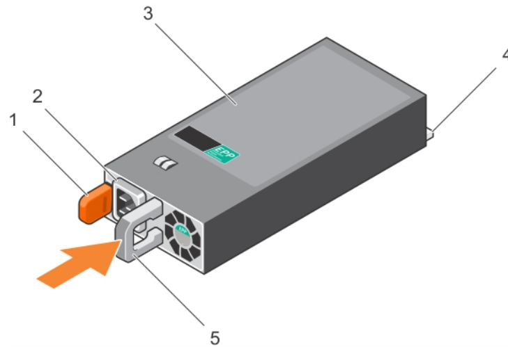
Figure 65. Installation d'un bloc d'alimentation (PSU) CA
