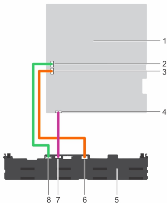
Figure 78. Schéma de câblage du fond de panier de disque dur à l'aide du contrôleur intégré
