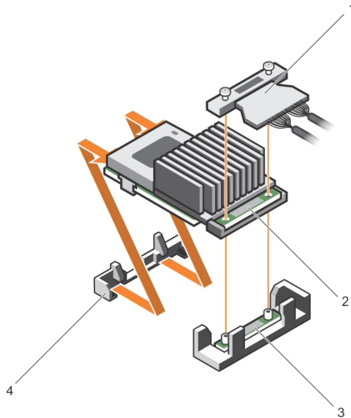
Figure 54. Retrait de la carte contrôleur de stockage intégrée
