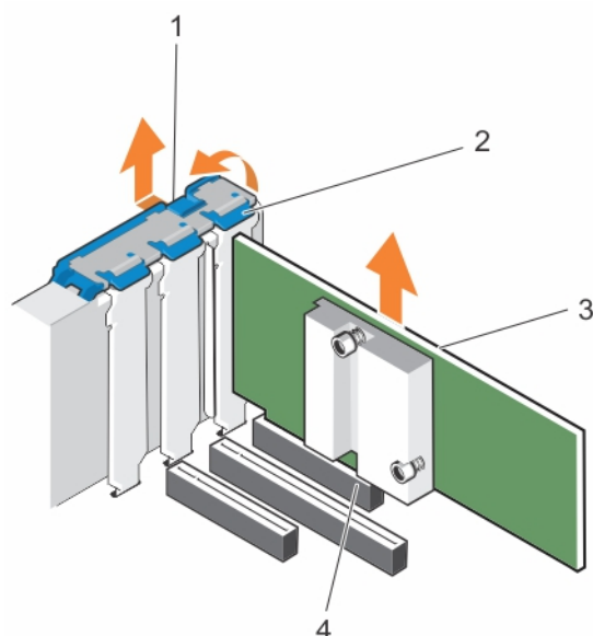
Figure 39. Retrait d'une carte d'extension de la carte système
