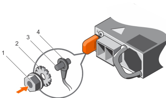
Figure 68. Assemblage et connexion du câble de mise à la terre
