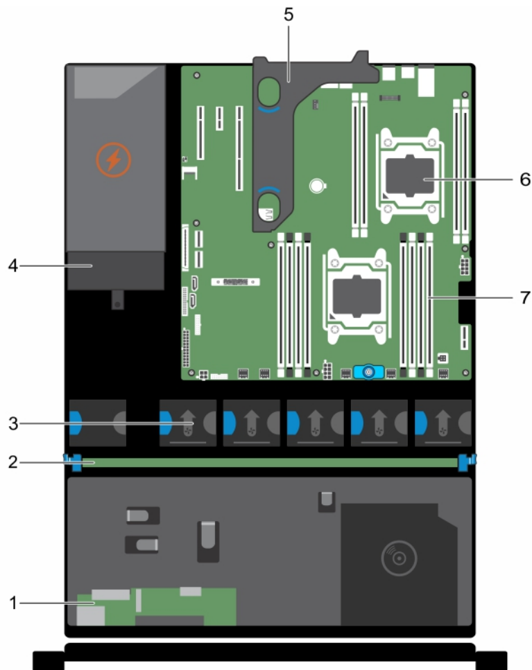
Figure 17. À l'intérieur du système - Châssis du bloc d'alimentation non redondant
