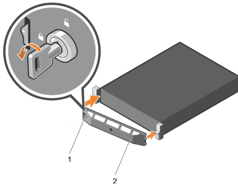
Figure 13. Installation du cadre avant optionnel
