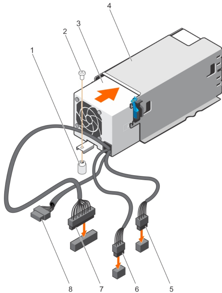
Figure 67. Installation d'un bloc d'alimentation en CA non redondant
