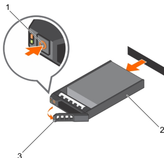
Figure 23. Retrait d'un disque dur ou SSD remplaçable à chaud
