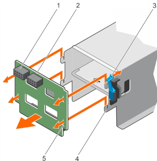
Figure 74. Retrait de la carte intercalaire d'alimentation
