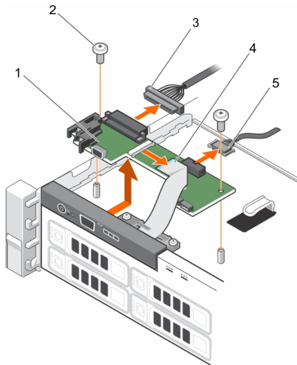
Figure 81. Retrait de la carte du panneau de commande
