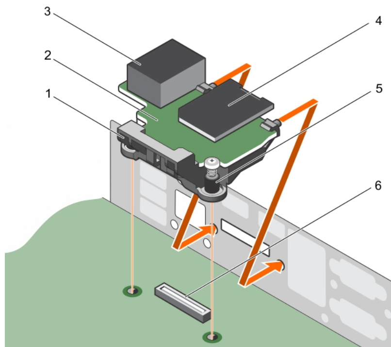
Figure 48. Installation de la carte des ports iDRAC
