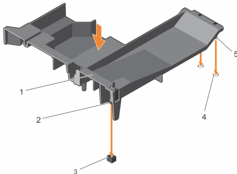
Figure 19. Installation du carénage de refroidissement
