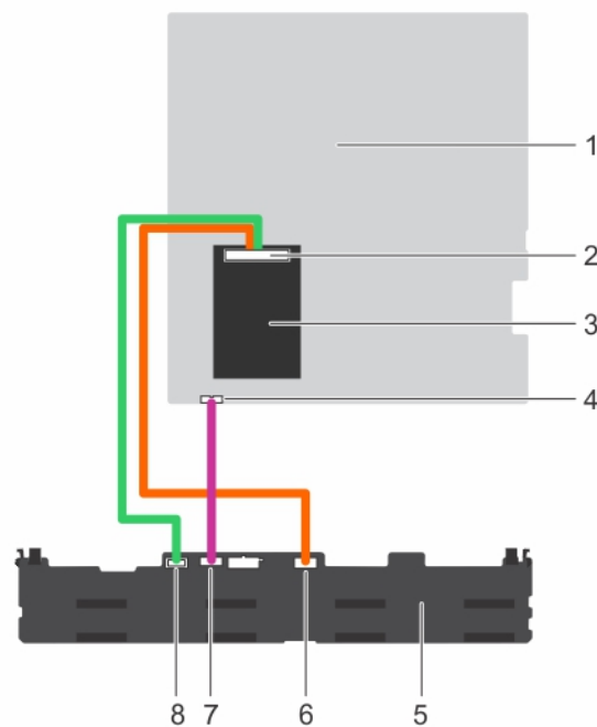
Figure 79. Schéma de câblage du fond de panier de disque dur à l'aide du contrôleur de stockage intégré
