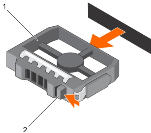
Figure 25. Retrait d'un cache de disque dur 3,5 pouces
