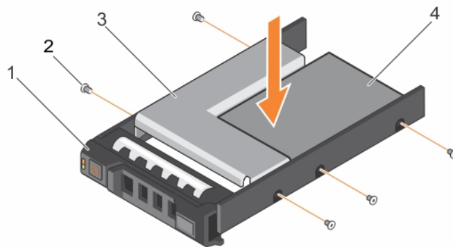
Figure 30. Installation d'un adaptateur de disque dur de 3,5 pouces dans un support de disques durs remplaçable à chaud
