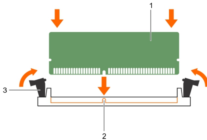
Figure 22. Installation de la barrette de mémoire
