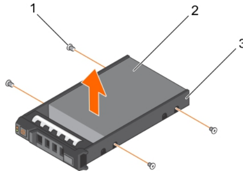
Figure 31. Retrait d'un disque dur d'un support de disque dur
