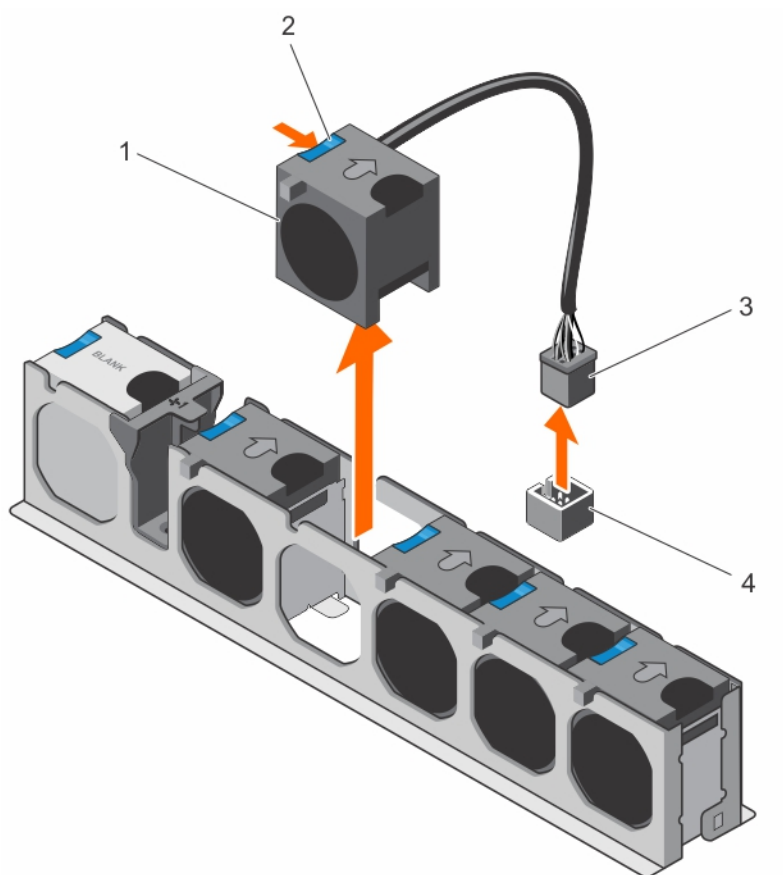
Figure 35. Retrait d'un ventilateur de refroidissement
