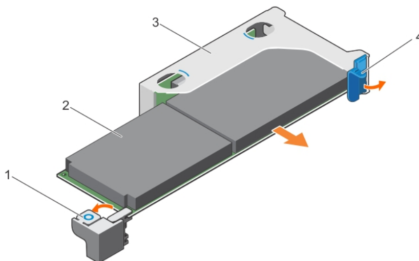
Figure 44. Retrait d'une carte de montage pleine hauteur, pleine longueur, d'une carte de montage pour carte d'extension
