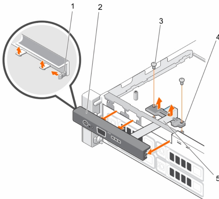
Figure 83. Retrait du panneau de commande
