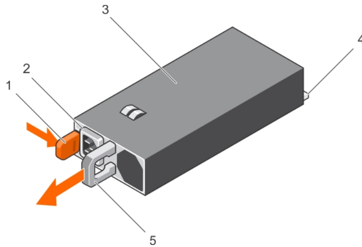
Figure 64. Retrait d'un bloc d'alimentation (PSU) CA
