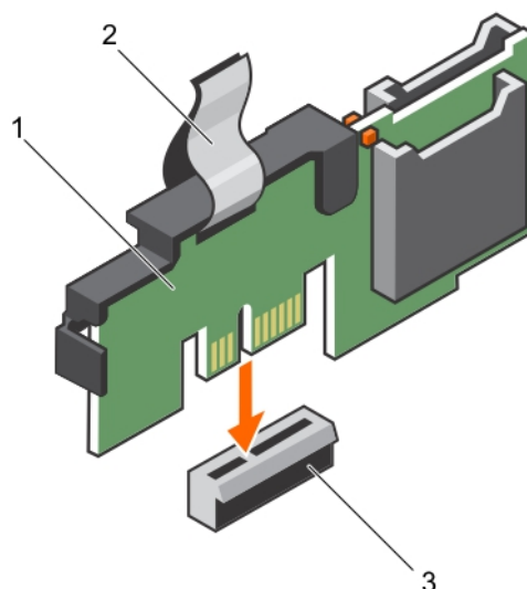
Figure 53. Installation du module SD interne double en option
