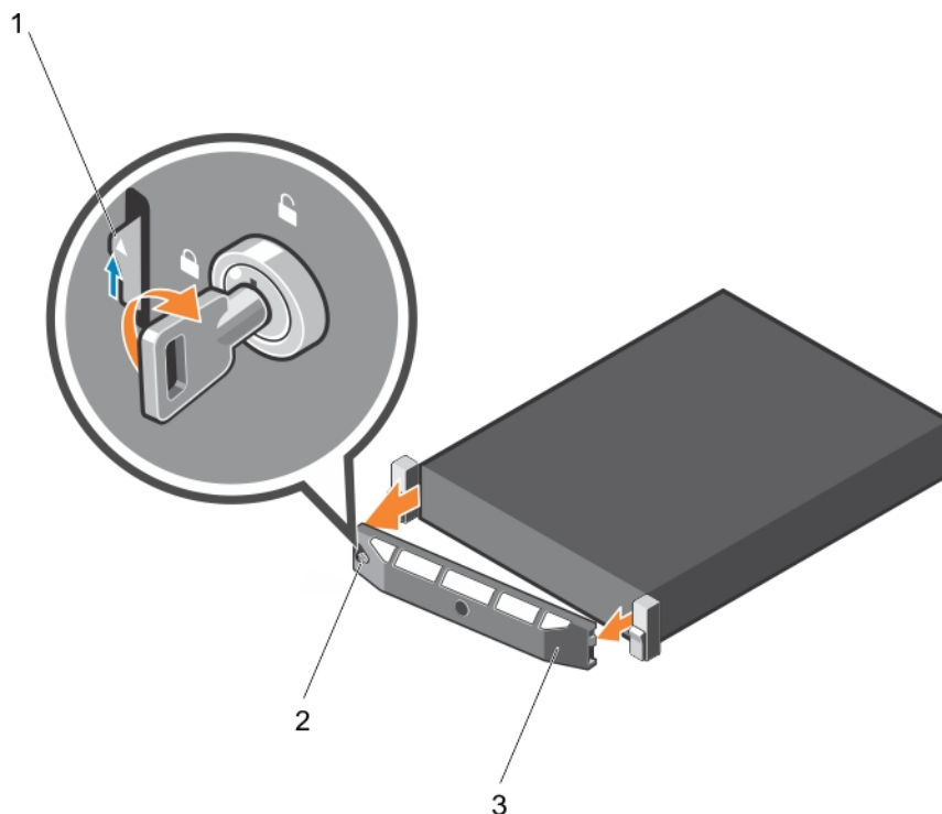
Figure 12. Retrait du cadre avant en option.
