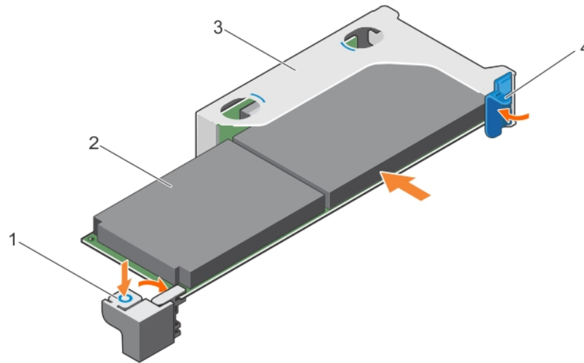
Figure 46. Installation d'une carte de montage pleine hauteur, pleine longueur, dans une carte de montage pour carte d'extension
