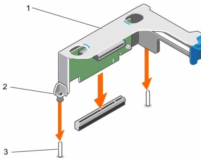
Figure 42. Installation de la carte de montage pour carte d'extension
