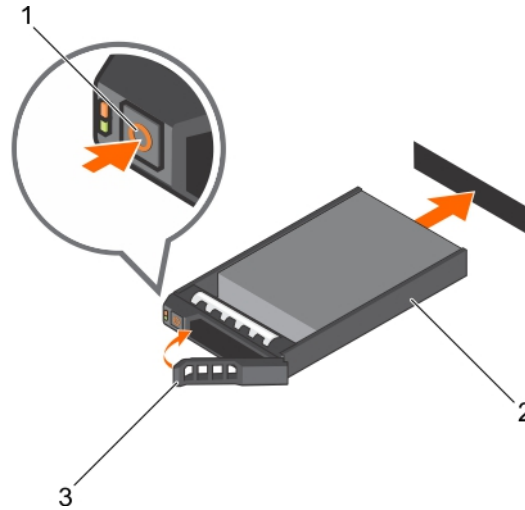
Figure 24. Installation d'un disque dur ou SSD remplaçable à chaud
