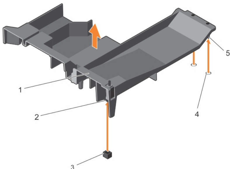
Figure 18. Retrait du carénage de refroidissement
