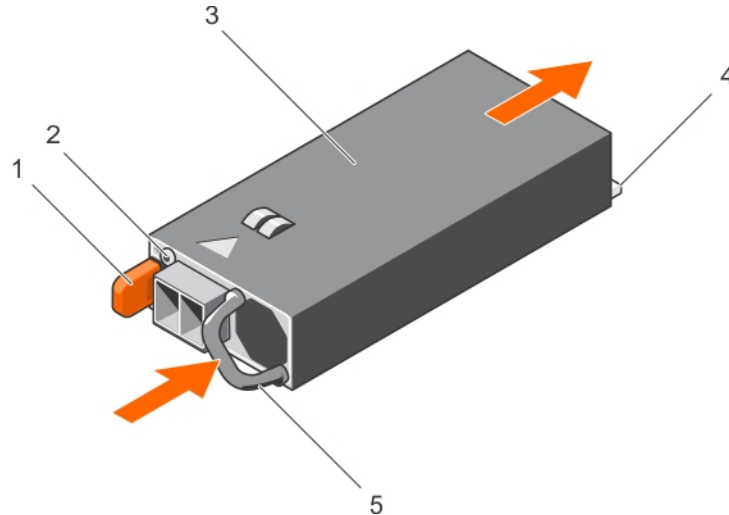
Figure 73. Installation d'un bloc d'alimentation en CC
