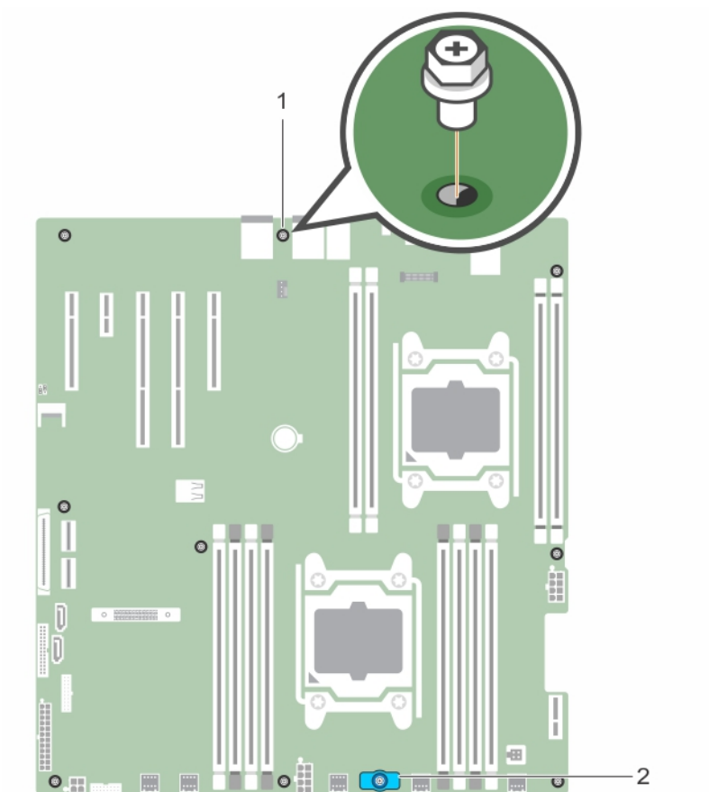
Figure 85. Emplacement de vis sur la carte système
