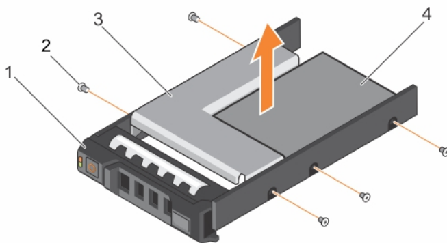
Figure 29. Retrait d'un adaptateur de disque dur remplaçable à chaud de 3,5 pouces d'un support de disque dur remplaçable à chaud de 3,5 pouces
