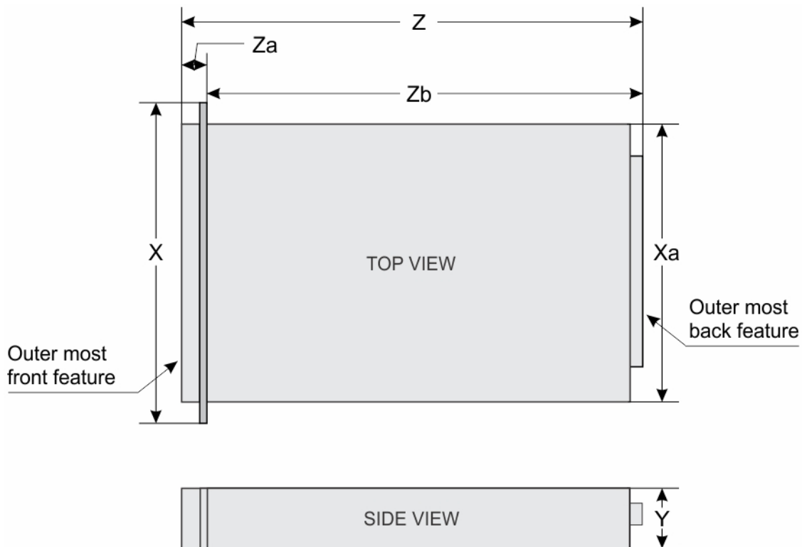
Figure 11. Dimensions du châssis du système PowerEdge R530
