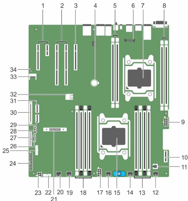
Figure 89. Connecteurs et cavaliers de la carte système.
