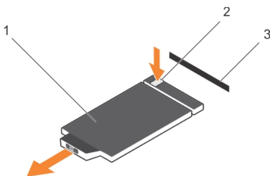
Figure 89. Retrait de la plaquette d'informations
