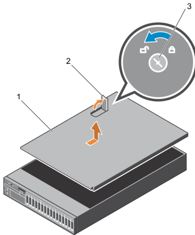
Figure 12. Retrait du capot du système
