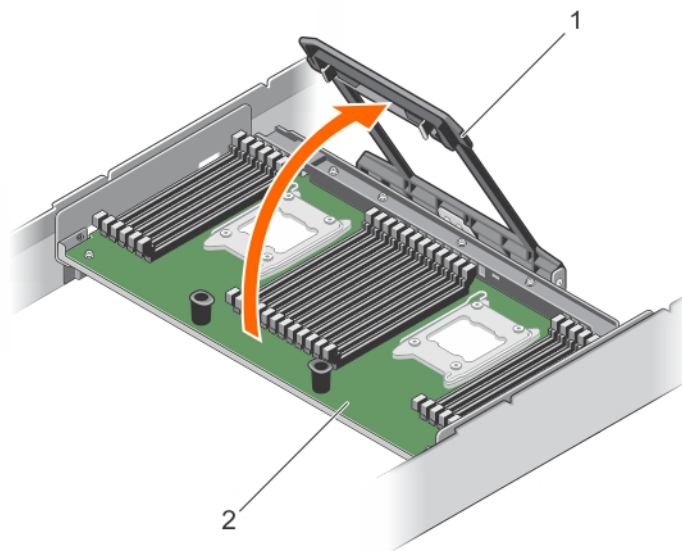
Figure 16. Dégagement du module PEM
