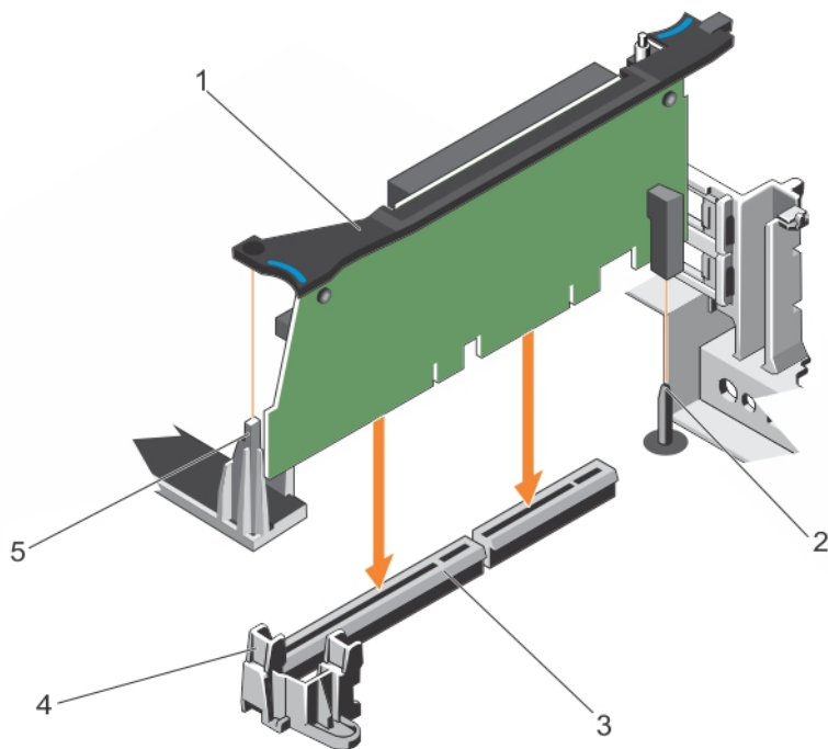
Figure 52. Installation de la carte de montage pour carte d'extension 3
