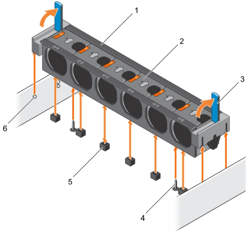
Figure 26. Retrait de l'assemblage de ventilation
