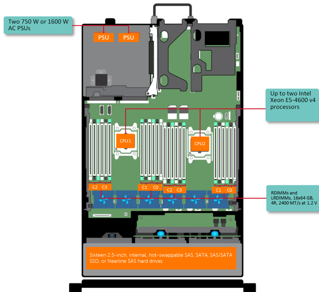
Figure 1. Configurations prises en charge pour un système PowerEdge R830 à deux processeurs
