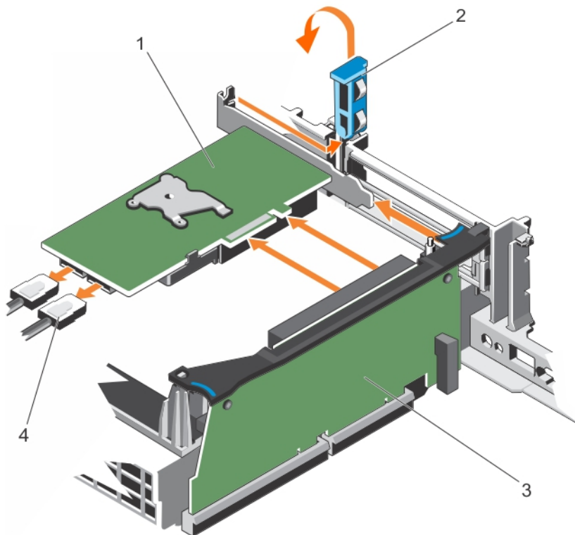
Figure 42. Retrait de la carte contrôleur de stockage intégrée
