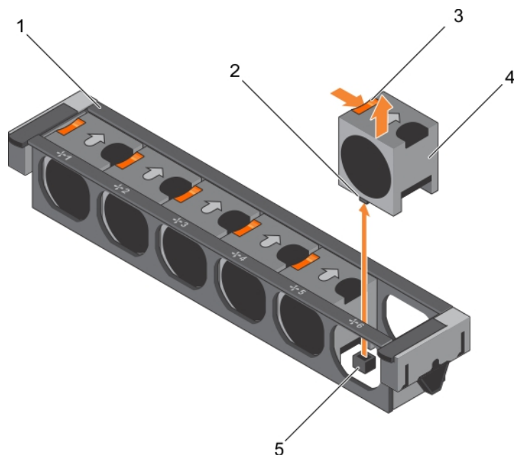
Figure 24. Retrait d'un ventilateur de refroidissement
