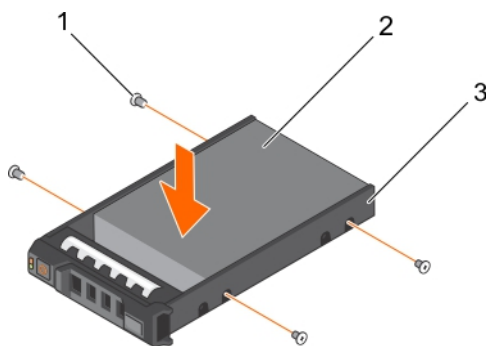
Figure 76. Installation d'un disque dur dans un support de disque dur
