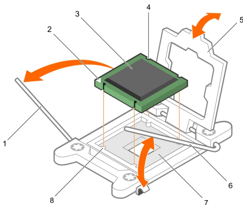
Figure 35. Installation d'un processeur
