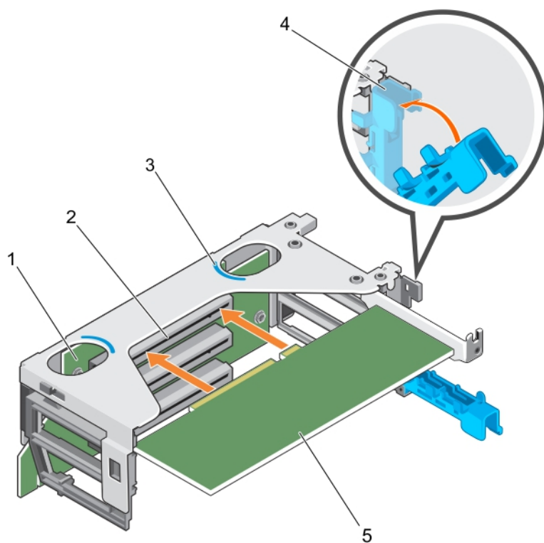
Figure 56. Installation d'une carte d'extension dans la carte de montage 2 pour carte d'extension
