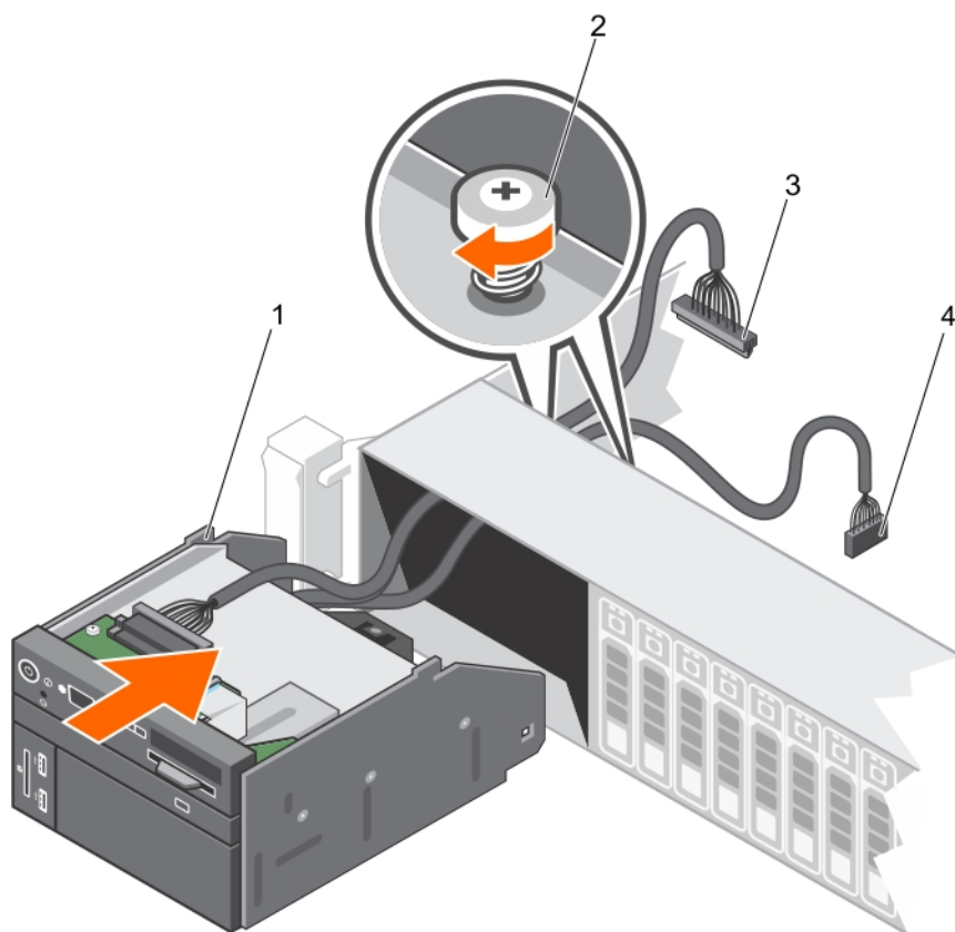
Figure 91. Installation du panneau de commande
