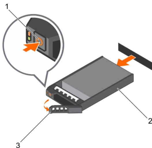
Figure 71. Retrait d'un disque dur ou SSD remplaçable à chaud
