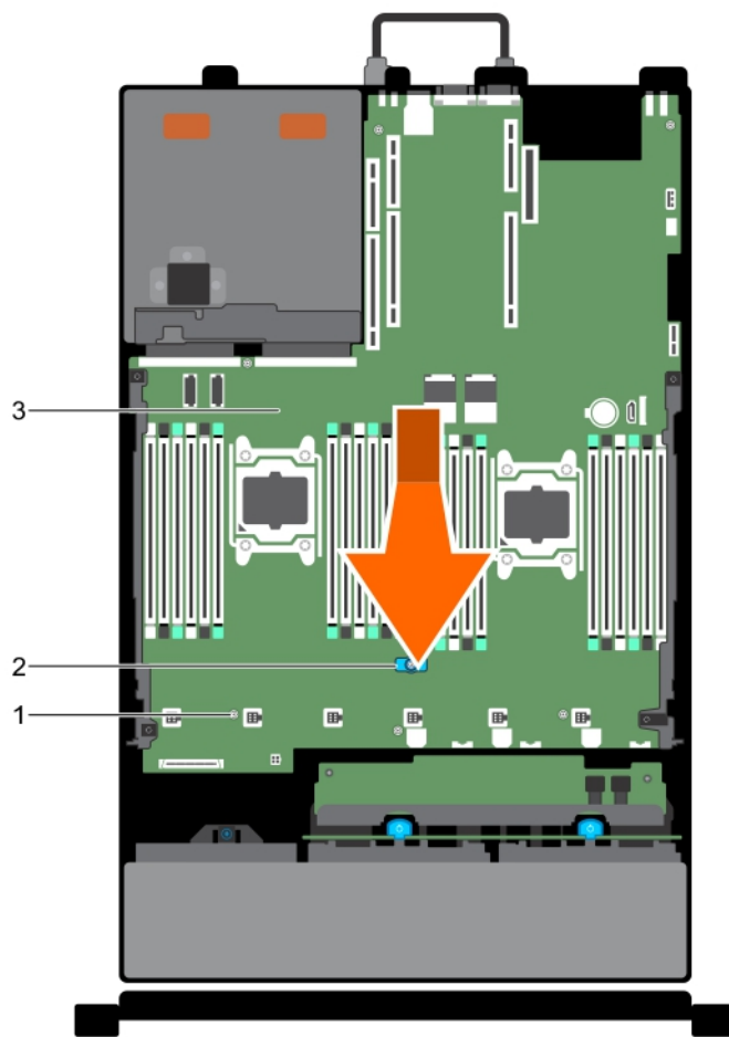
Figure 93. Retrait de la carte système
