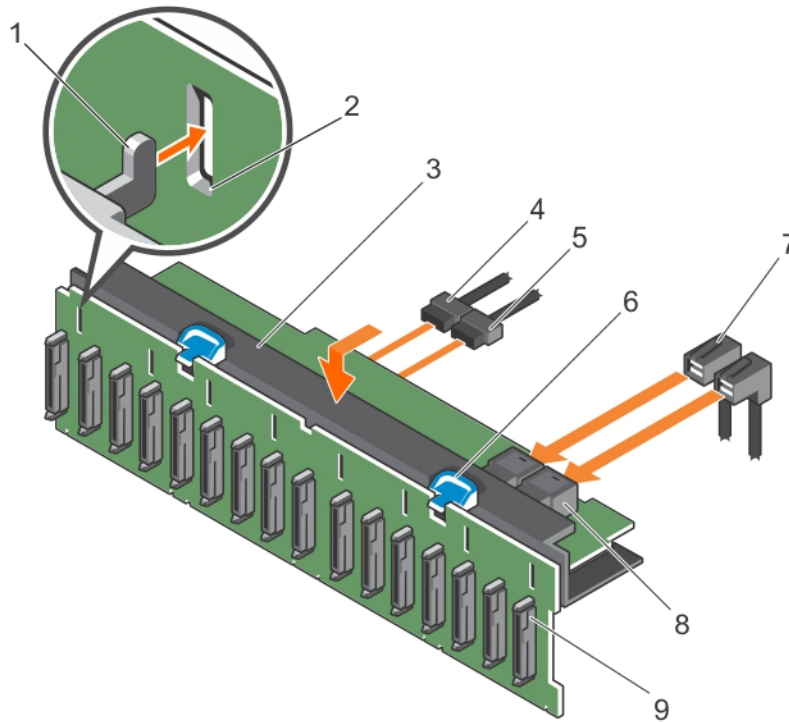
Figure 85. Installation du fond de panier SAS/SATA (x16) de 2,5 pouces
