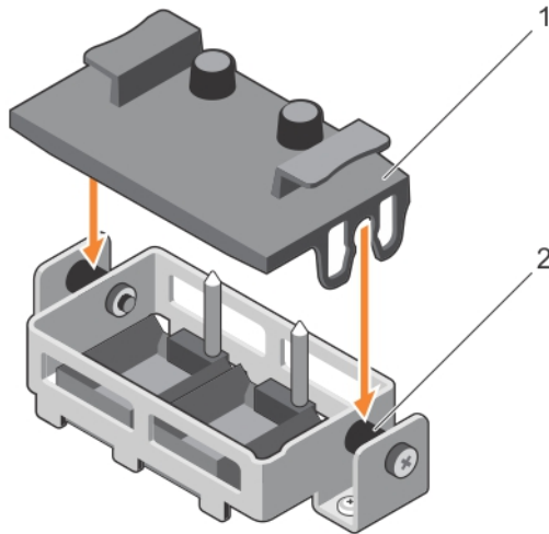
Figure 18. Installation de la plaque de recouvrement sur le connecteur QPI
