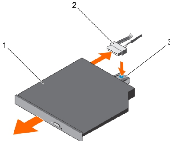
Figure 77. Retrait du lecteur optique en option
