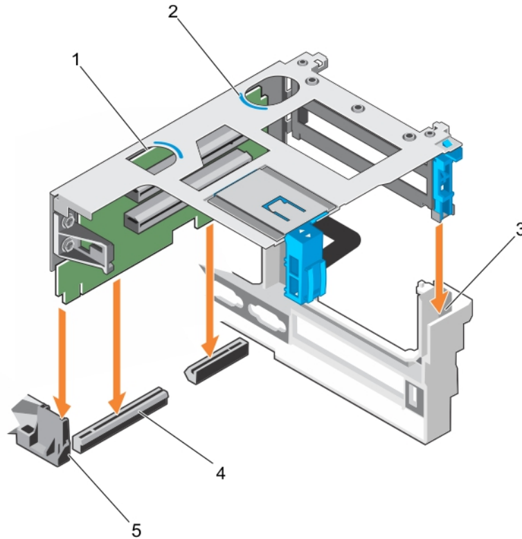
Figure 50. Installation de la carte de montage pour carte d'extension 1
