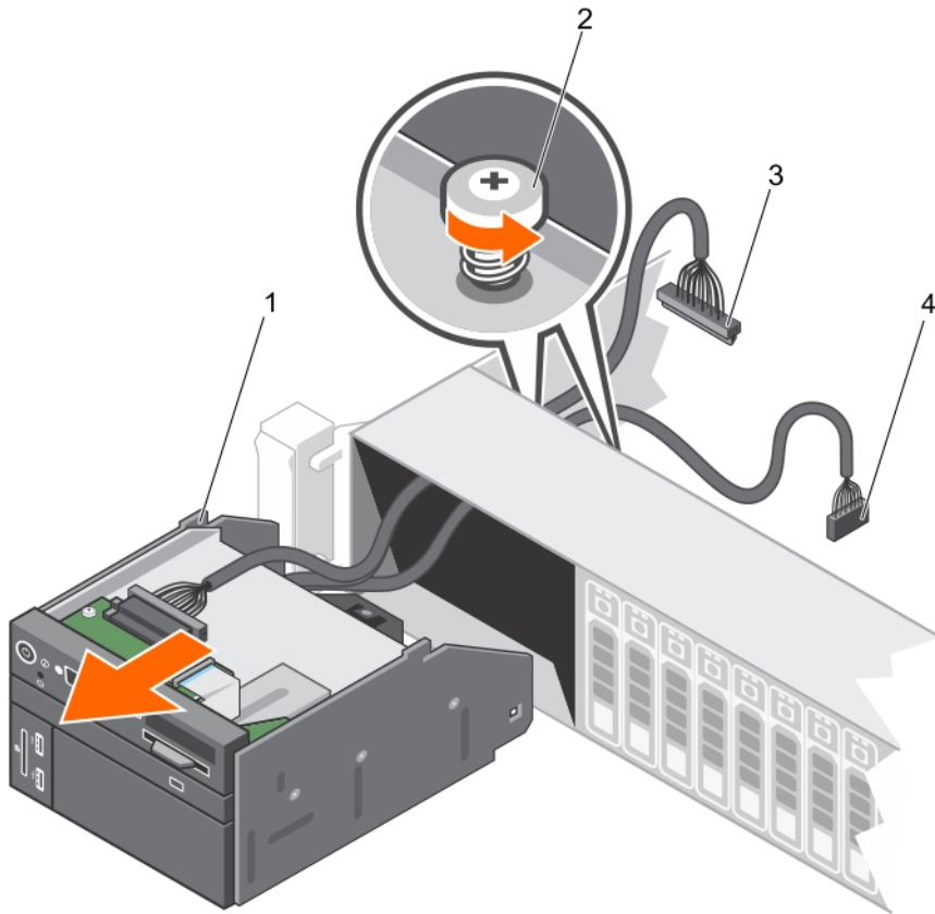
Figure 87. Retrait du panneau de commande
