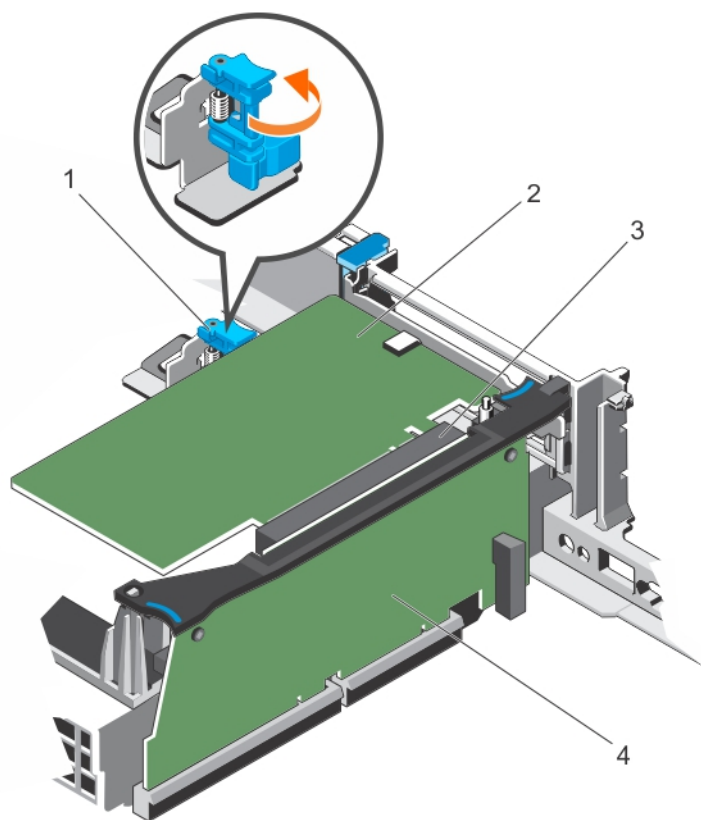
Figure 58. Retrait d'une carte d'extension pleine hauteur de la carte de montage pour carte d'extension 3
