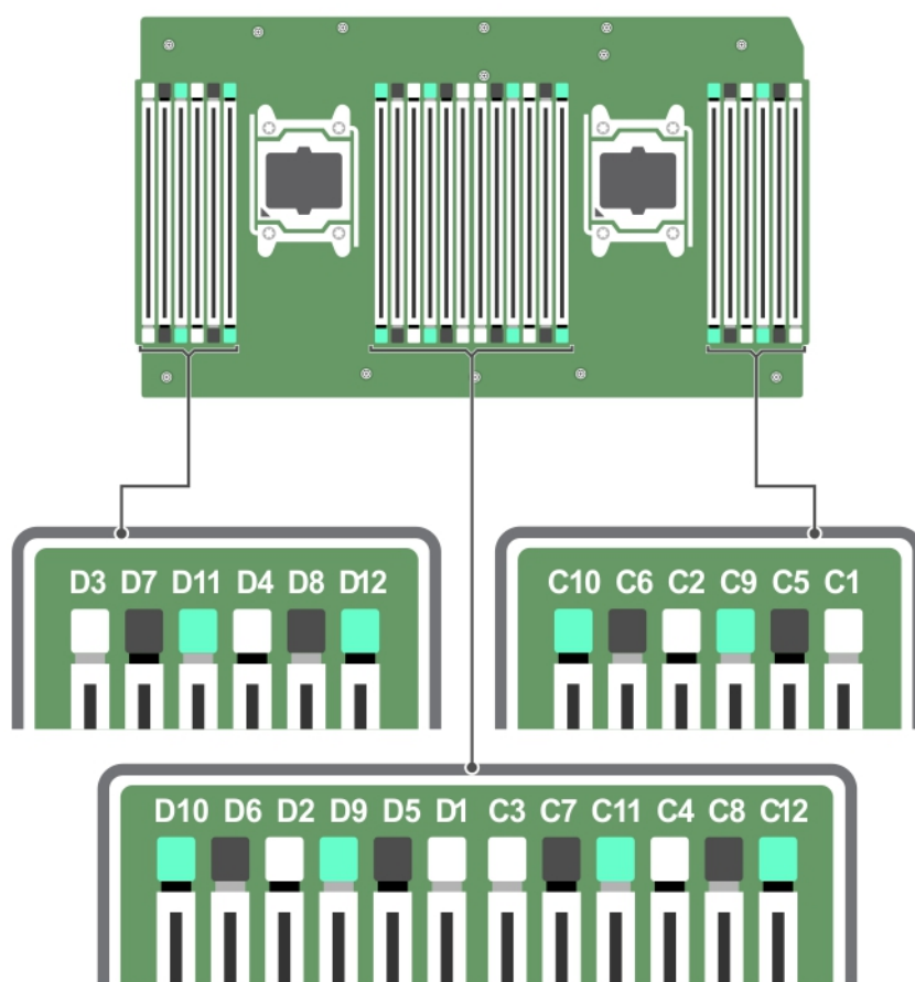
Figure 29. Emplacements de supports de mémoire sur le module d'extension de processeur
