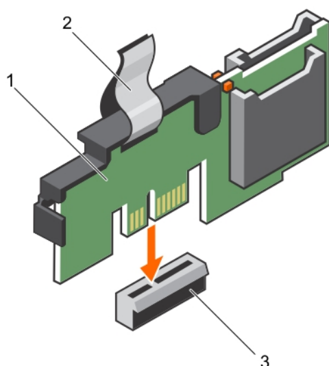
Figure 64. Installation du module SD interne double en option
