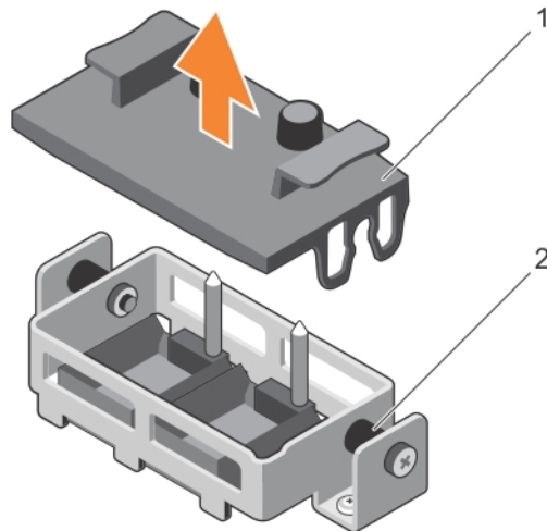
Figure 19. Retrait de la plaque de recouvrement du connecteur QPI
