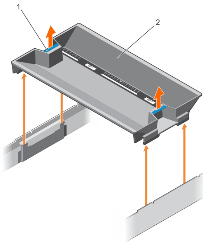
Figure 22. Retrait du carénage de refroidissement
