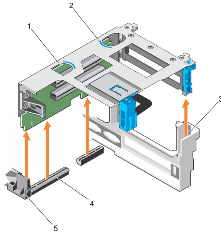
Figure 44. Retrait de la carte de montage pour carte d'extension 1
