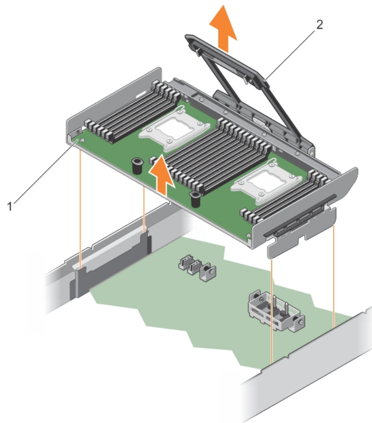
Figure 17. Retrait du module PEM
