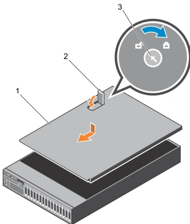
Figure 13. Installation du capot du système
