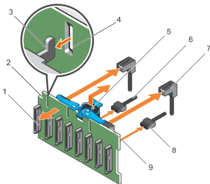
Figure 83. Retrait du fond de panier SAS/SATA de 2,5 pouces (x8)
