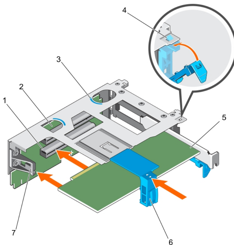
Figure 54. Installation d'une carte d'extension dans la carte de montage 1 pour carte d'extension
