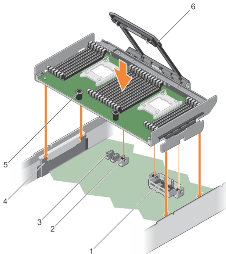
Figure 20. Installation du module PEM
