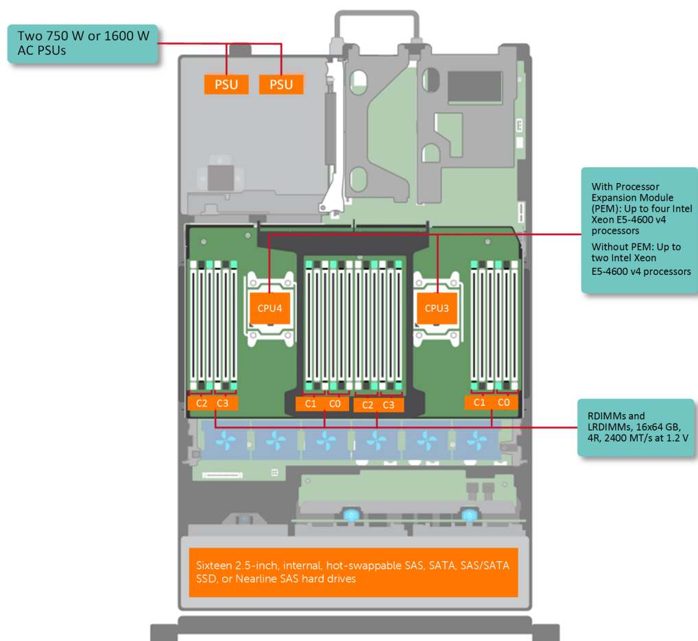
Figure 2. Configurations prises en charge pour un système PowerEdge R830 à quatre processeurs
