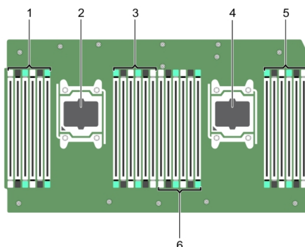
Figure 97. Connecteurs du module d'extension du processeur
