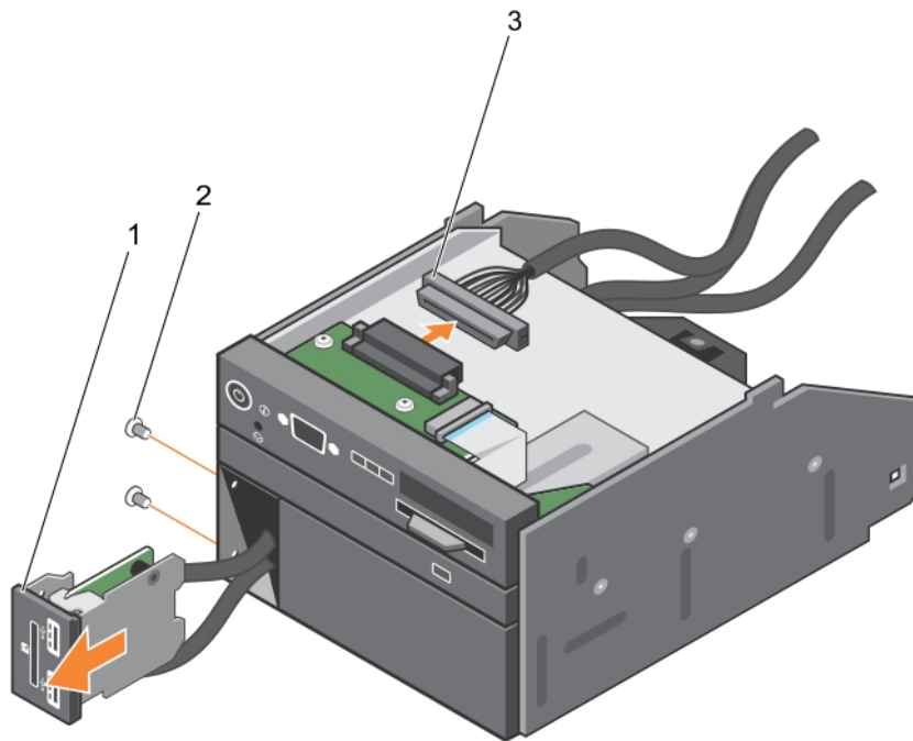
Figure 88. Retrait du connecteur vFlash/module de connecteur USB
