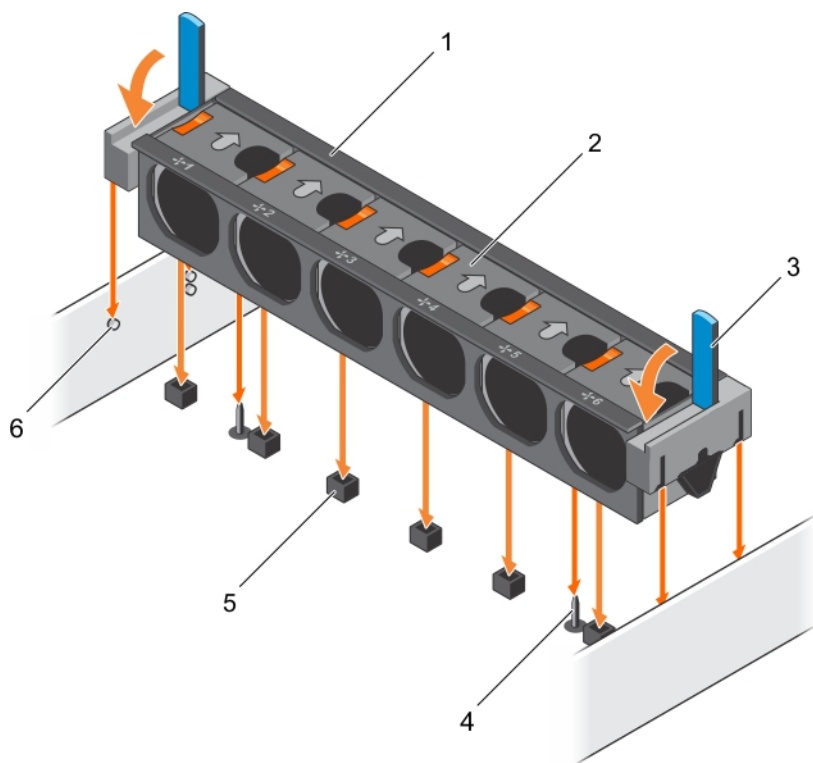
Figure 27. Installation de l'assemblage de ventilation
