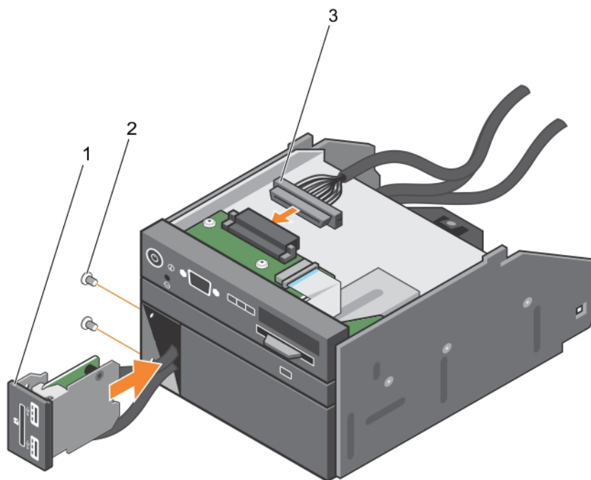
Figure 90. Installation du connecteur vFlash/module de connecteur USB
