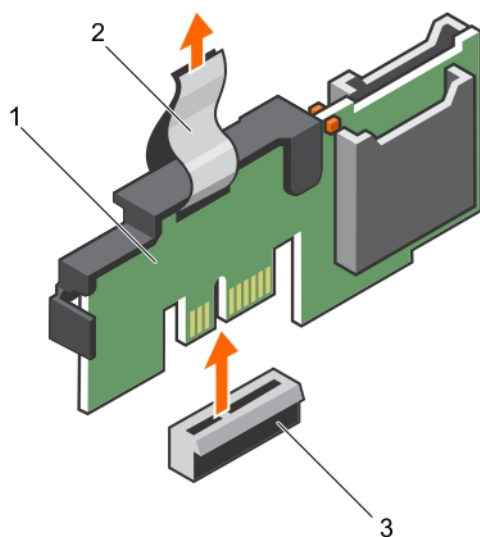
Figure 63. Retrait du module SD interne double (IDSDM)
