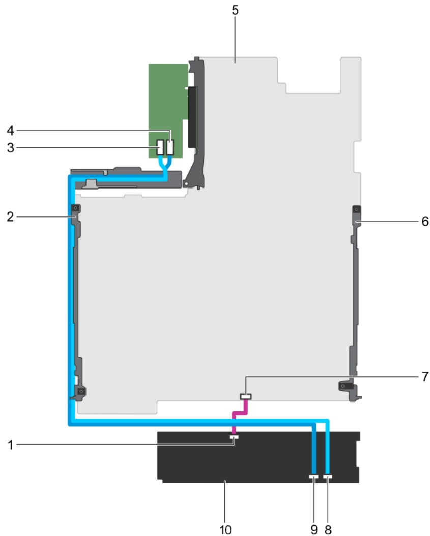
Figure 82. Schéma de câblage : fond de panier SAS/SATA (x16) de 2,5 pouces
