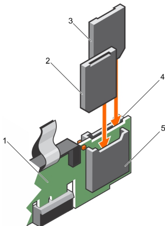
Figure 62. Installation d'une carte SD interne
