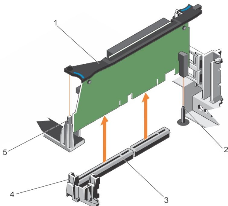
Figure 48. Retrait de la carte de montage pour carte d'extension 3
