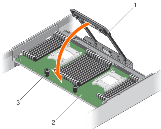
Figure 21. Fixation du module PEM sur le châssis à l'aide du levier de dégagement
