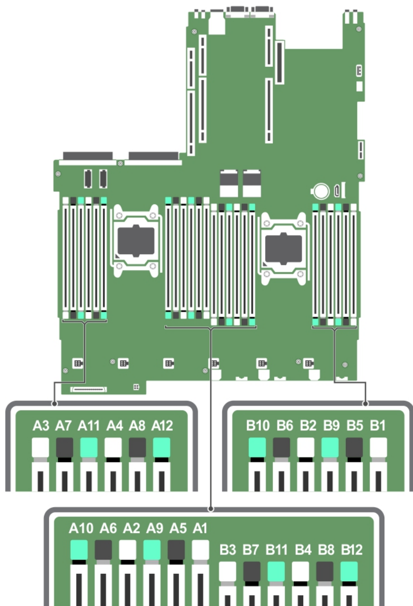
Figure 28. Emplacement des supports de mémoire
