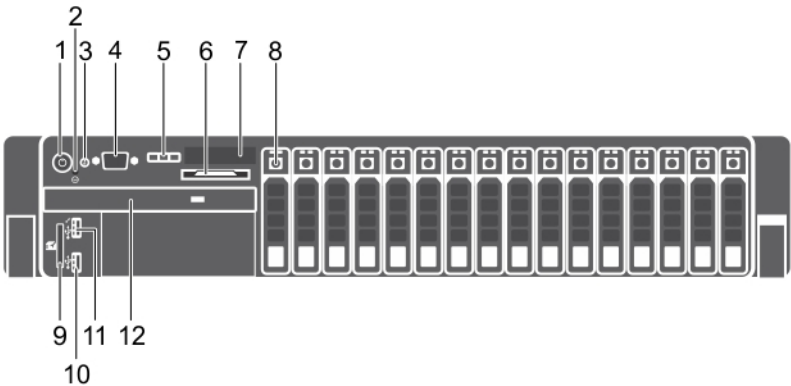
Figure 3. Fonctions du panneau avant (châssis de disque dur de 2,5 pouces)
