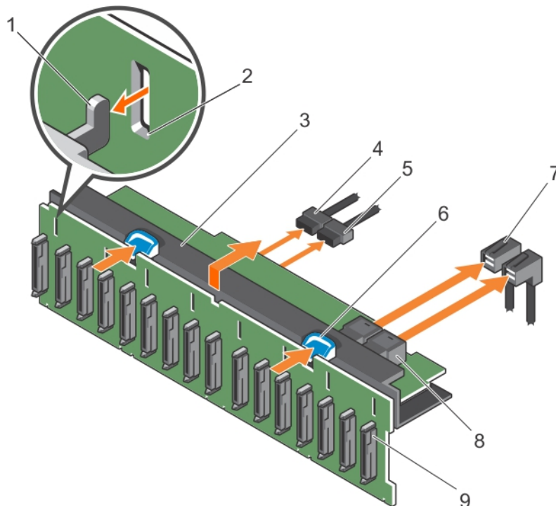
Figure 81. Retrait du fond de panier SAS/SATA (x16) de 2,5 pouces
