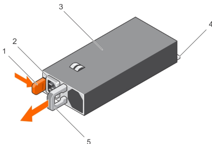
Figure 40. Retrait d'un bloc d'alimentation (PSU) CA
