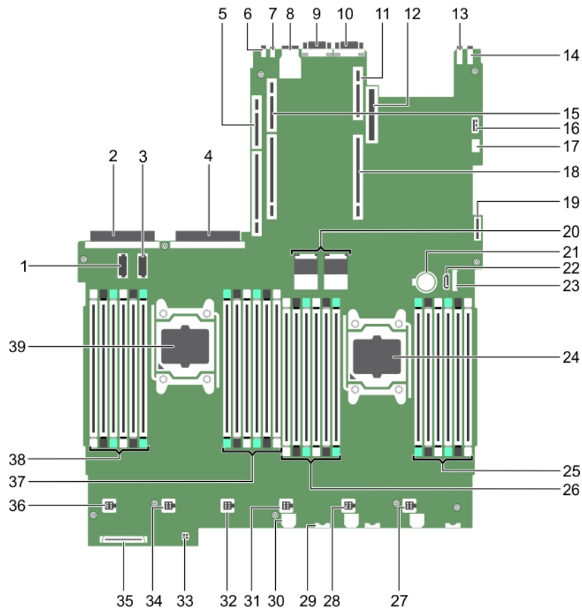
Figure 96. Connecteurs de la carte système
