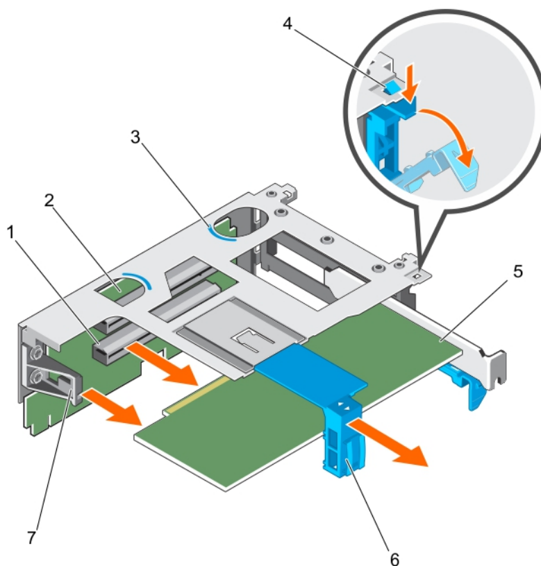
Figure 53. Retrait d'une carte d'extension de la carte de montage pour carte d'extension 1
