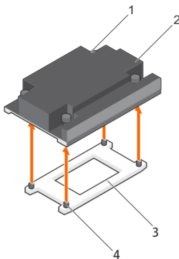
Figure 32. Retrait d'un dissipateur de chaleur
