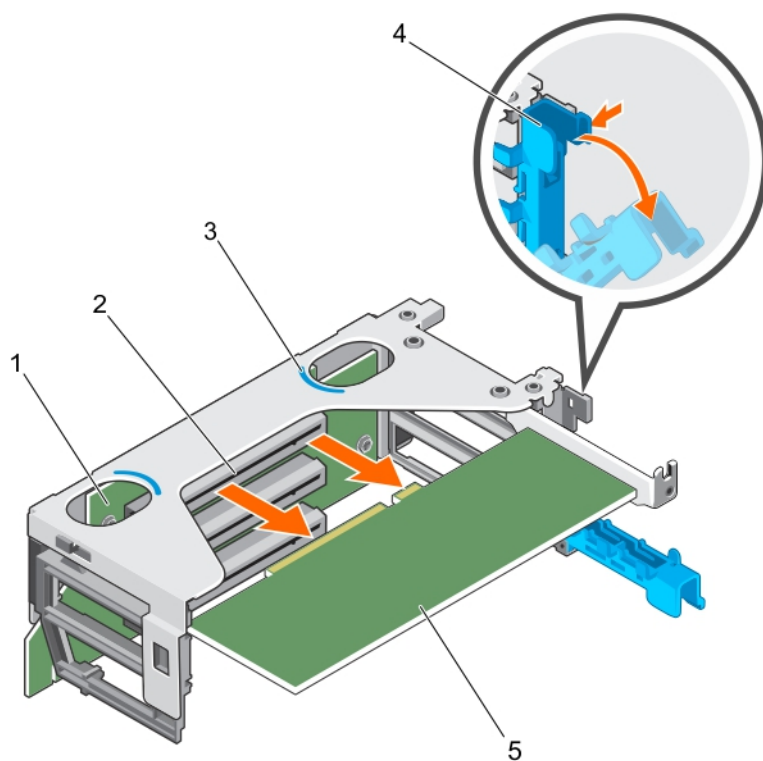
Figure 55. Retrait d'une carte d'extension de la carte de montage pour carte d'extension 2
