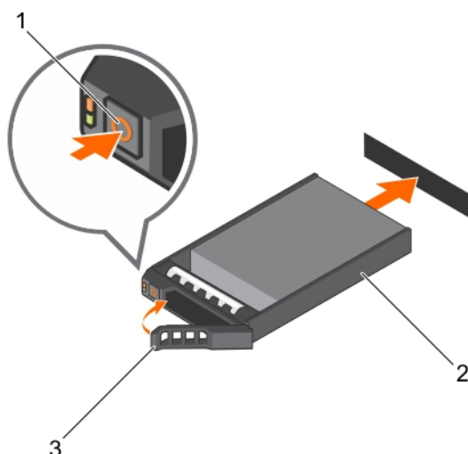
Figure 72. Installation d'un disque dur ou SSD remplaçable à chaud
