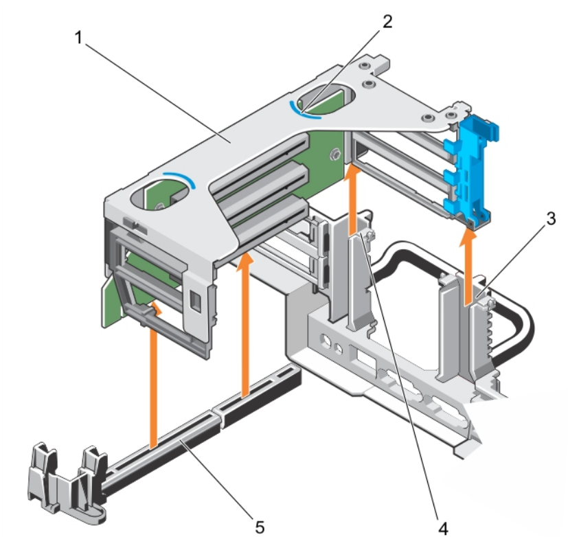
Figure 46. Retrait de la carte de montage pour carte d'extension 2
