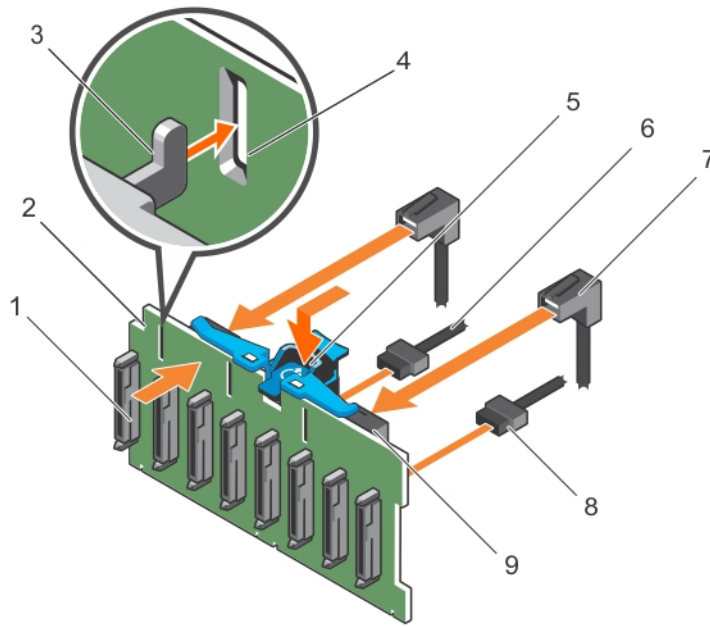
Figure 86. Installation du fond de panier SAS/SATA de 2,5 pouces (x8)
