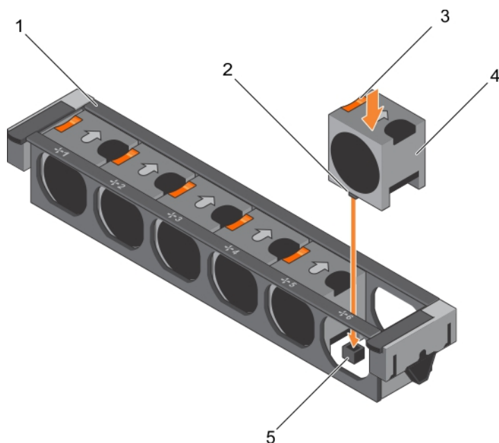
Figure 25. Installation d'un ventilateur de refroidissement
