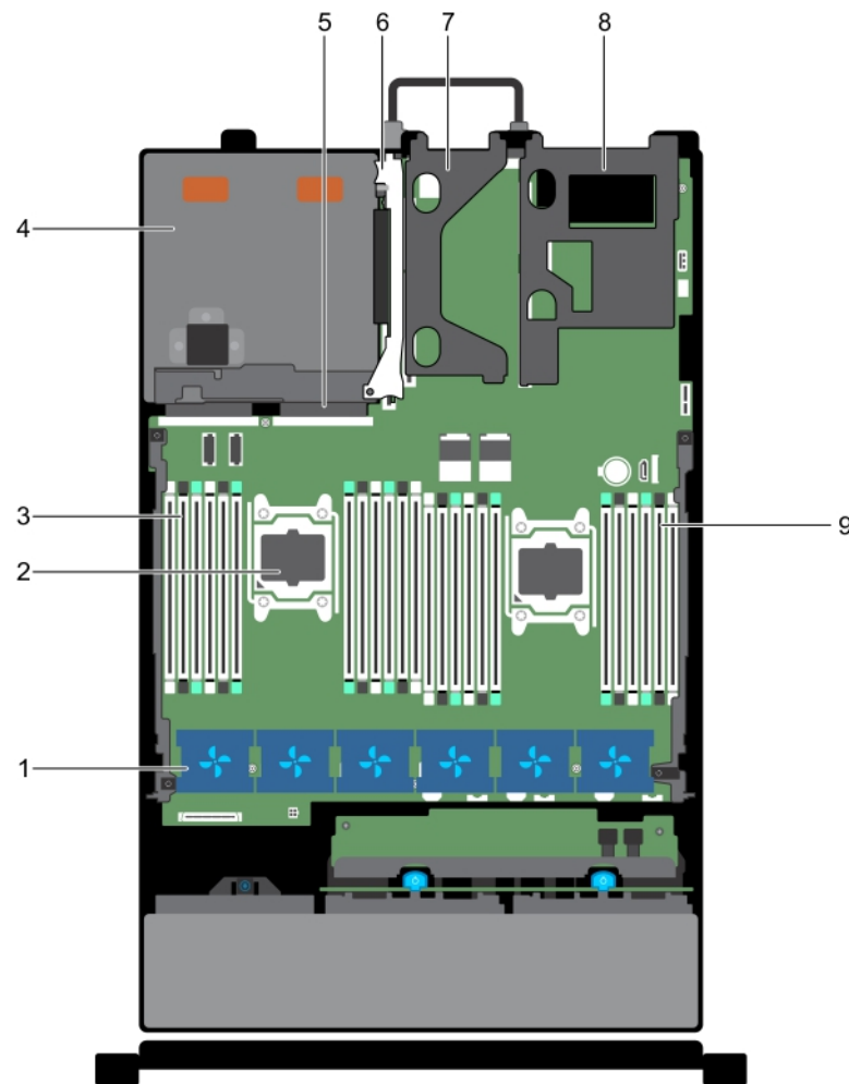
Figure 14. Intérieur du système — Système à deux processeurs
