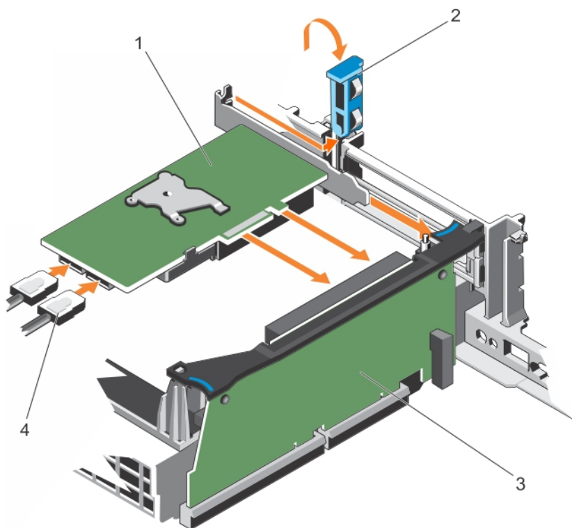
Figure 43. Installation de la carte contrôleur de stockage intégrée
