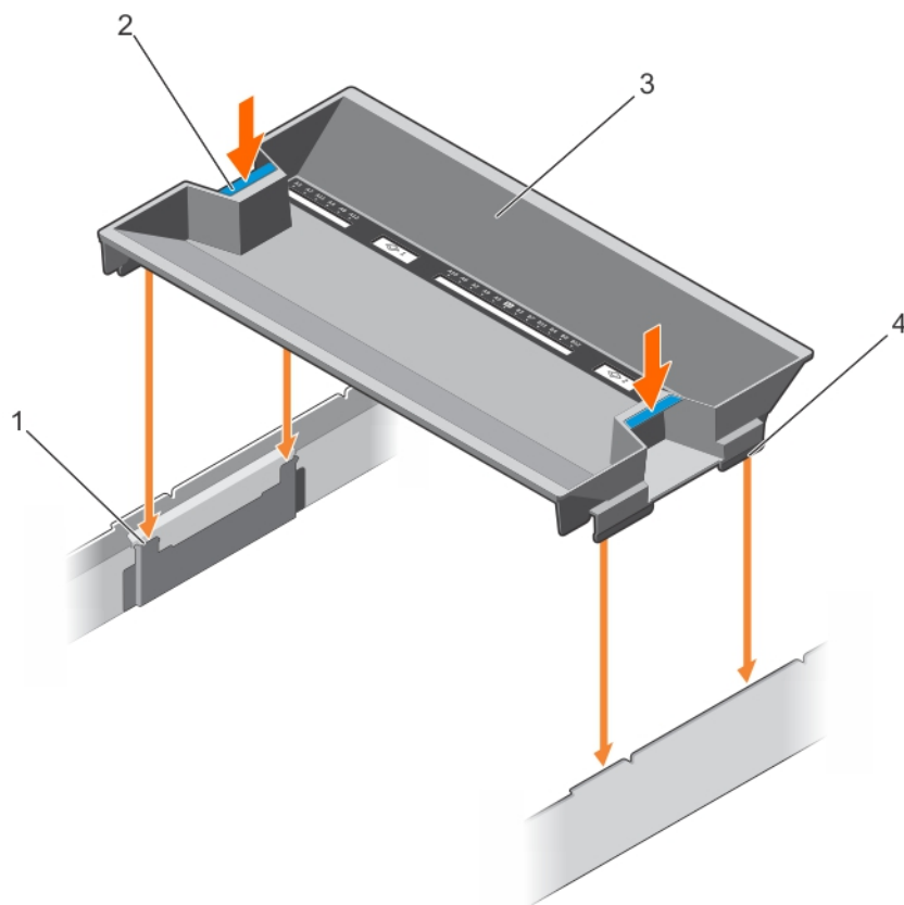
Figure 23. Installation du carénage de refroidissement
