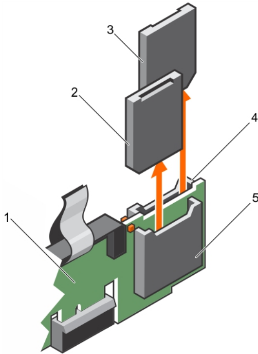
Figure 61. Retrait d'une carte SD interne
