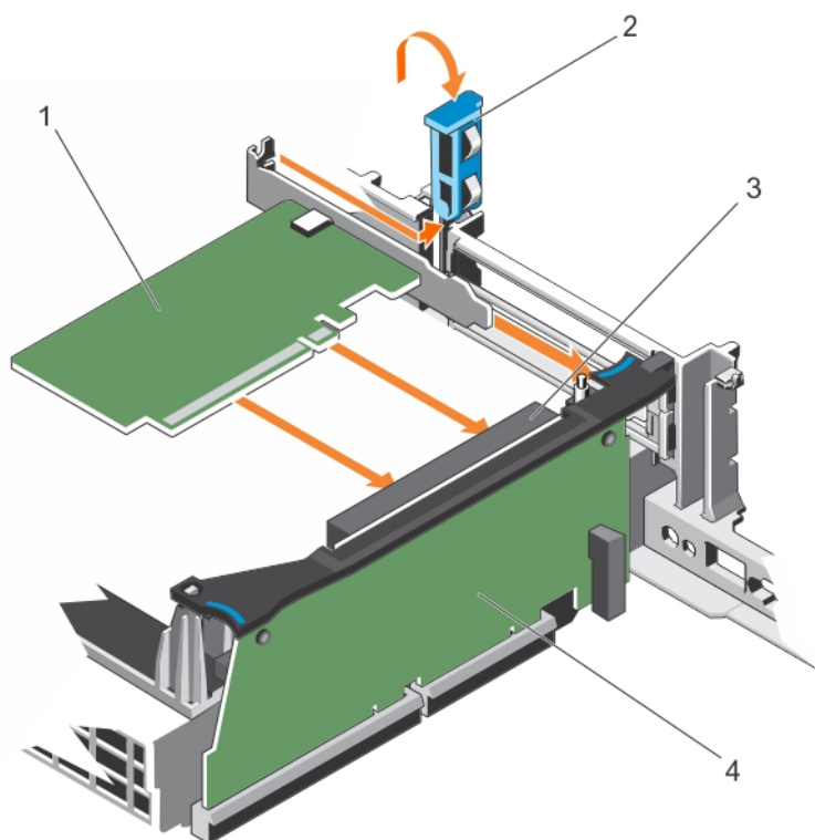
Figure 59. Installation d'une carte d'extension mi-hauteur dans la carte de montage pour carte d'extension 3
