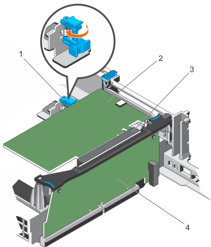
Figure 60. Installation d'une carte d'extension pleine hauteur dans la carte de montage pour carte d'extension 3
