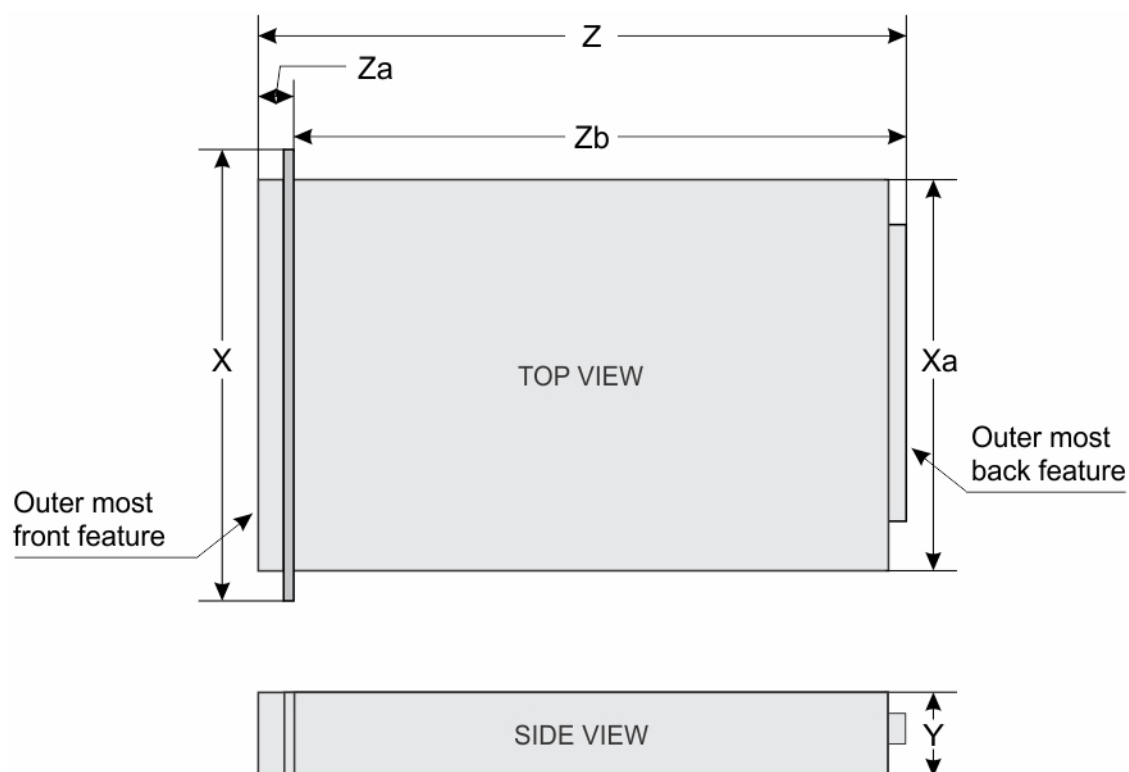
Figure 9. Dimensions du système PowerEdge R830
