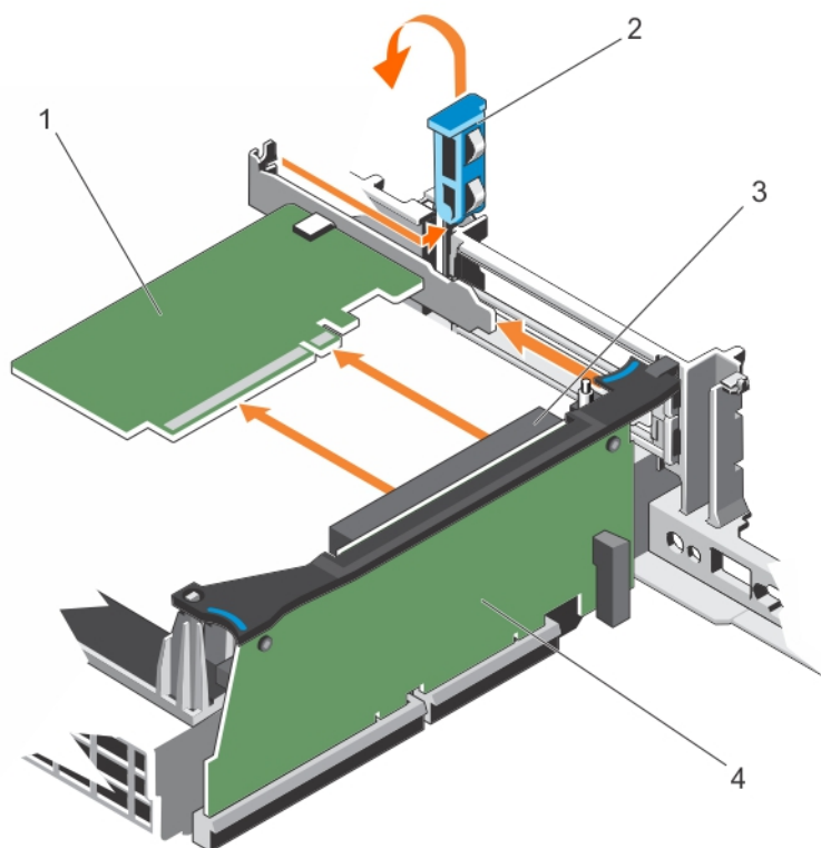
Figure 57. Retrait d'une carte d'extension mi-hauteur de la carte de montage de carte d'extension 3
