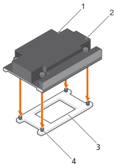
Figure 37. Installation du dissipateur de chaleur
