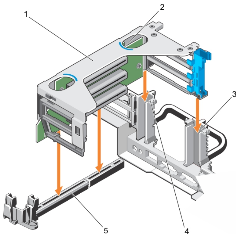
Figure 51. Installation de la carte de montage pour carte d'extension 2
