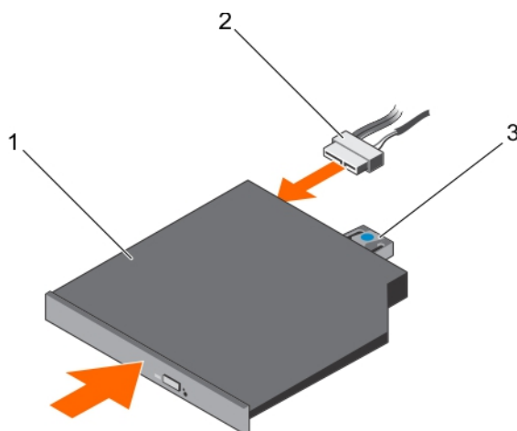
Figure 78. Installation du lecteur optique en option
