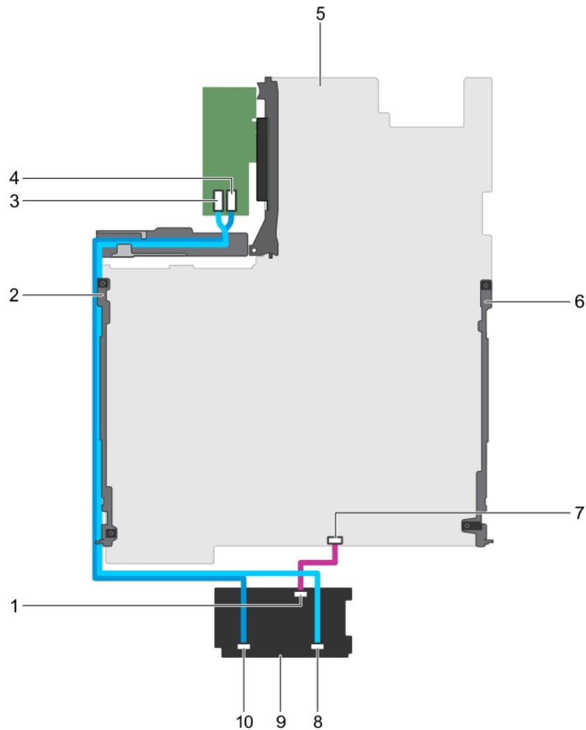
Figure 84. Schéma de câblage : fond de panier SAS/SATA de 2,5 pouces (x8)
