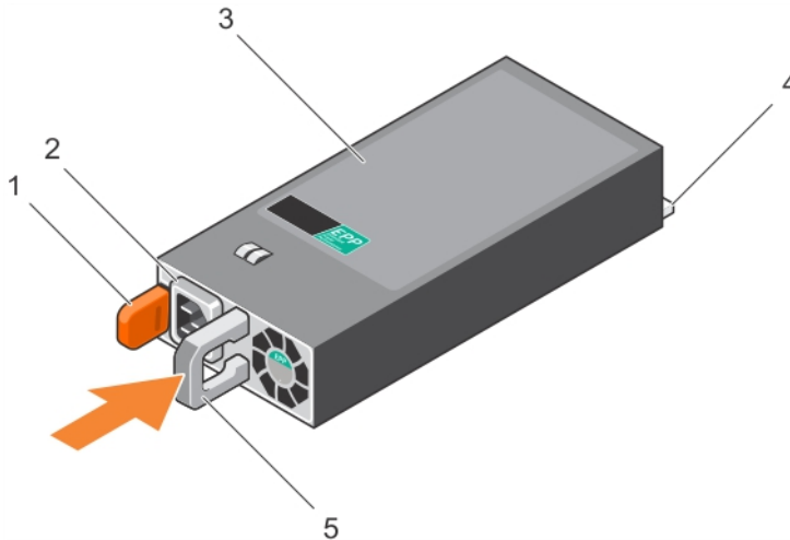
Figure 41. Installation d'un bloc d'alimentation (PSU) CA
