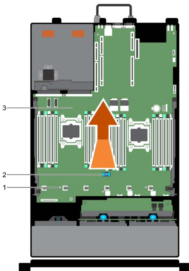
Figure 94. Retrait de la carte système
