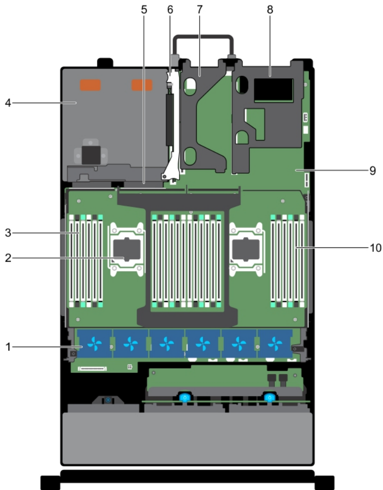
Figure 15. Intérieur du système — Système à quatre processeurs avec module d'extension de processeur (PEM)
