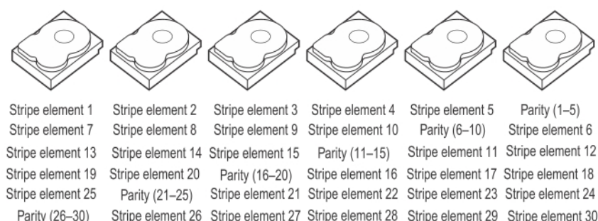
Figure 26. Exemple de parité distribuée (RAID 5)
