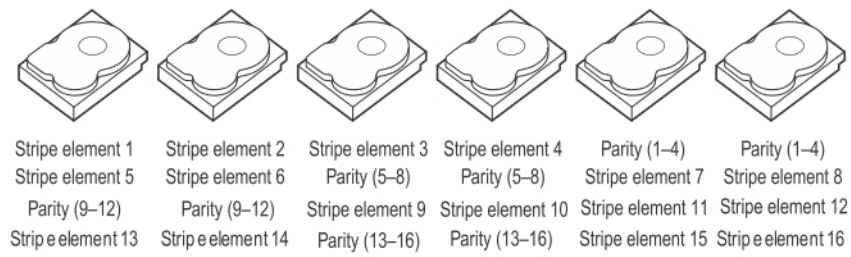
Figure 27. Exemple de parité distribuée double (RAID 6)
