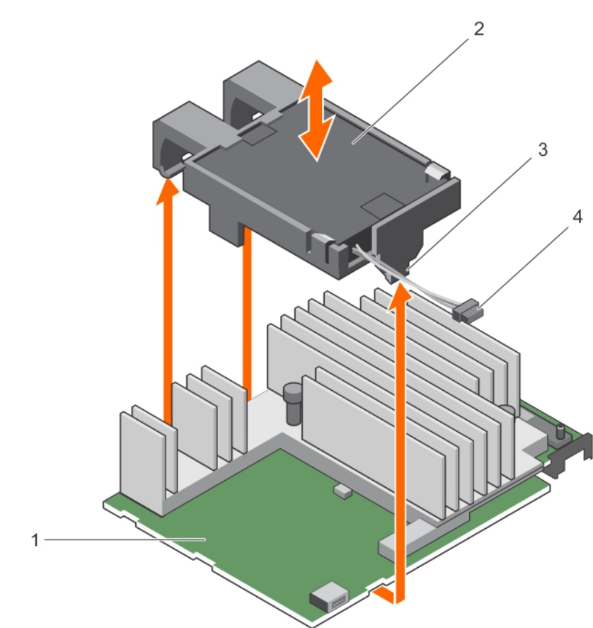
Figure 12. Retrait du support de la batterie
