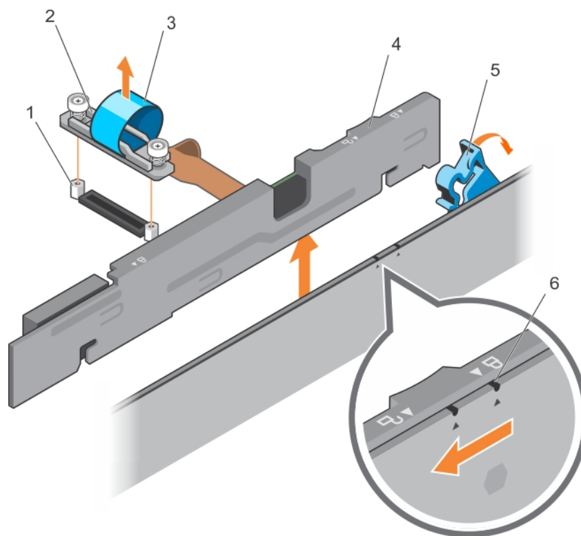
Figure 14. Retrait et installation d'une carte H730P Slim
