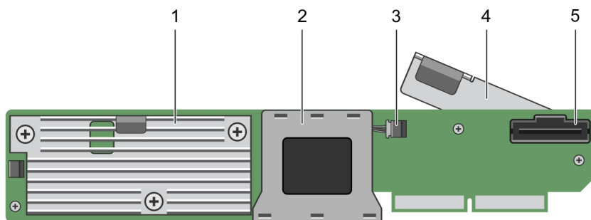
Figure 5. Caractéristiques de la carte d'extension PERC H730P MX
