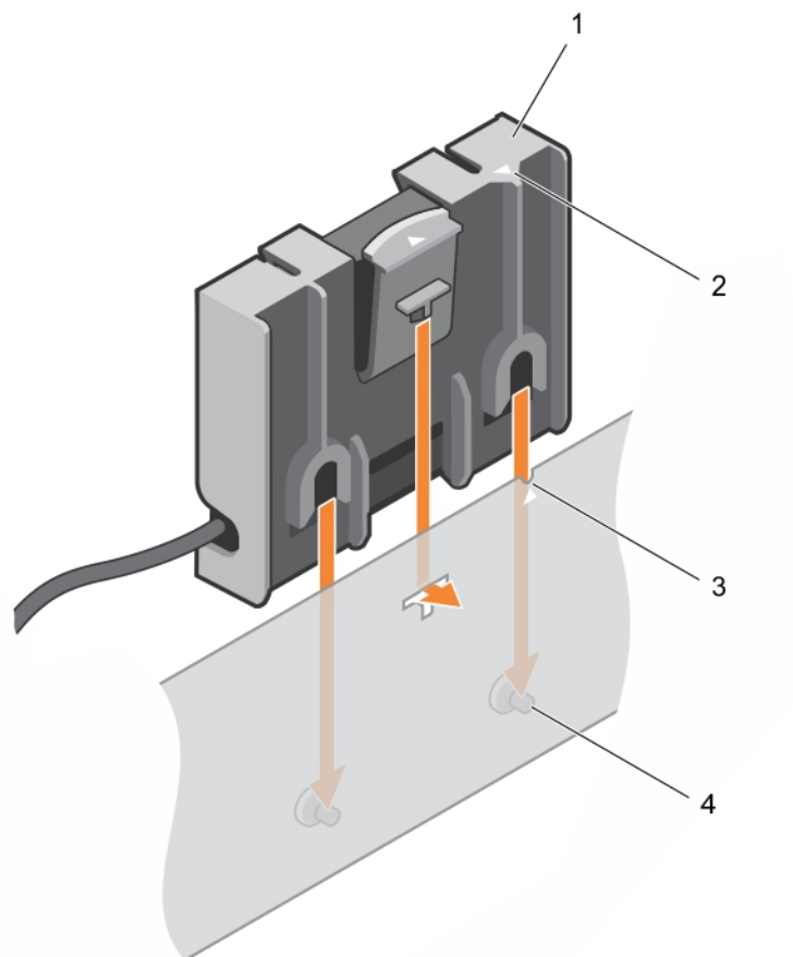
Figure 20. Remise en place du support de la batterie
