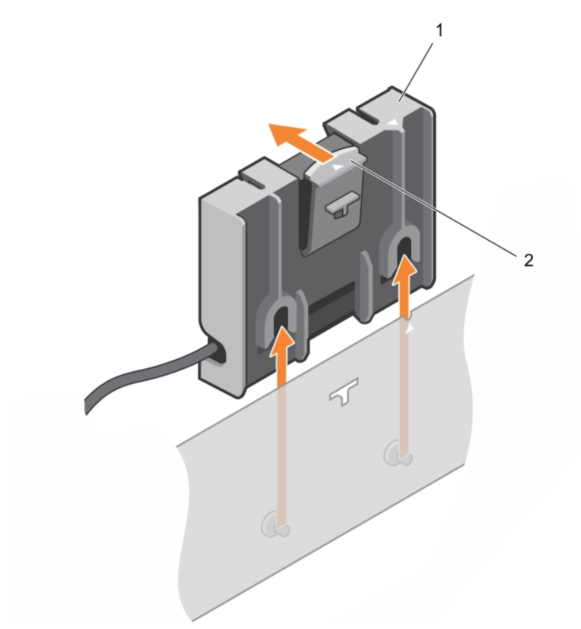
Figure 17. Retrait du support de la batterie
