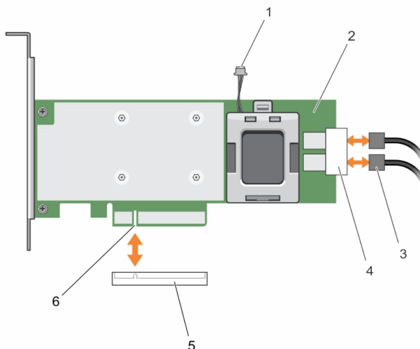
Figure 10. Retrait et installation de la carte PERC 9
