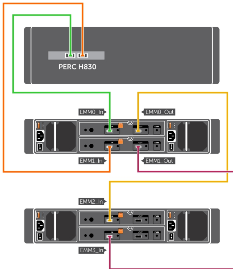
Figure 8. Ports de carte PERC H830
