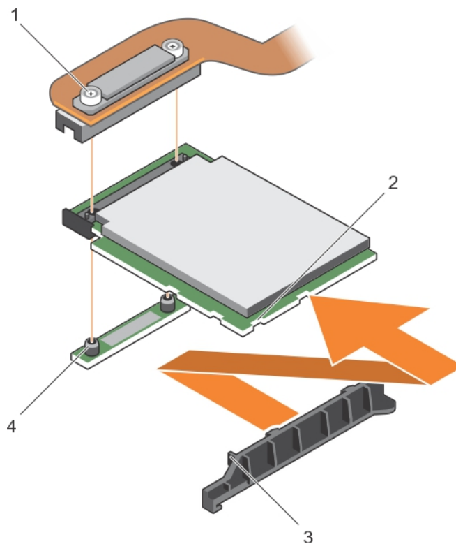
Figure 16. Retrait et installation du contrôleur mini-lame PERC 9
