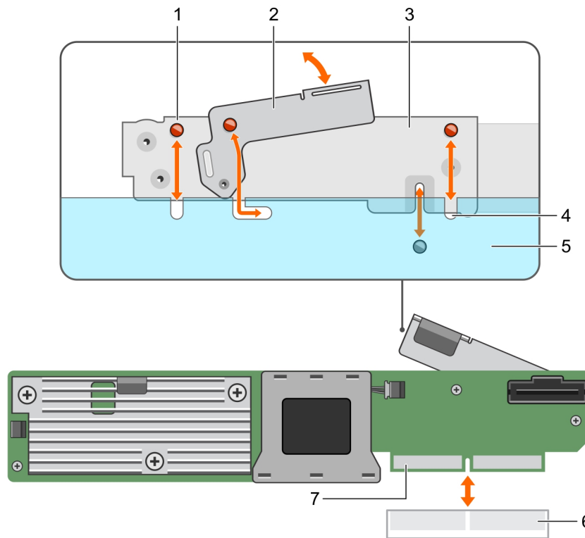
Figure 9. Retrait et installation de la carte d'extension de carte PERC H730P MX
