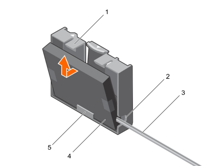
Figure 18. Retrait de la batterie de son support
