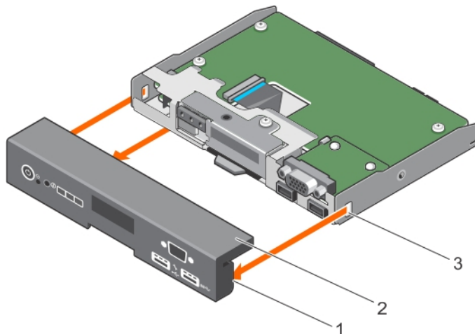
Figure 99. Retrait du capot du panneau de commande pour des systèmes équipés d'écran LCD
