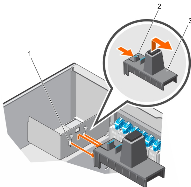
Figure 63. Retrait du support de carte d'extension
