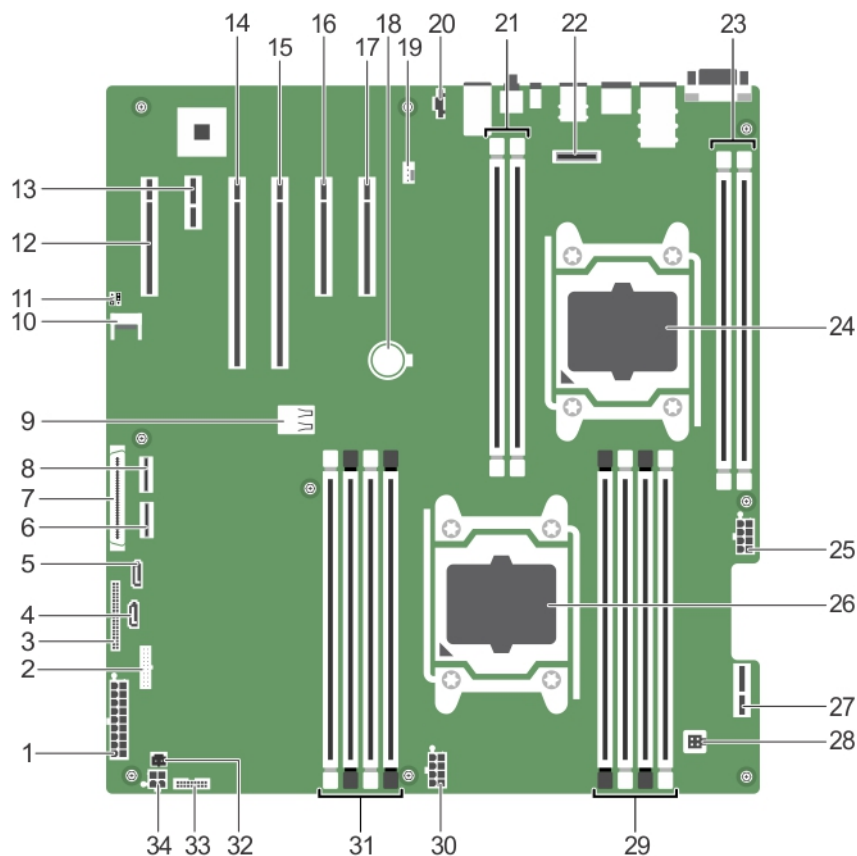
Figure 118. Connecteurs de la carte système
