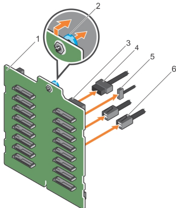
Figure 46. Retrait d'un fond de panier de disques durs x16
