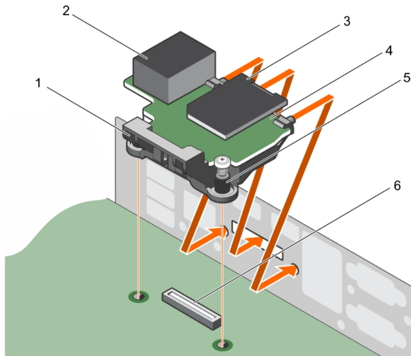
Figure 72. Installation de la carte des ports iDRAC
