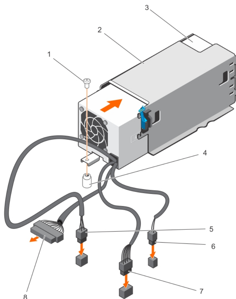
Figure 91. Installation d'un bloc d'alimentation câblé
