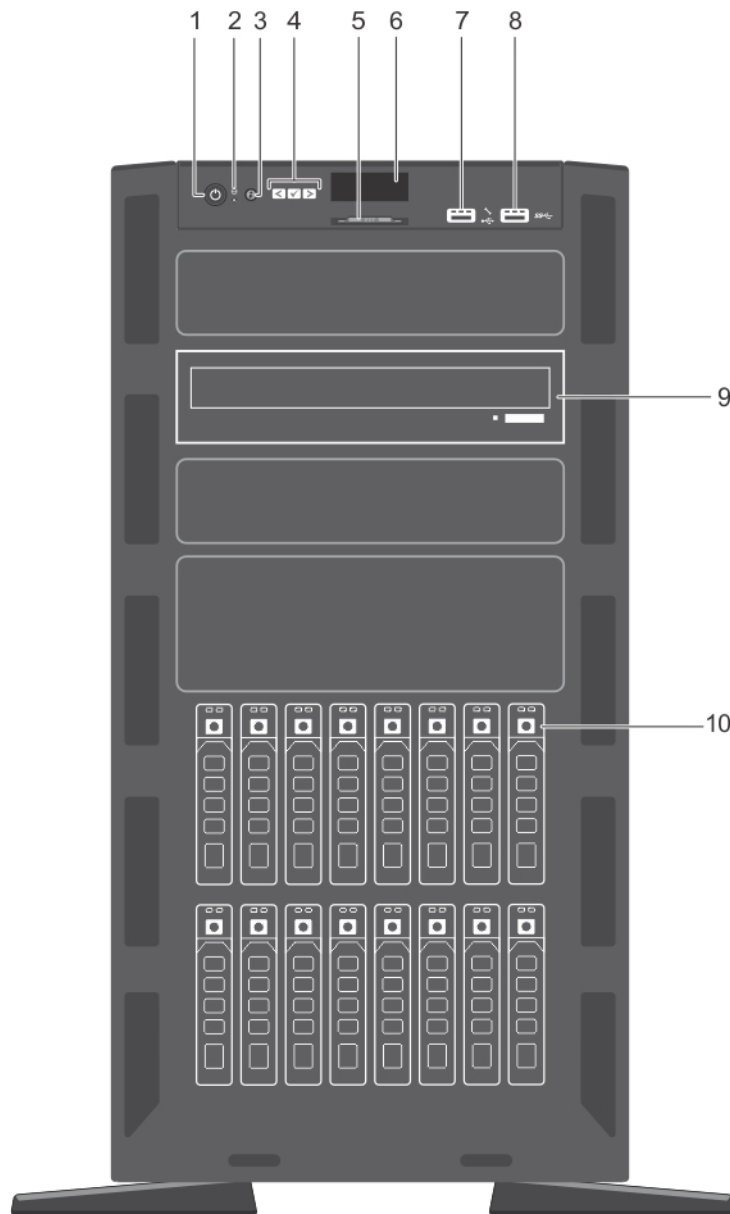
Figure 2. Fonctions du panneau avant d'un châssis de 16 disques durs de 2,5 pouces remplaçables à chaud
