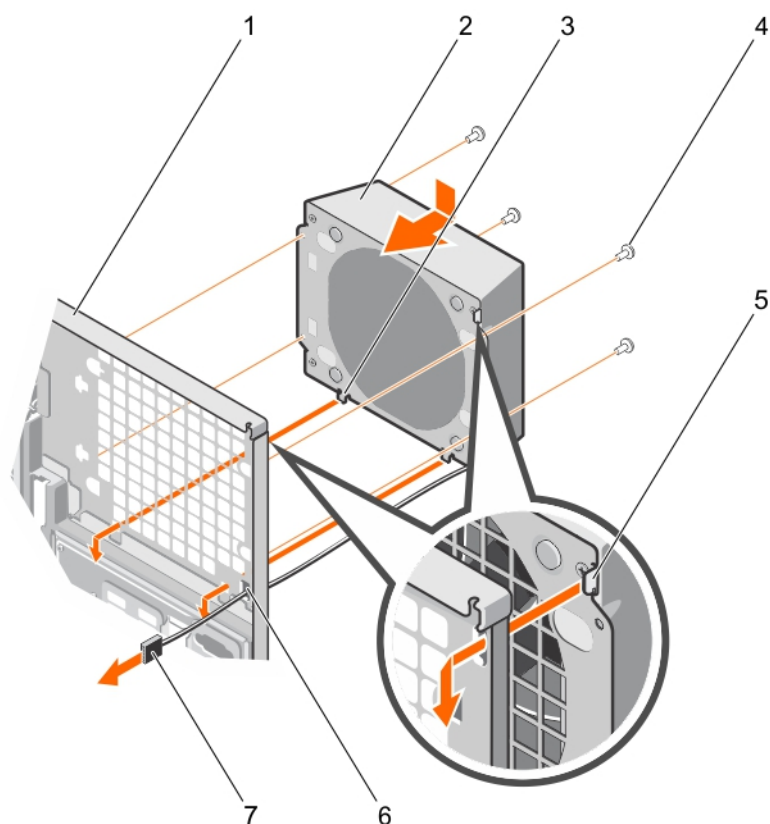
Figure 60. Installation du ventilateur de refroidissement externe
