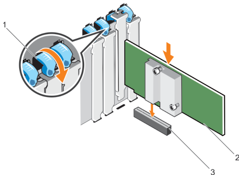
Figure 67. Installation d'une carte d'extension
