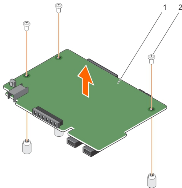
Figure 104. Retrait et installation du panneau de commande pour des systèmes équipés de disques durs remplaçables à chaud
