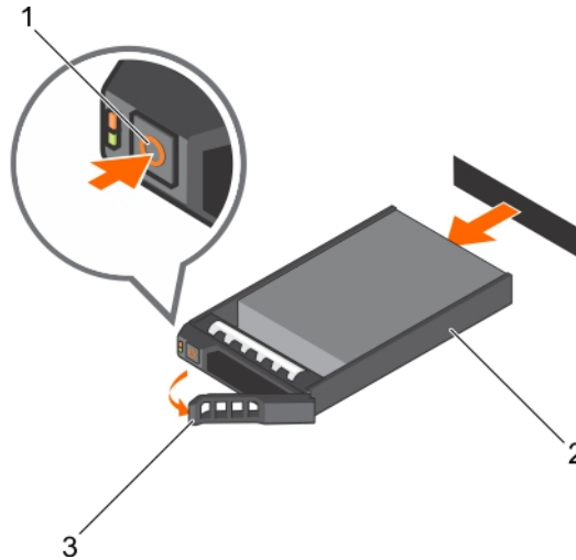
Figure 29. Retrait d'un disque dur ou SSD remplaçable à chaud
