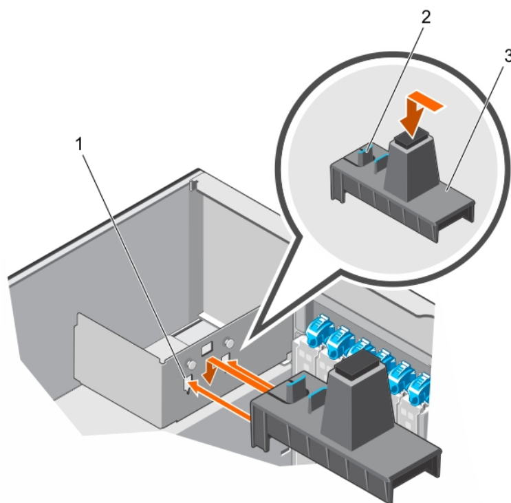
Figure 64. Installation du support de carte d'extension
