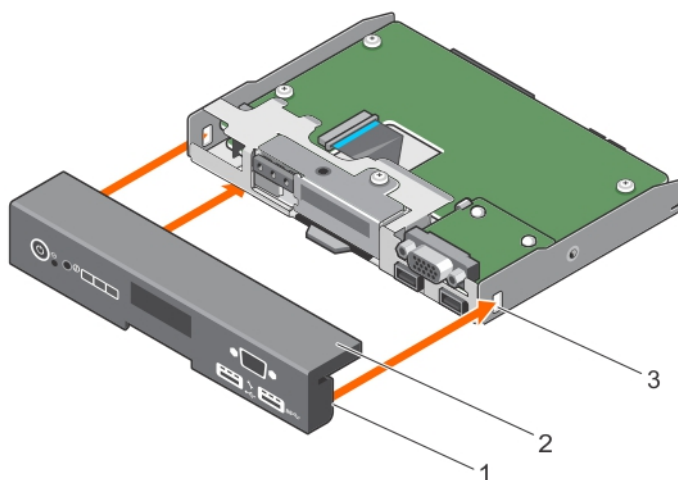
Figure 101. Installation du capot du panneau de commande pour des systèmes équipés d'écran LCD
