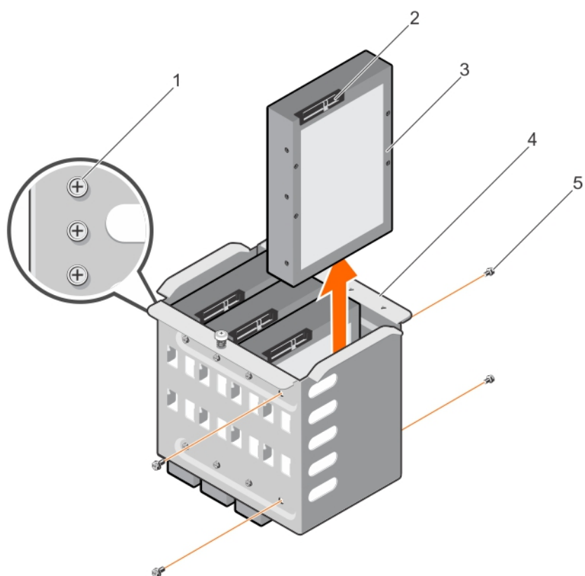
Figure 42. Retrait d'un disque dur câblé
