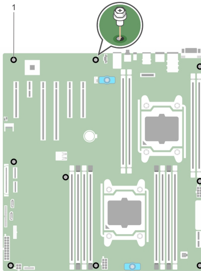
Figure 114. Installation des vis sur la carte système
