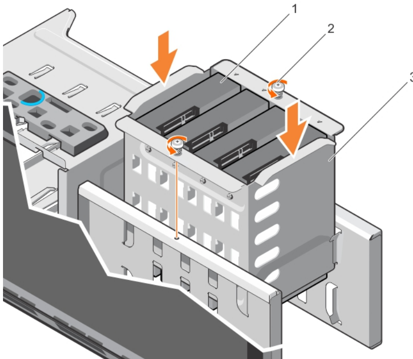
Figure 41. Installation de la baie de disque dur interne
