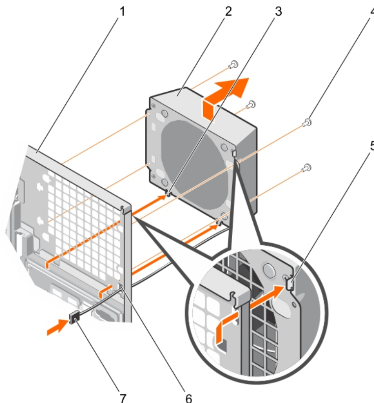
Figure 59. Retrait du ventilateur de refroidissement externe
