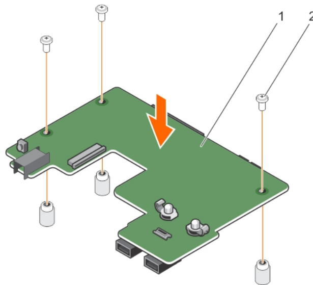
Figure 105. Installation de la carte du panneau de commande pour des systèmes équipés de disques durs remplaçables à chaud
