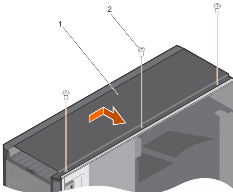
Figure 116. Retrait du capot supérieur du système
