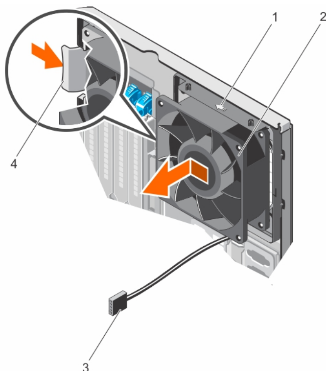
Figure 57. Retrait du ventilateur de refroidissement interne
