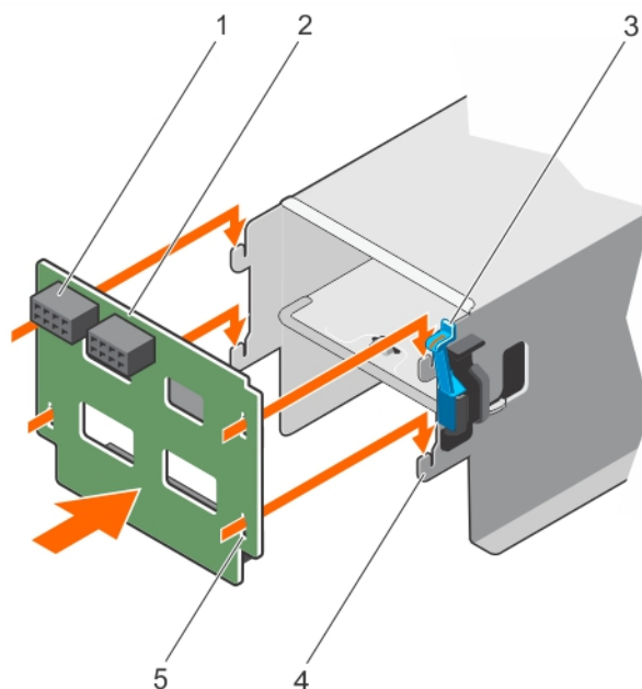
Figure 93. Installation de la carte intercalaire d'alimentation
