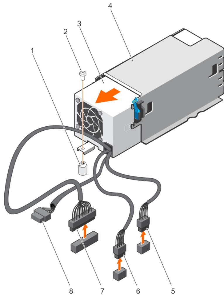
Figure 89. Retrait d'un bloc d'alimentation câblé
