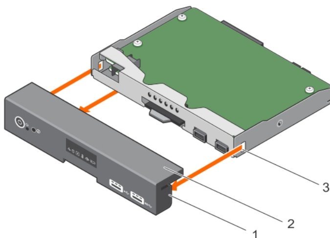
Figure 100. Retrait du capot du panneau de commande pour des systèmes équipés d'écran LED
