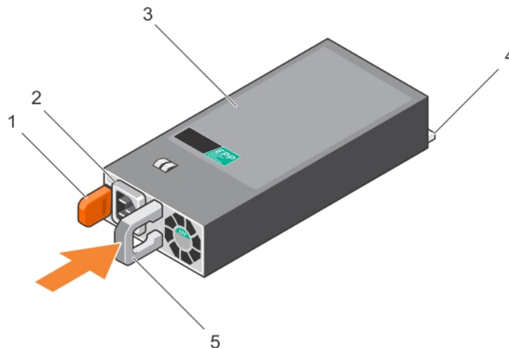
Figure 85. Installation d'un bloc d'alimentation redondant
