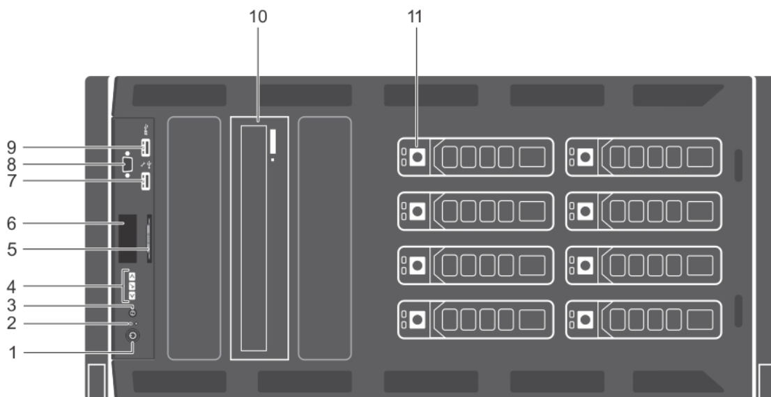
Figure 4. Fonctions du panneau avant d'un châssis de 8 disques durs de 3,5 pouces remplaçables à chaud en mode rack
