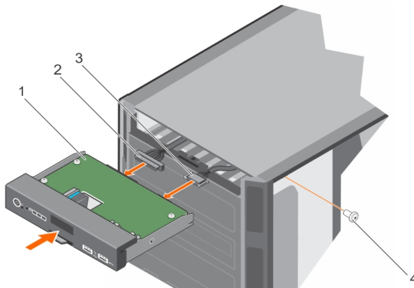
Figure 98. Installation du panneau de commande
