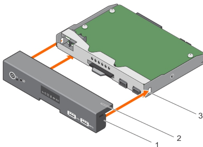
Figure 102. Installation du capot du panneau de commande pour des systèmes équipés d'écran LED
