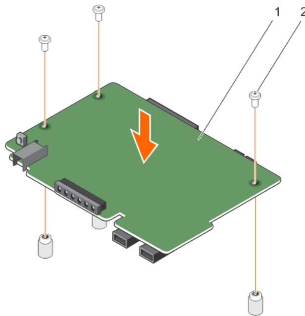
Figure 106. Installation du panneau de commande pour des systèmes équipés de disques durs câblés
