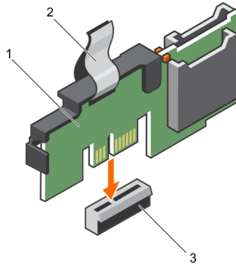
Figure 76. Installation du module SD interne double en option
