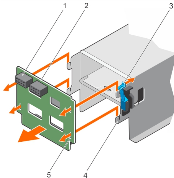
Figure 92. Retrait et installation de la carte intercalaire d'alimentation
