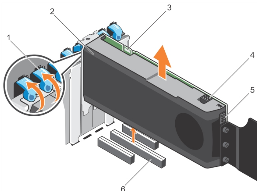
Figure 69. Retrait d'une carte GPU
