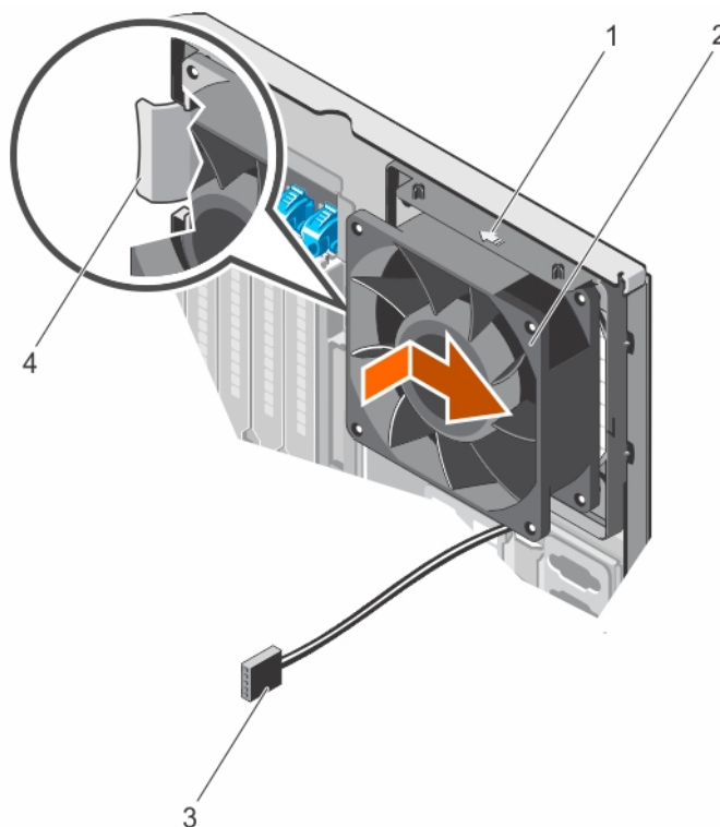
Figure 58. Installation du ventilateur de refroidissement interne
