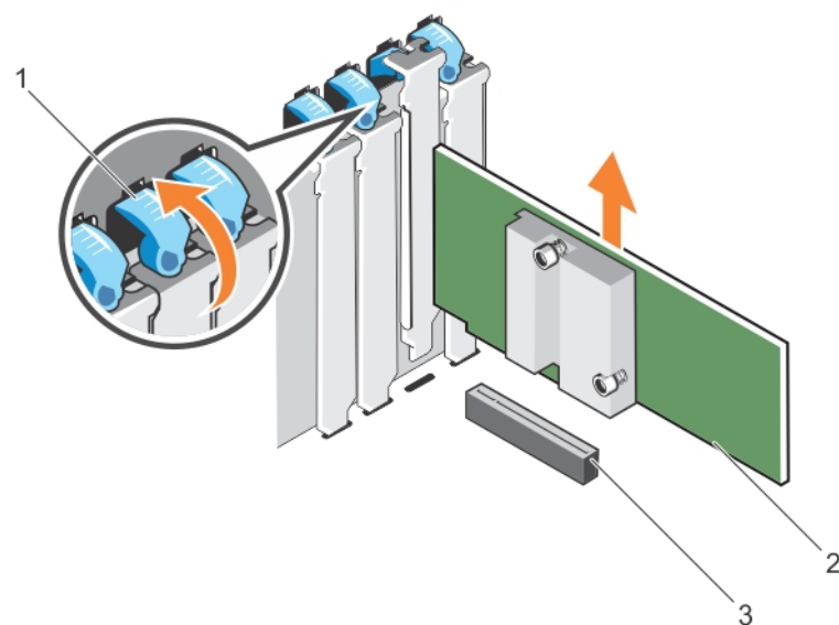
Figure 65. Retrait d'une carte d'extension
