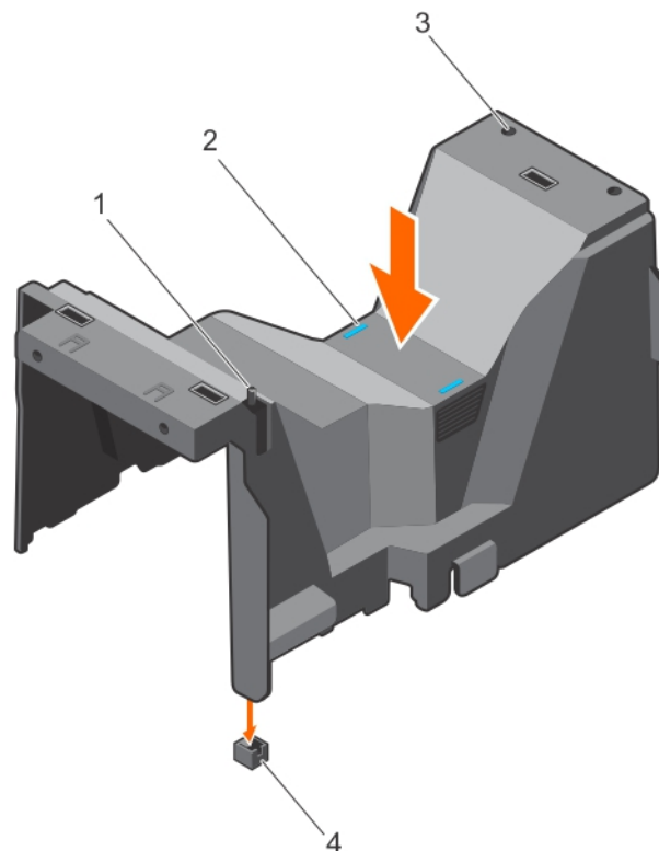
Figure 28. Installation du carénage de refroidissement
