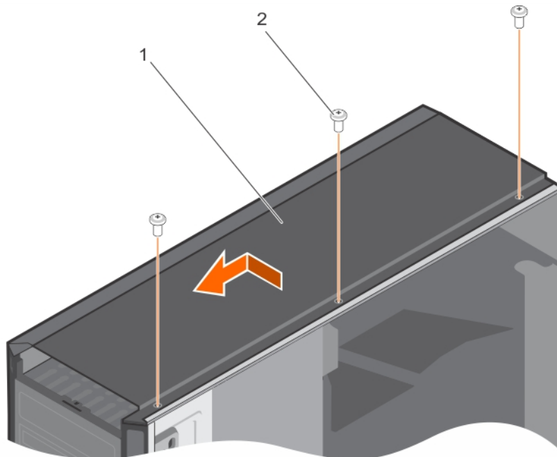
Figure 117. Installation du capot supérieur du système
