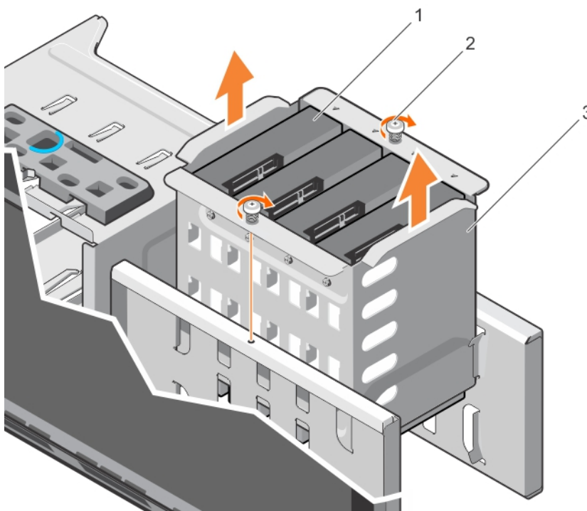
Figure 40. Retrait de la baie de disque dur interne
