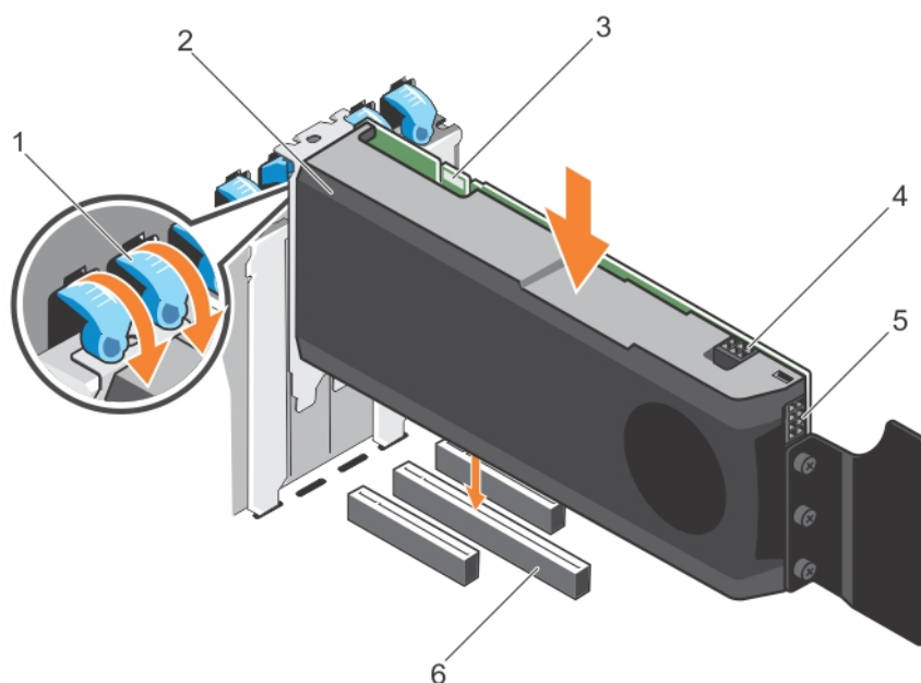
Figure 70. Installation d'une carte GPU
