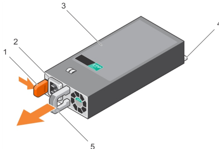
Figure 84. Retrait d'un bloc d'alimentation (PSU) CA
