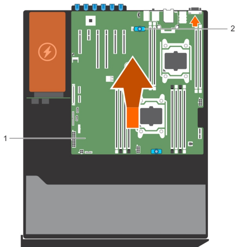
Figure 113. Installation de la carte système
