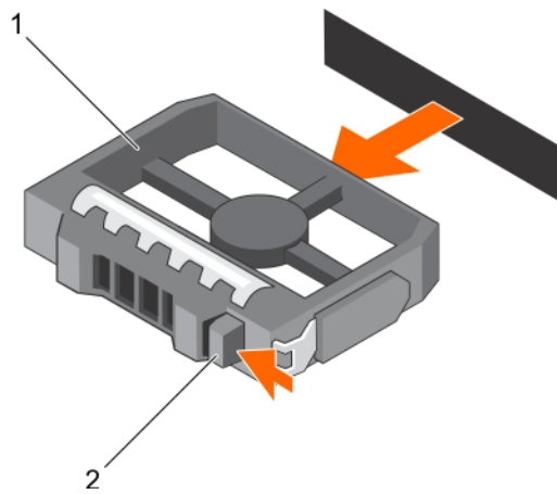
Figure 32. Retrait d'un cache de disque dur de 2,5 pouces
