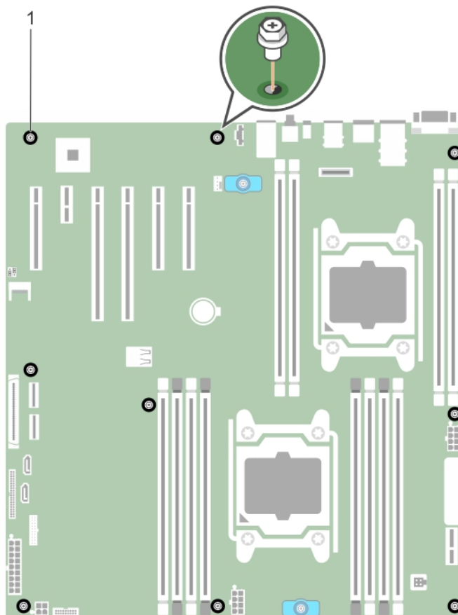
Figure 111. Retrait des vis sur la carte système.\
