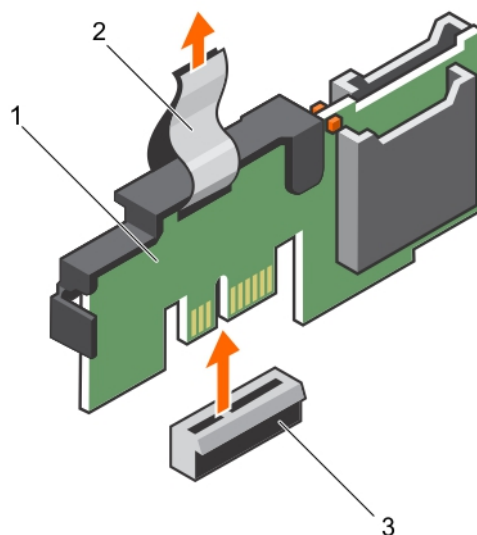
Figure 75. Retrait du module SD interne double (IDSDM)
