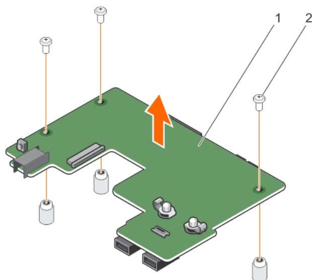
Figure 103. Retrait de la carte du panneau de commande de systèmes équipés de disques durs remplaçables à chaud
