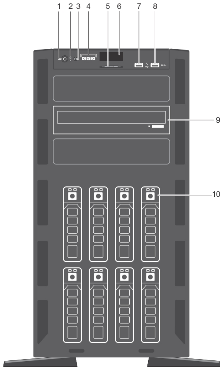
Figure 3. Fonctions du panneau avant d'un châssis de 8 disques durs de 3,5 pouces remplaçables à chaud
