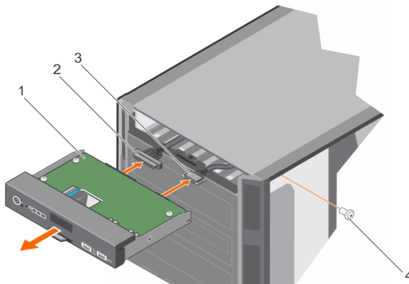
Figure 96. Retrait de l'assemblage du panneau de commande
