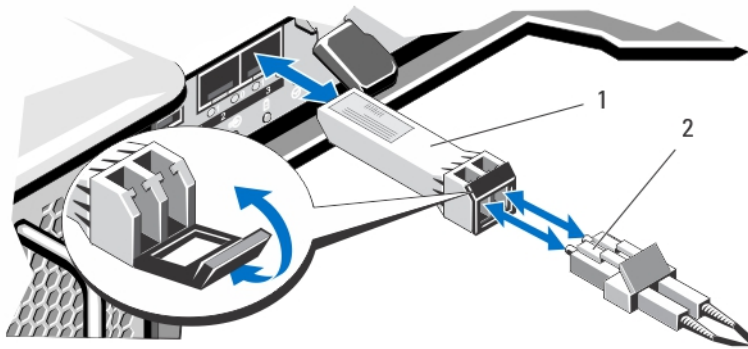
Figure 27. Retrait d'un module SFP
