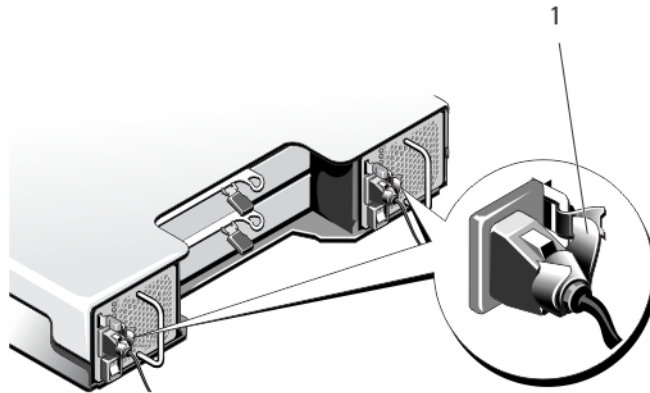
Figure 21. Fixation du câble d'alimentation
