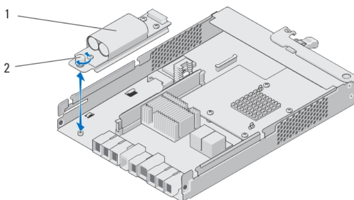
Figure 19. Retrait et installation de l'unité de batterie de secours du module de contrôleur RAID
