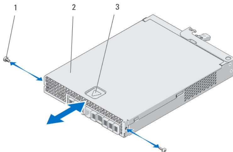
Figure 18. Ouverture et fermeture du module de contrôleur RAID
