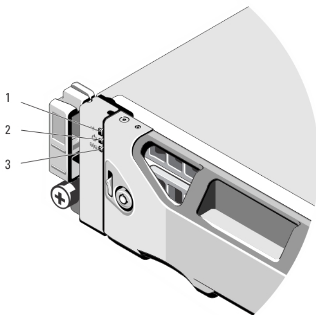
Figure 3. Fonctions et voyants du cadre avant
