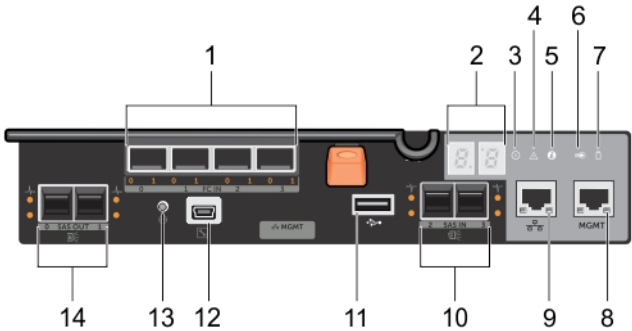
Figure 7. Module de contrôleur RAID Fibre Channel MD3800f et MD3820f Series
