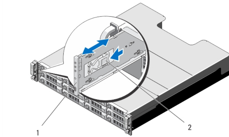
Figure 20. Retrait et installation du panneau de commande : PowerVault MD3800i
