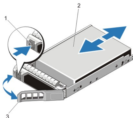
Figure 11. Retrait et installation d'un disque physique remplaçable à chaud
