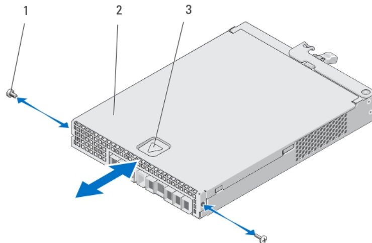
Figure 16. Ouverture et fermeture du module de contrôleur RAID
