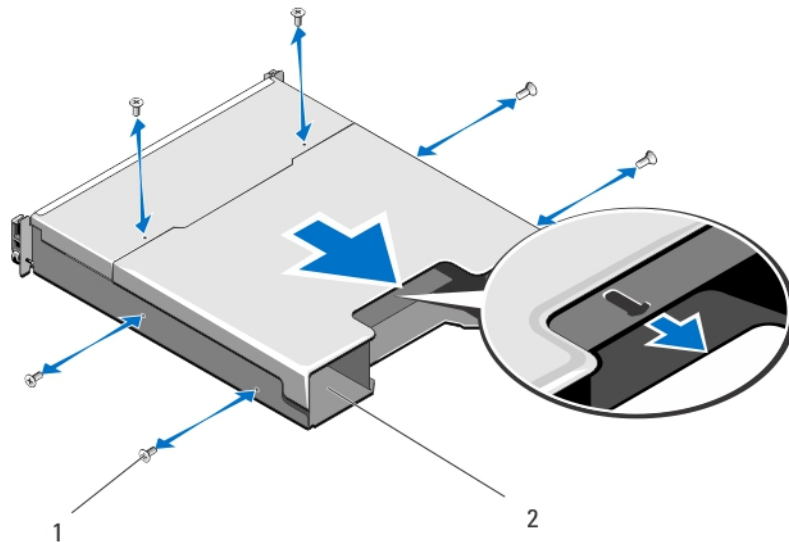
Figure 22. Retrait et installation du bâti du bloc d'alimentation/module de contrôleur RAID
