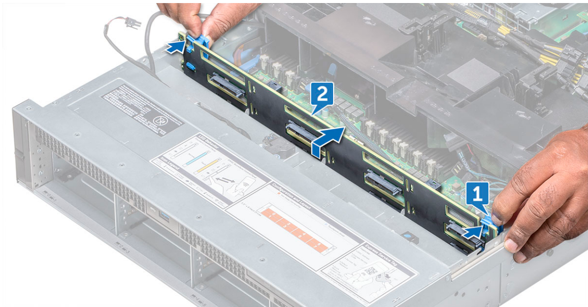
Figure 23. Retrait du fond de panier de disque dur
