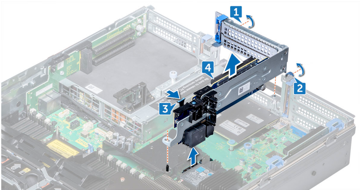
Figure 21. Retrait de la carte de montage pour carte d'extension 2A
