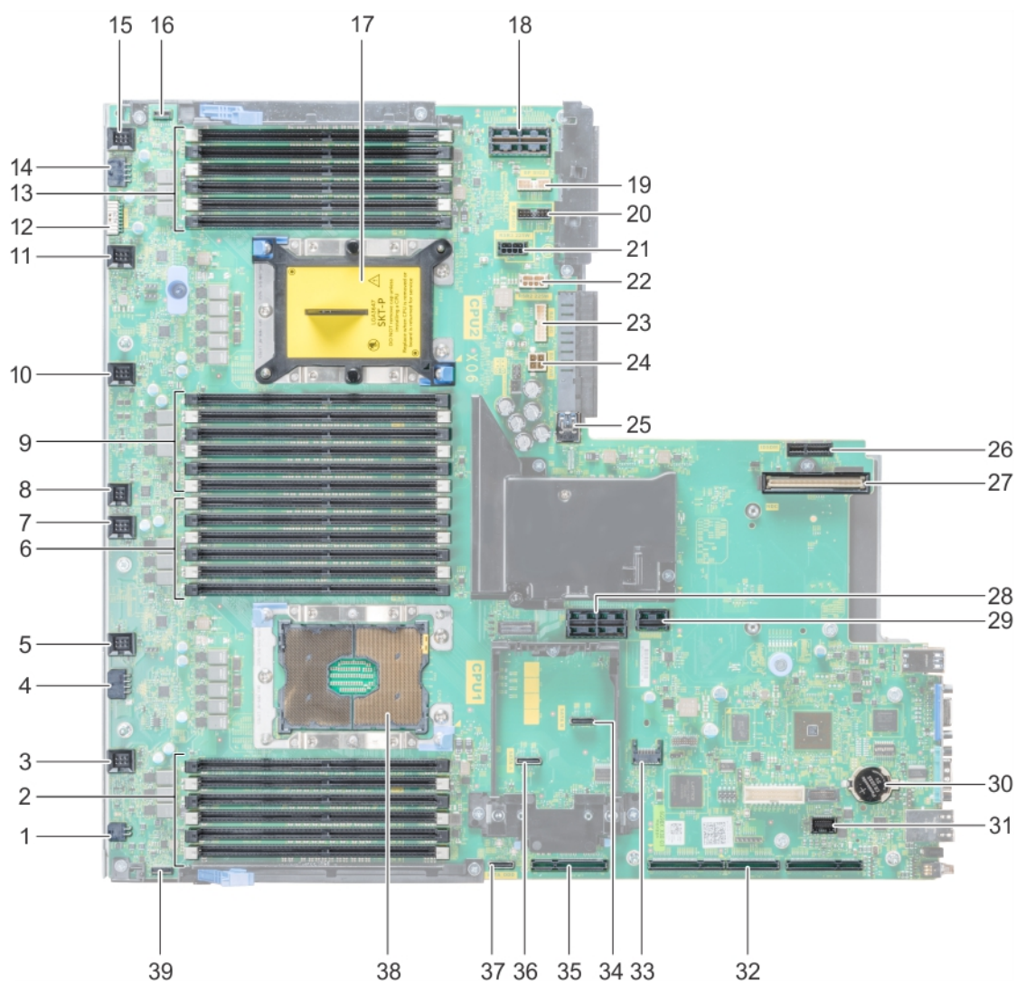
Figure 10. Connecteurs et cavaliers de la carte système
