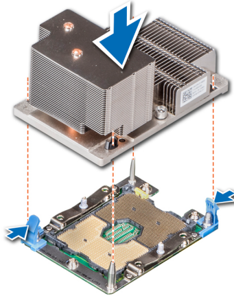
Figure 16. Installation du module du processeur et du dissipateur de chaleur (2U)
