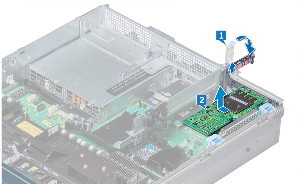
Figure 17. Retrait d'une carte d'extension de la carte de montage pour carte d'extension 1
