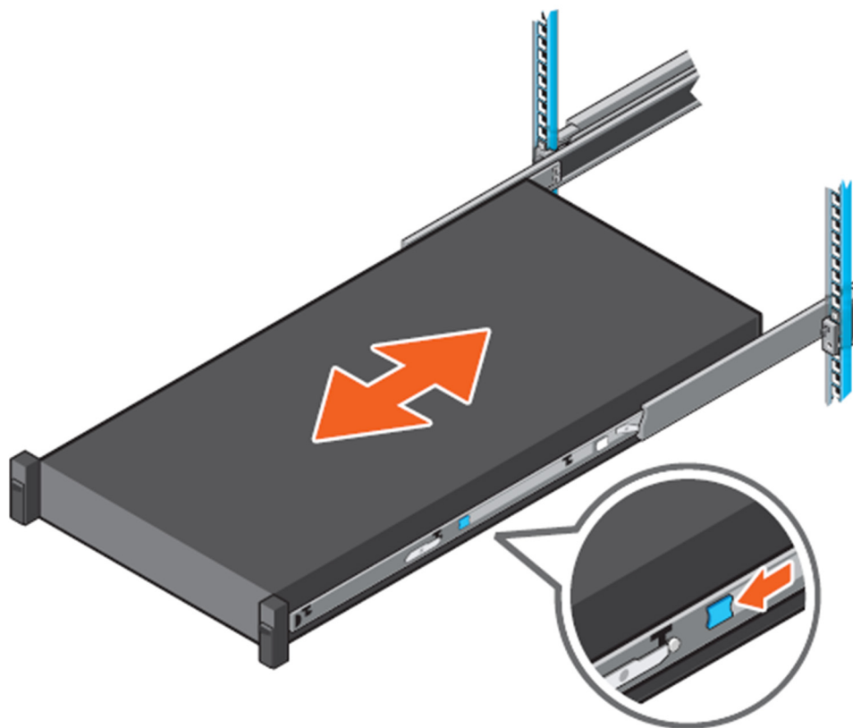
Figure 27. Glissement du système dans le rack
