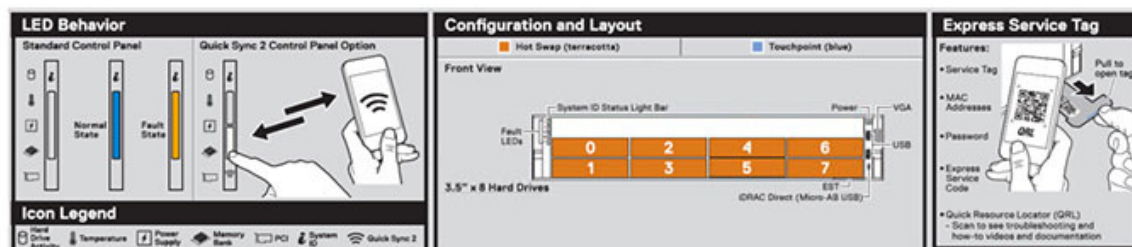
Figure 3. Comportement des voyants LED, numéro de service express, configuration et disposition
