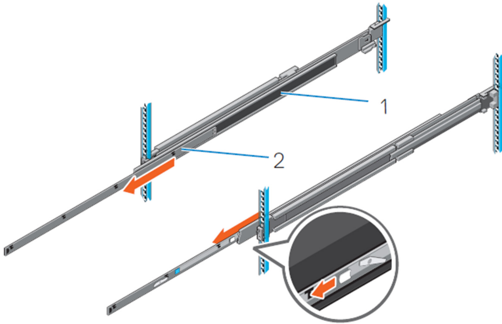
Figure 28. Dégagement du rail intermédiaire
