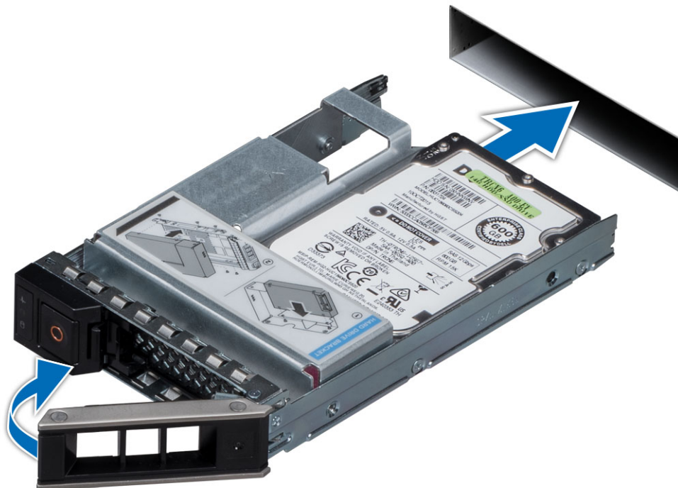
Figure 12. Installation du disque dur
