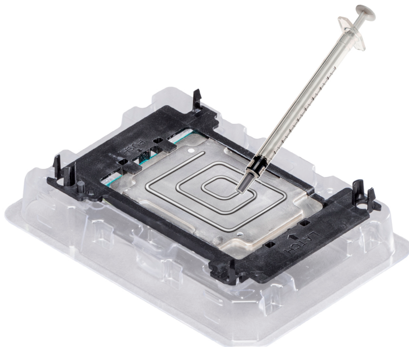
Figure 15. Application de graisse thermique sur la partie supérieure du processeur
