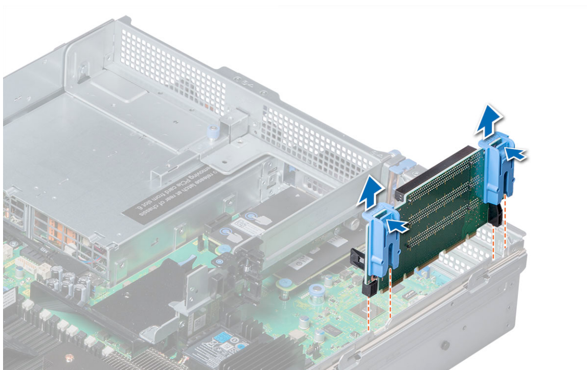
Figure 20. Retrait de la carte de montage 1 pour carte d'extension
