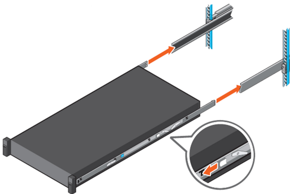
Figure 30. Installation du système sur les rails étendus
