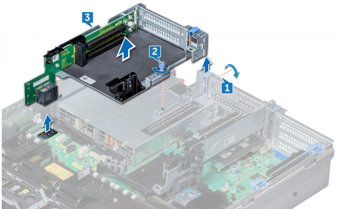
Figure 22. Retrait de la carte de montage pour carte d'extension 3
