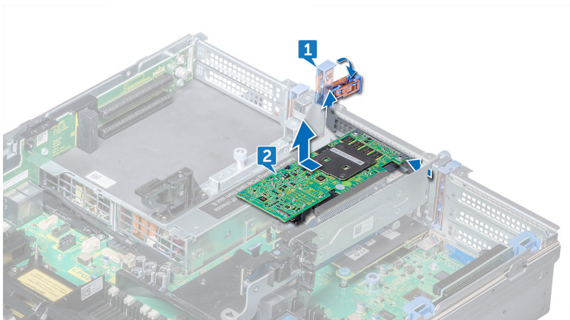
Figure 18. Retrait d'une carte d'extension de la carte de montage pour carte d'extension 2
