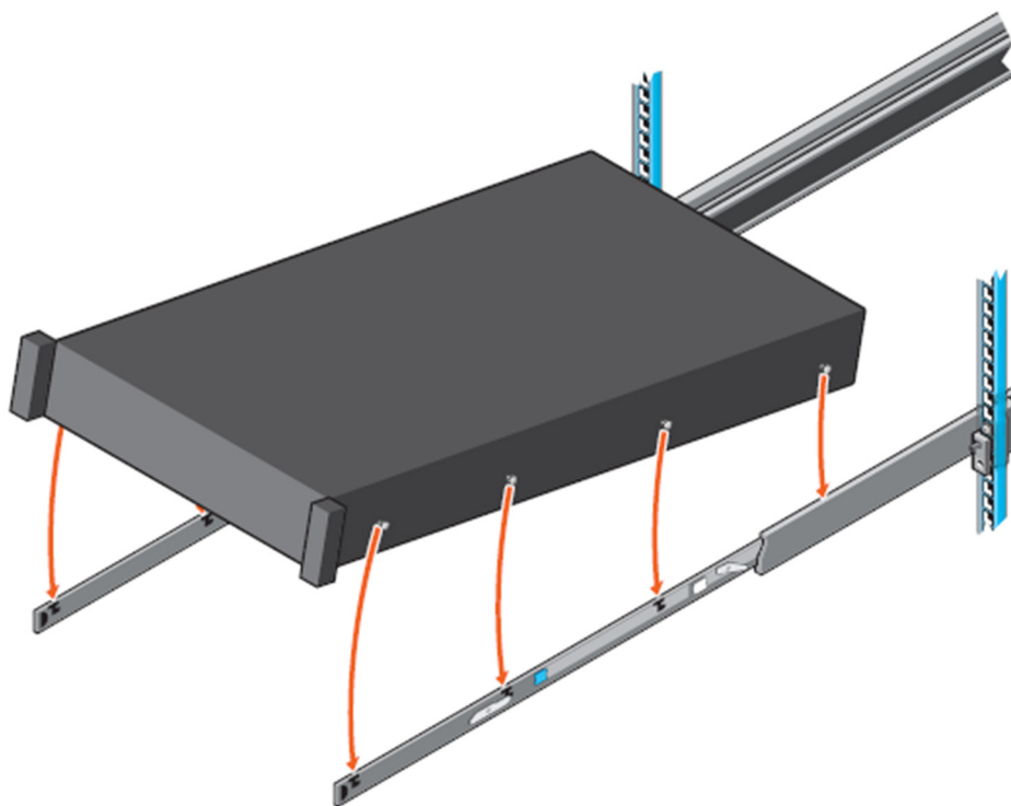
Figure 26. Insertion des fixations des rails dans les logements en J
