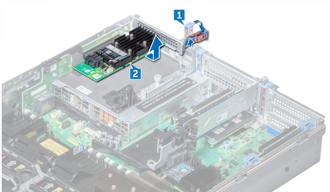
Figure 19. Retrait d'une carte d'extension de la carte de montage pour carte d'extension 3
