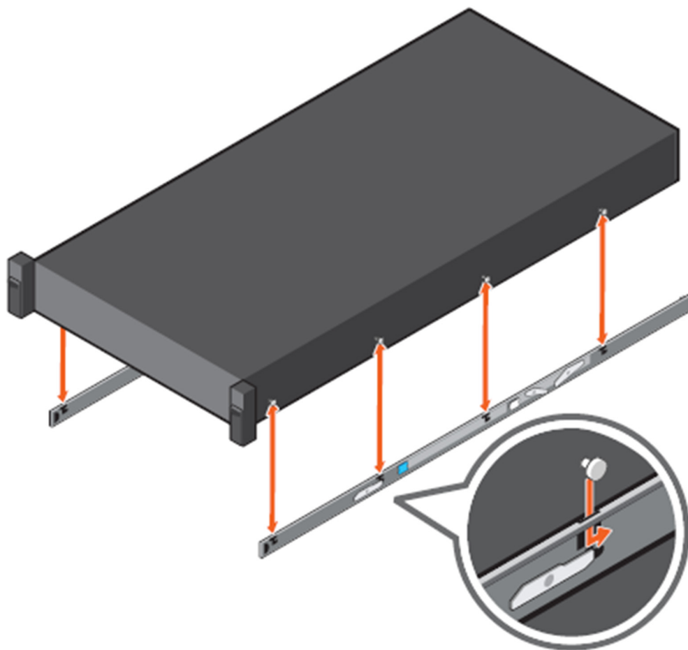
Figure 29. Fixation des rails internes sur le système
