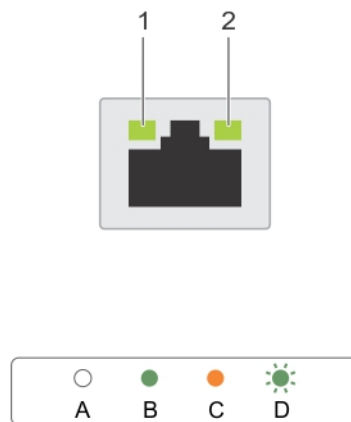
Figure 48. Voyants de carte réseau
