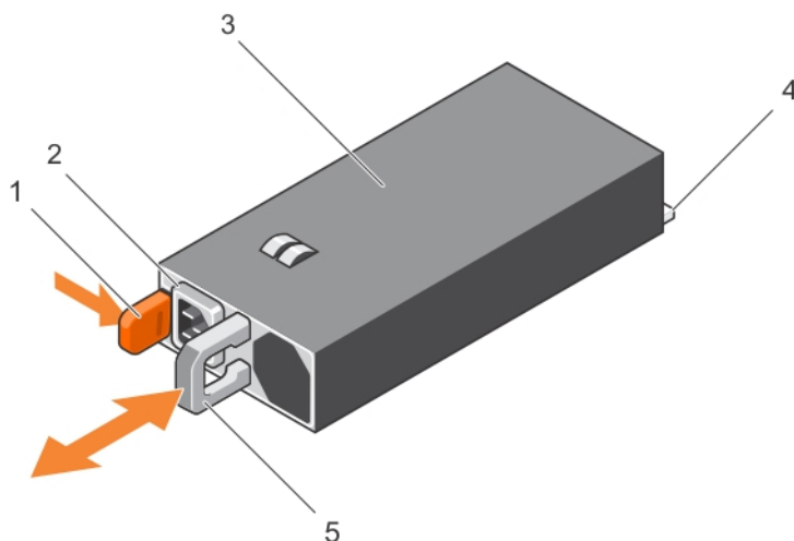
Figure 40. Retrait et installation d'un bloc d'alimentation en CA
