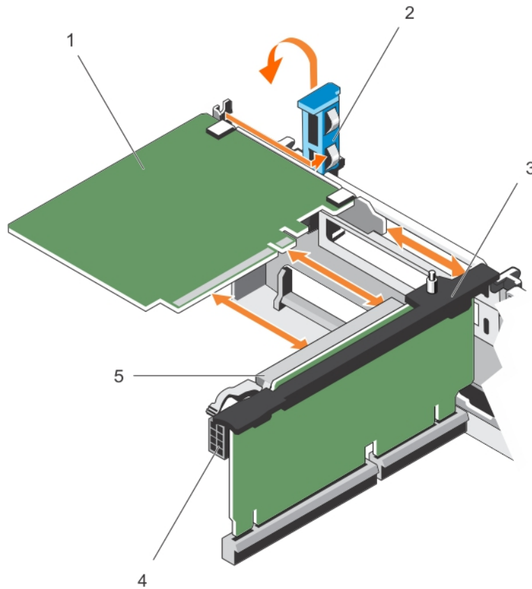
Figure 20. Retrait et installation d'une carte d'extension dans la carte de montage 2 ou 3 pour carte d'extension
