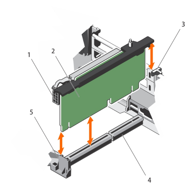
Figure 25. Retrait et installation de la carte de montage pour carte d'extension 2
