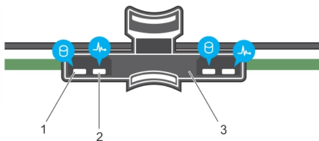
Figure 3. voyants des disques durs sur le fond de panier du plateau du disque dur
