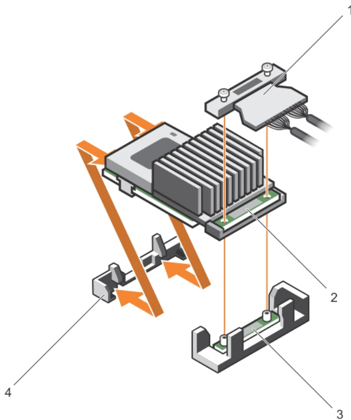
Figure 33. Retrait et installation de la carte contrôleur de stockage intégrée
