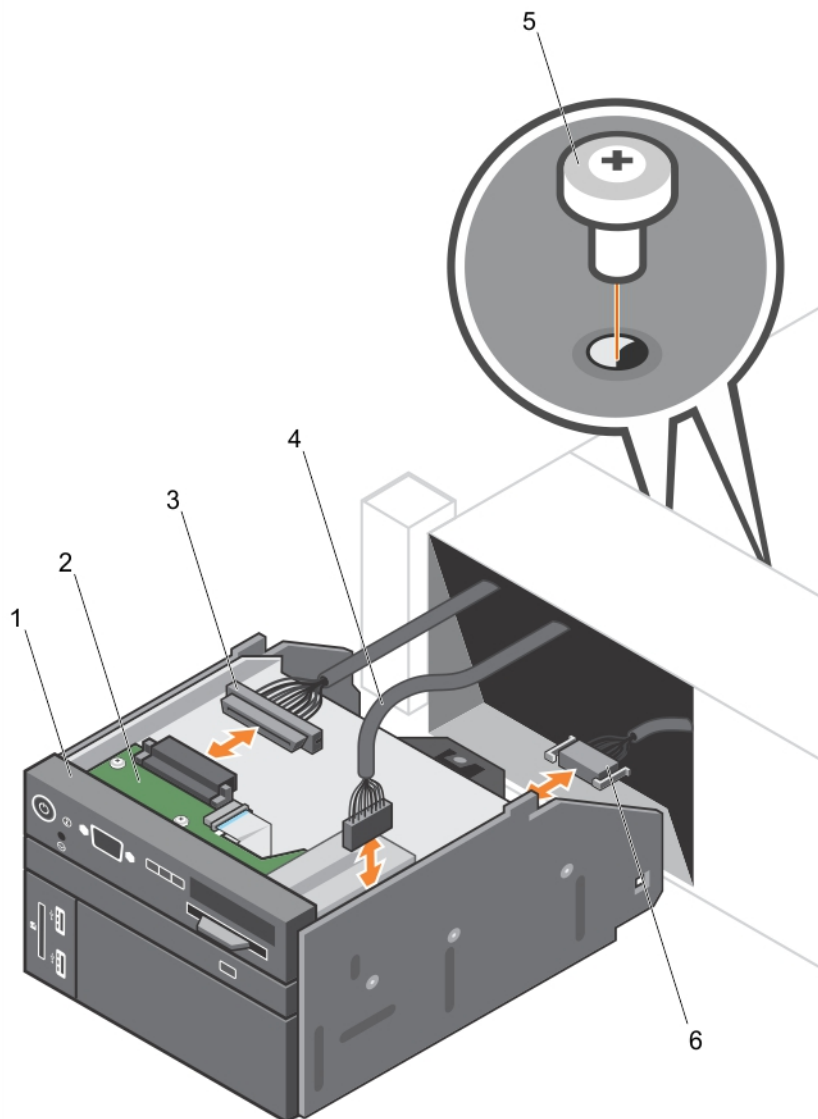
Figure 44. Retrait et installation du panneau de commande : système de disques durs de 2,5 pouces — PowerEdge R730
