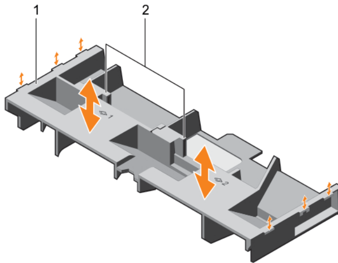
Figure 7. Retrait et installation du carénage de refroidissement
