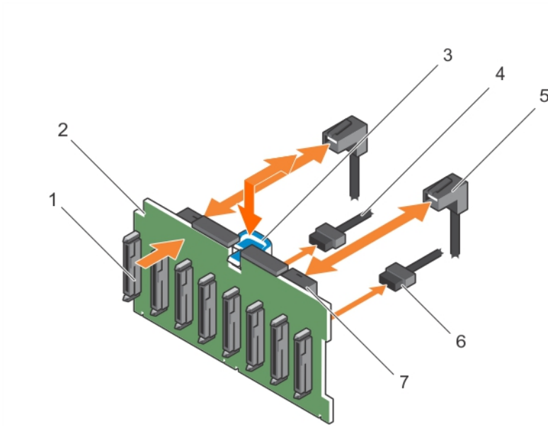
Figure 43. Retrait et installation du fond de panier de disque dur/SSD de 2,5 pouces (x8) : Precision Rack 7910
