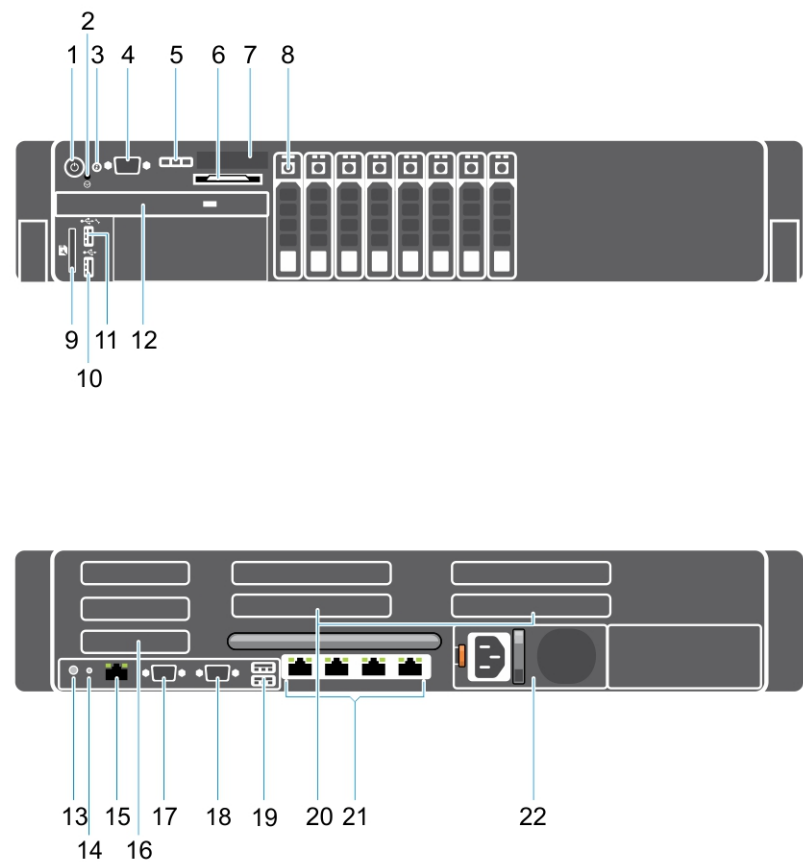
Figure 4. Vues avant et arrière
