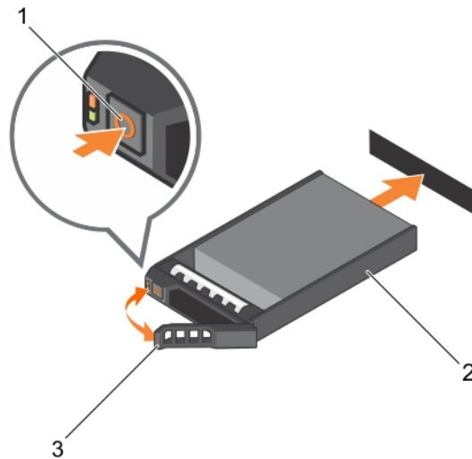
Figure 11. Retrait et installation d'un disque dur
