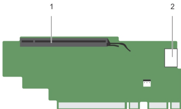
Figure 29. Identification des connecteurs de la carte de montage pour carte d'extension 3 (alternative).
