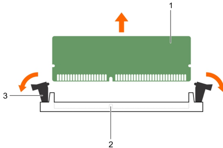
Figure 8. Retrait d'une barrette de mémoire
