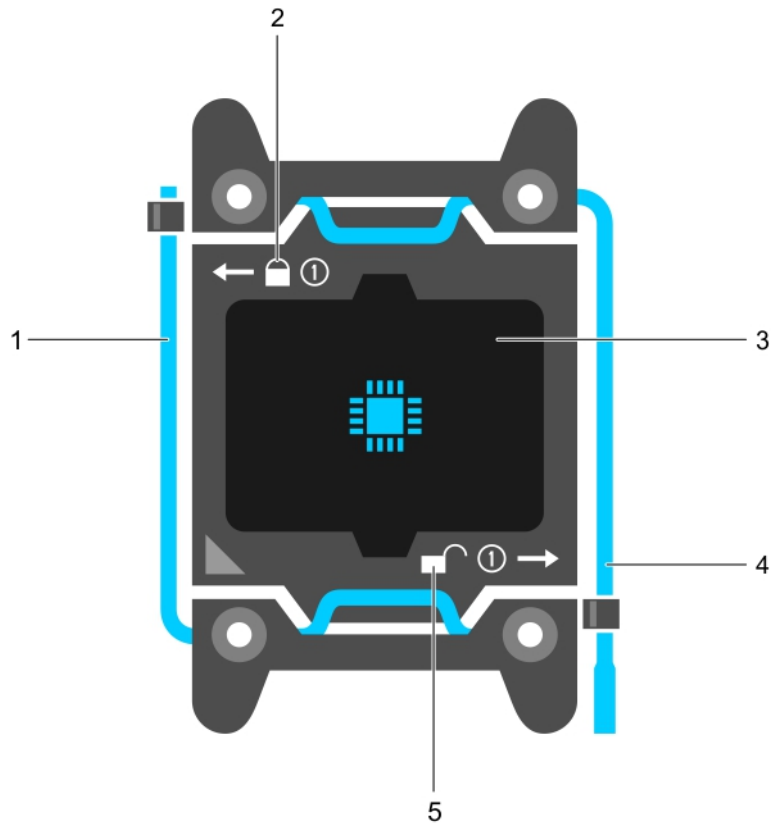
Figure 36. Protection du processeur
