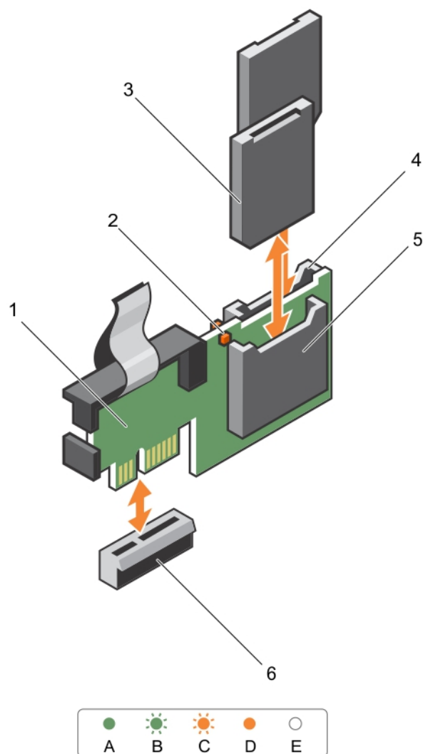
Figure 32. Retrait et installation du module SD interne double (IDSDM)
