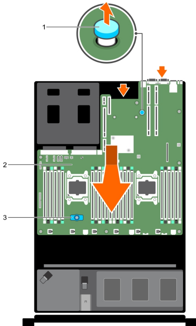
Figure 65. Retrait de la carte système
