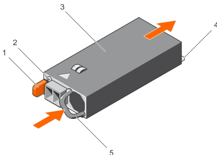
Figure 55. Installation d'un bloc d'alimentation en CC
