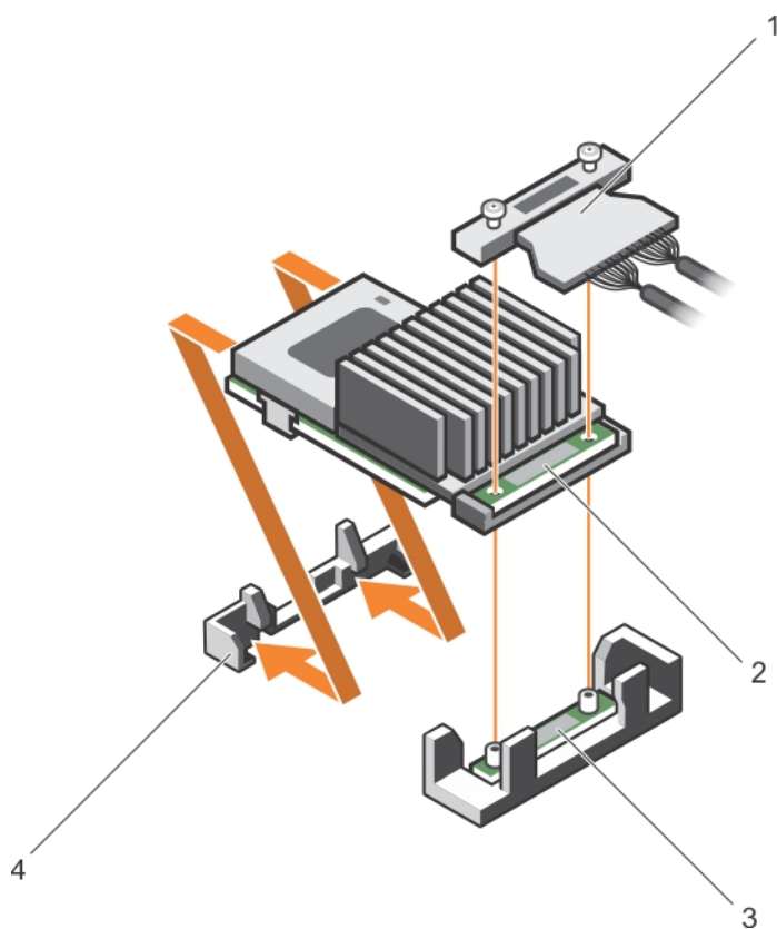
Figure 45. Installation de la carte contrôleur de stockage intégrée
