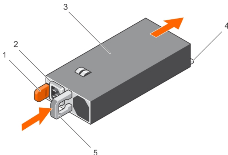
Figure 53. Installation d'un bloc d'alimentation en CA
