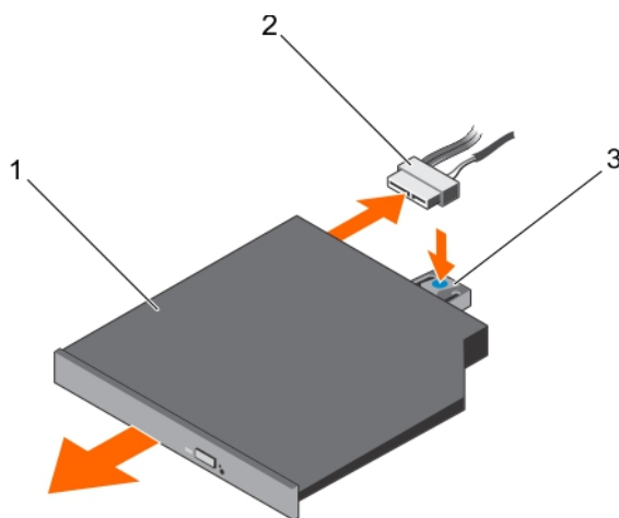
Figure 28. Retrait du lecteur optique en option
