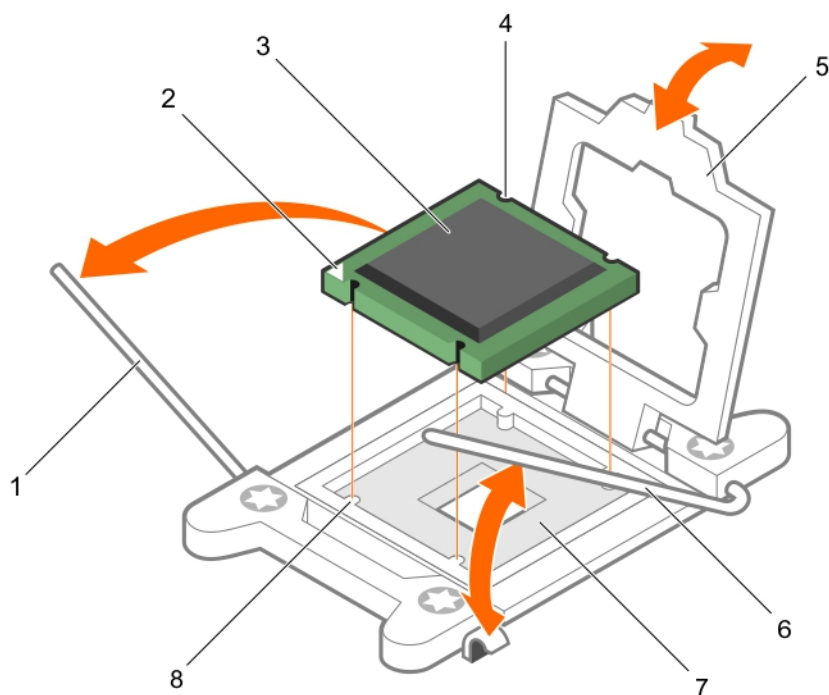
Figure 49. Retrait et installation d'un processeur
