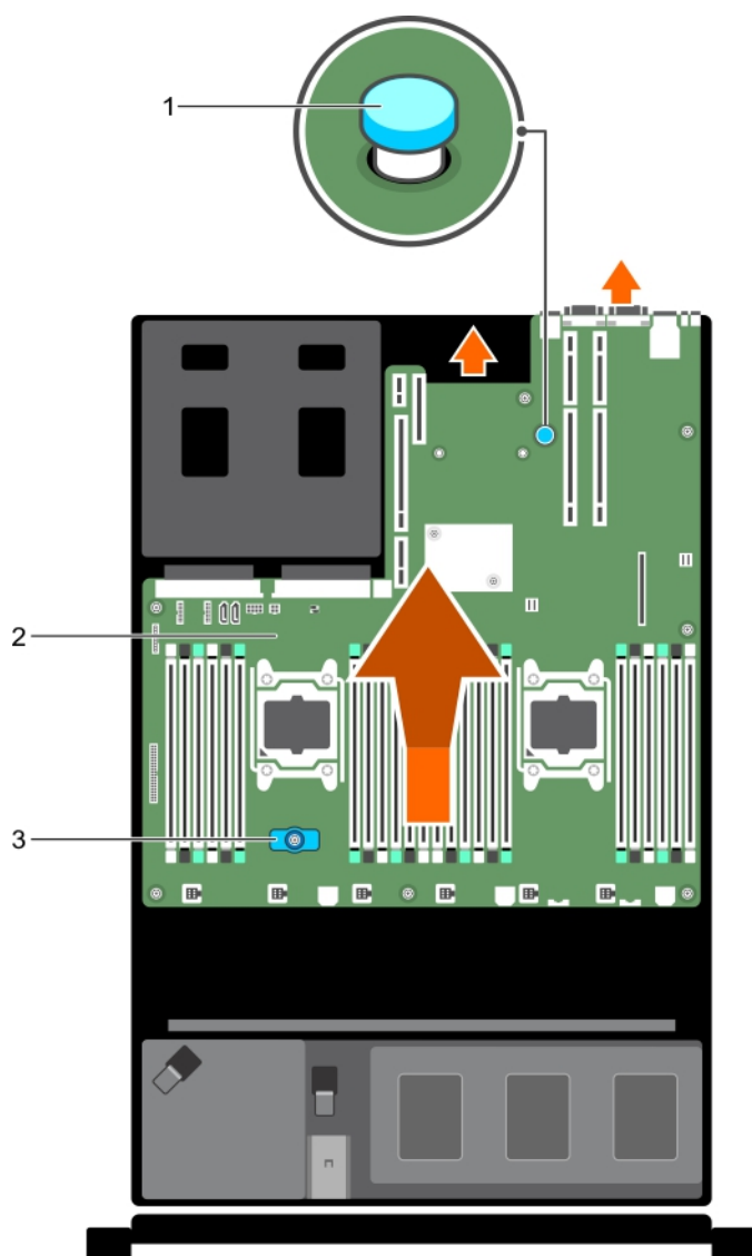
Figure 66. Installation de la carte système
