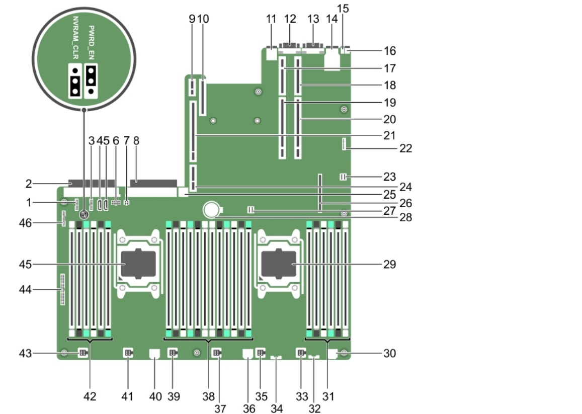
Figure 68. Connecteurs et cavaliers de la carte système
