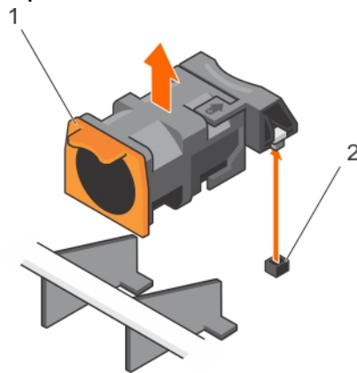
Figure 32. Retrait d'un ventilateur de refroidissement
