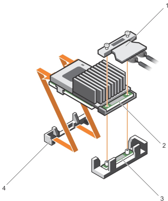
Figure 44. Retrait de la carte contrôleur de stockage intégrée
