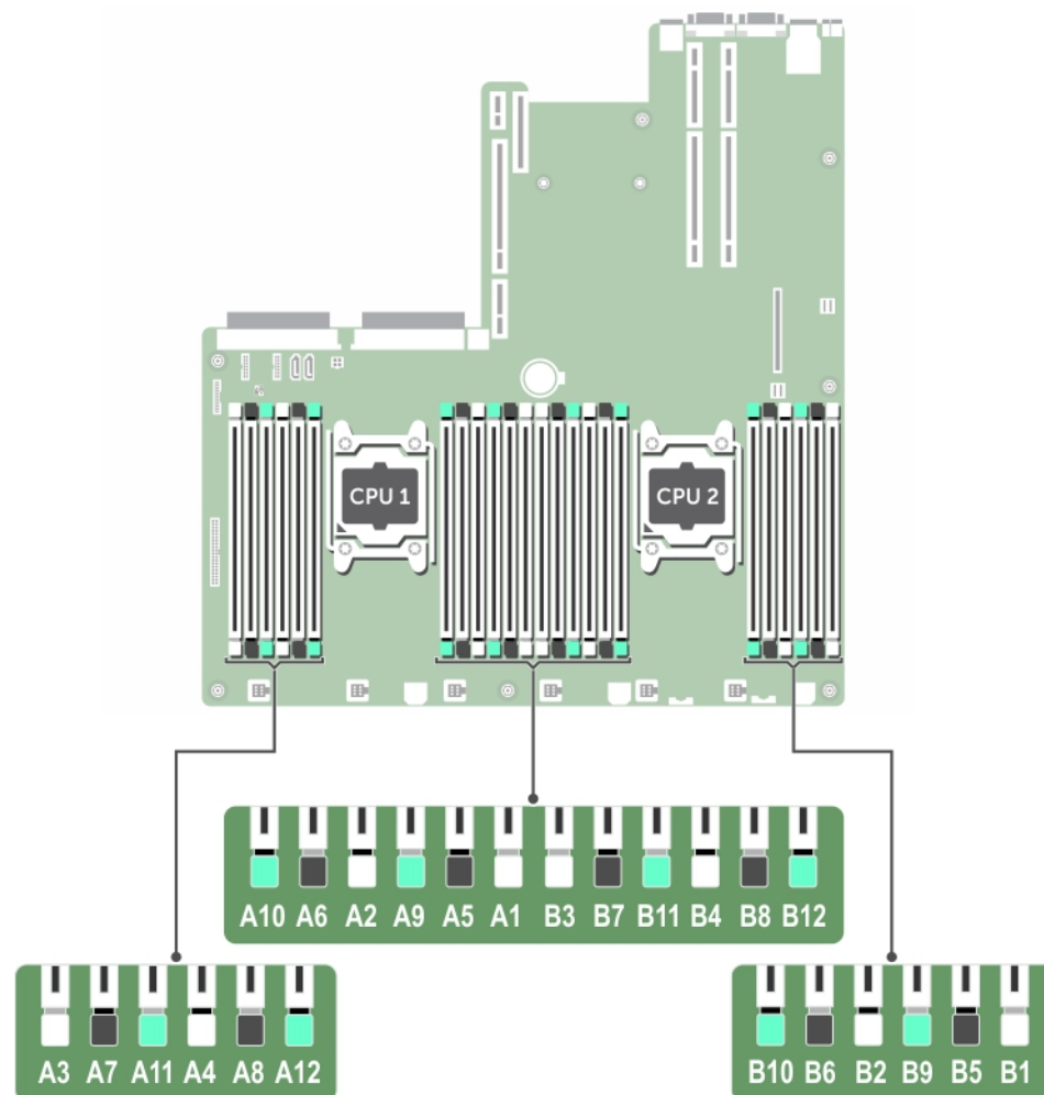
Figure 19. Emplacement des supports de mémoire
