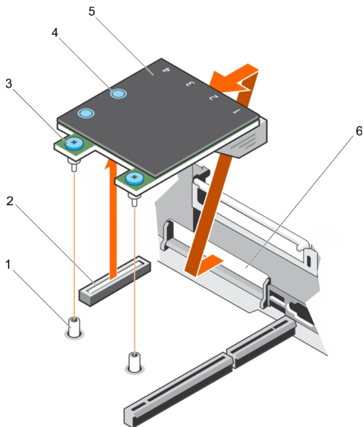
Figure 46. Retrait de la carte NDC
