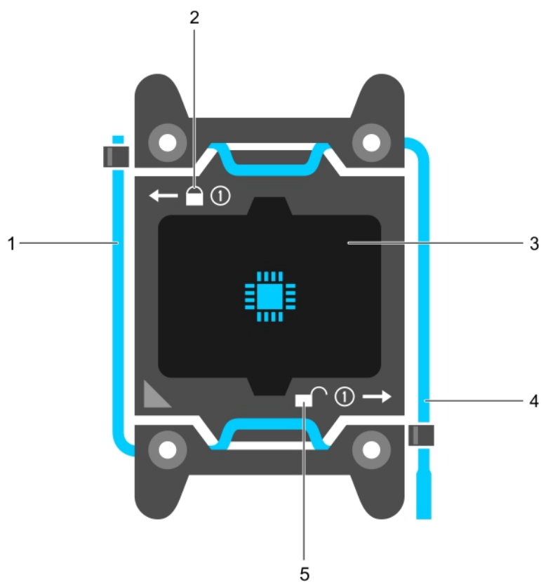
Figure 48. Protection du processeur
