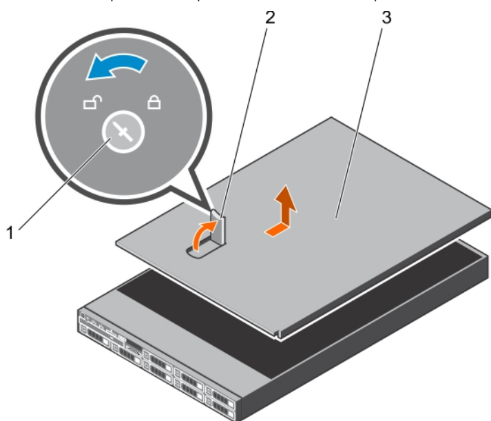
Figure 15. Retrait du capot du système
