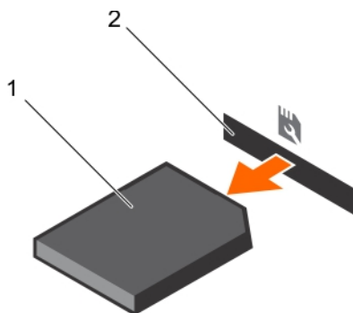
Figure 25. Retrait et installation de la carte SD vFlash
