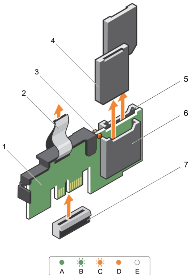
Figure 27. Retrait du module SD interne double (IDSDM)
