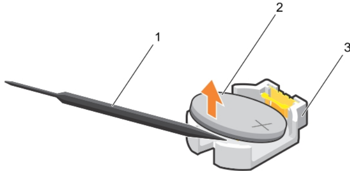
Figure 33. Retrait de la pile du système
