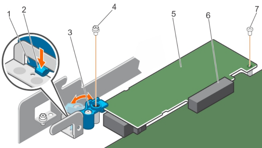
Figure 23. Ouverture et fermeture du verrou de la carte PERC
