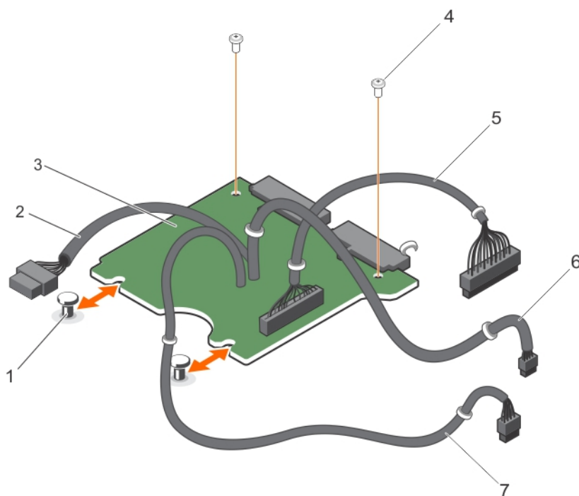
Figure 39. Retrait et installation de la carte intercalaire d'alimentation
