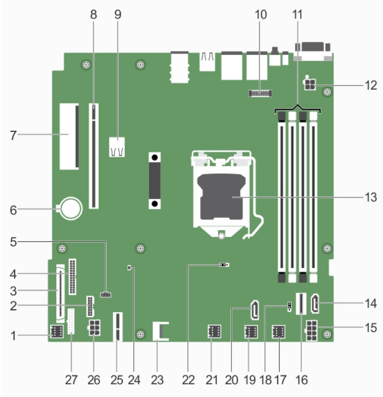
Figure 42. Connecteurs de la carte système
