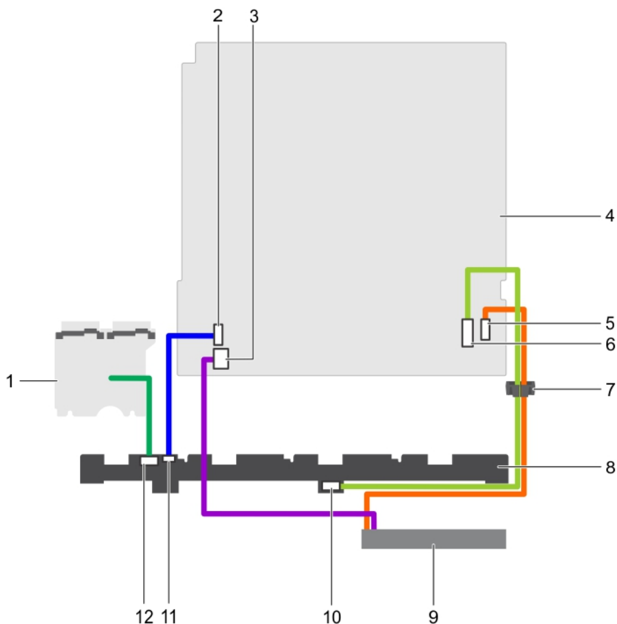
Figure 36. Schéma de câblage : fond de panier des quatre disques durs de 3,5 pouces
