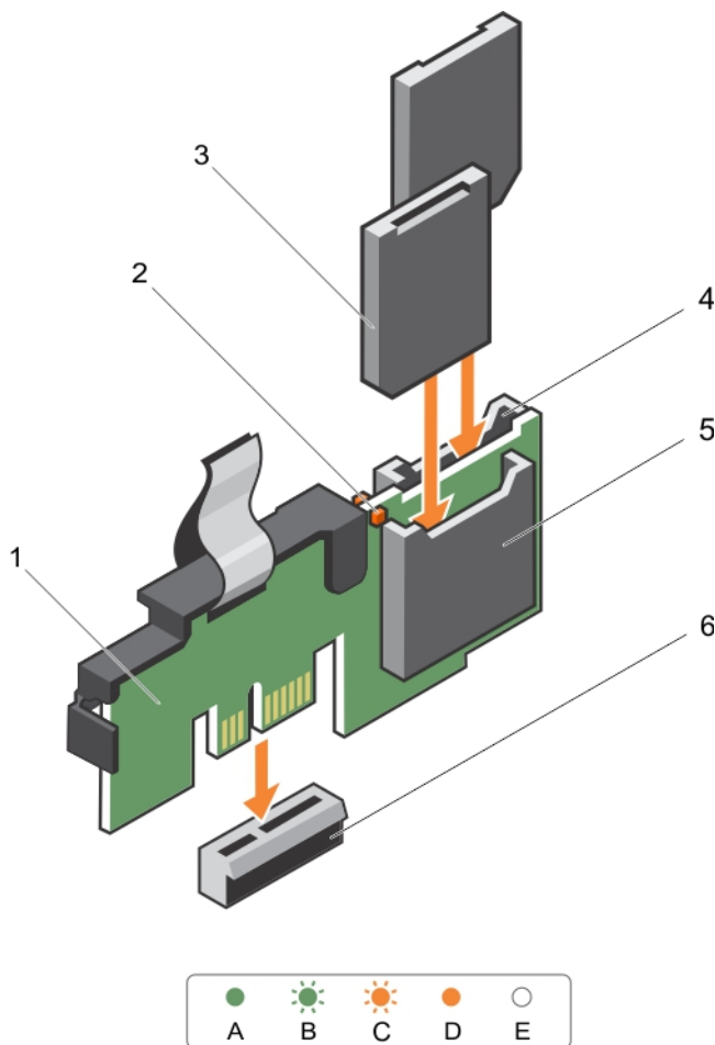
Figure 28. Installation du module SD interne double en option
