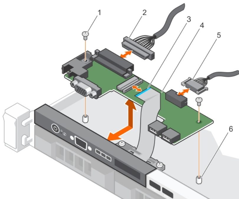
Figure 38. Retrait et installation de la carte du panneau de commande LCD module de panneau de commande – châssis à quatre disques durs
