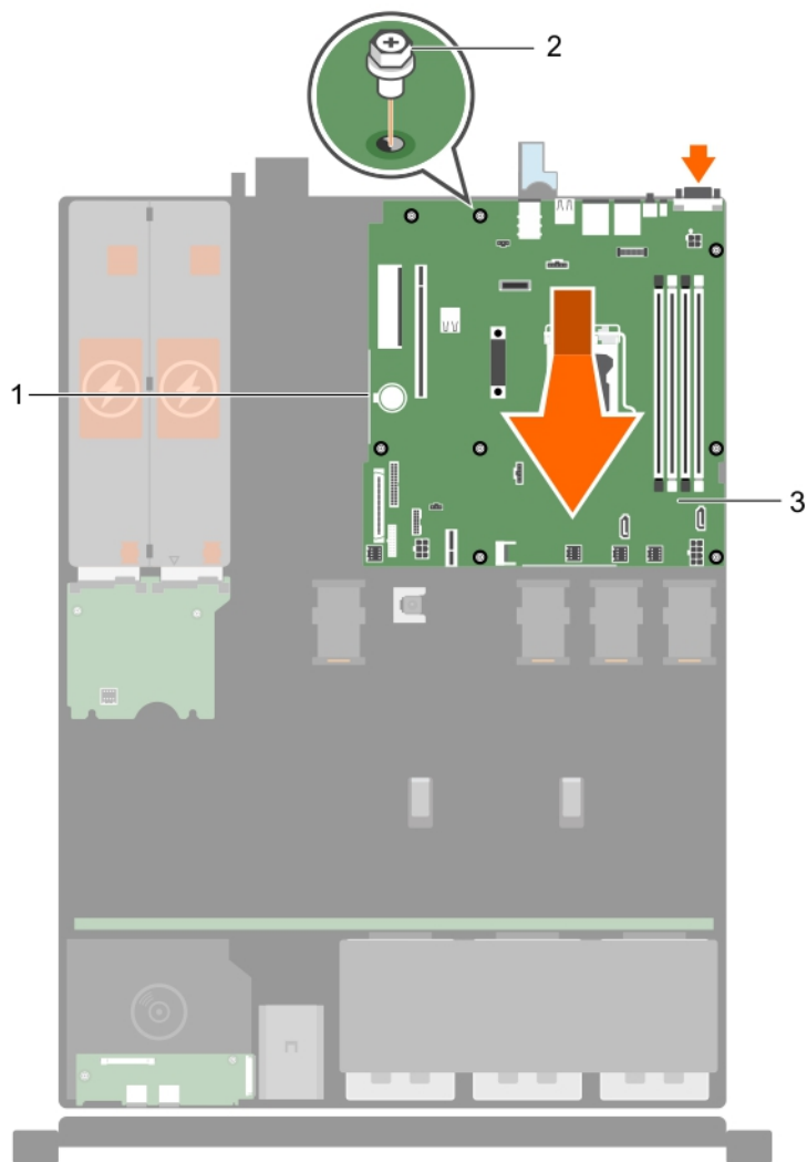
Figure 41. Retrait et installation de la carte système
