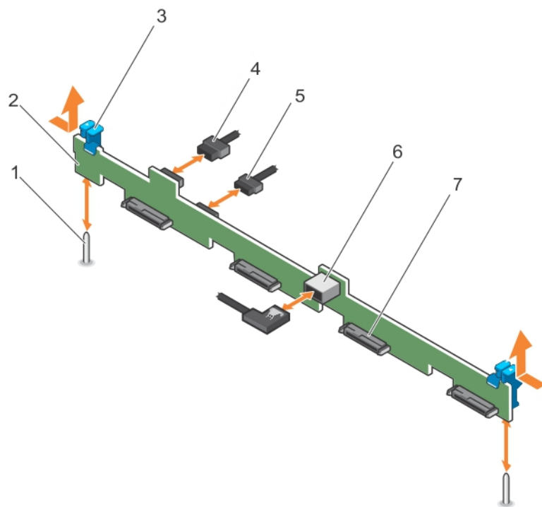
Figure 35. Retrait et installation du fond de panier des quatre disques durs de 3,5 pouces
