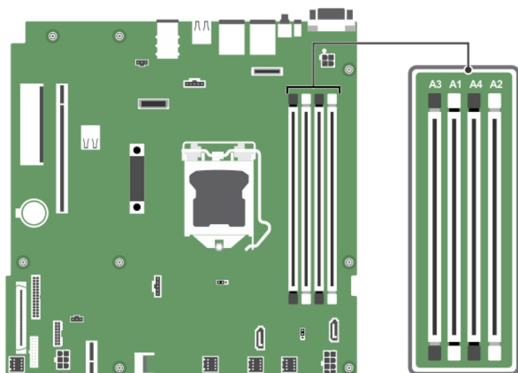
Figure 12. Emplacements des supports de mémoire sur la carte système
