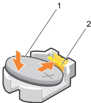
Figure 34. Installation de la pile du système
