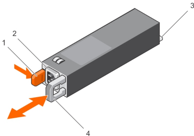
Figure 31. Retrait et installation d'un bloc d'alimentation redondant
