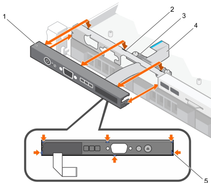
Figure 37. Retrait et installation du panneau de commande LCD – châssis de quatre disques durs 3,5 pouces remplaçables à chaud
