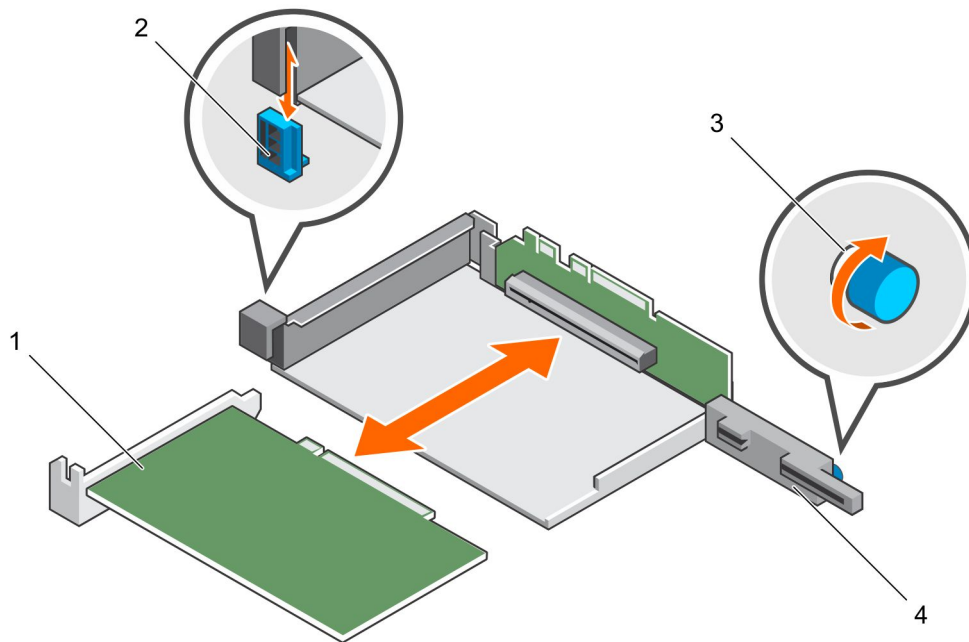
Figure 18. Installation d'une carte d'E/S dans la carte de montage 1
