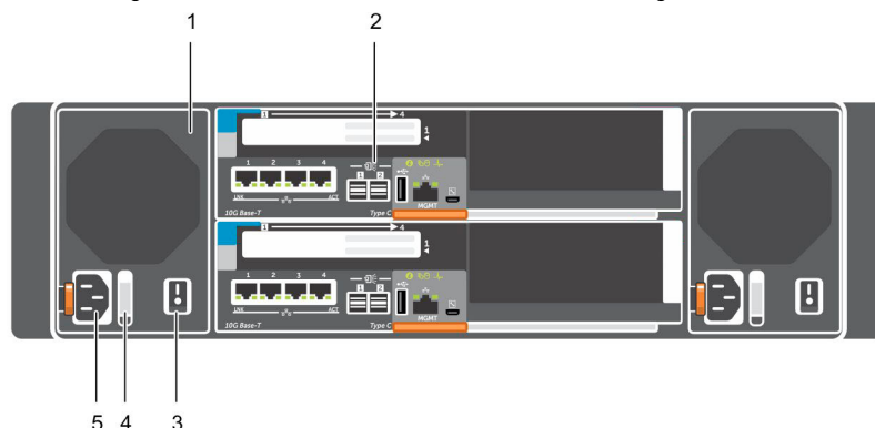
Figure 2. Vue du panneau arrière du Système de stockage SC5020 Series
