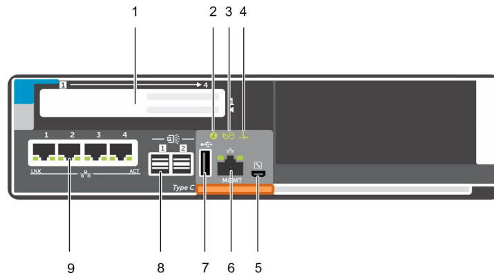
Figure 5. Contrôleur de stockage Série SC5020
