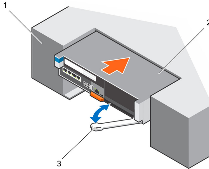
Figure 11. Retrait et installation d'un Contrôleur de stockage
