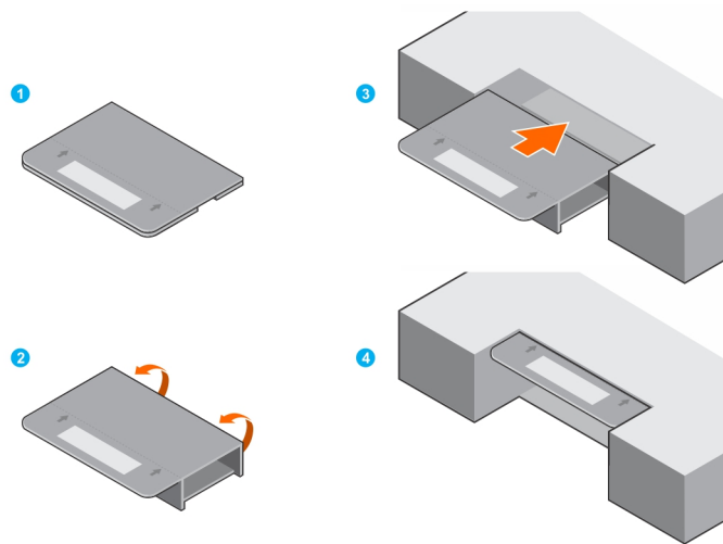
Figure 10. Installation du déflecteur de maintenance
