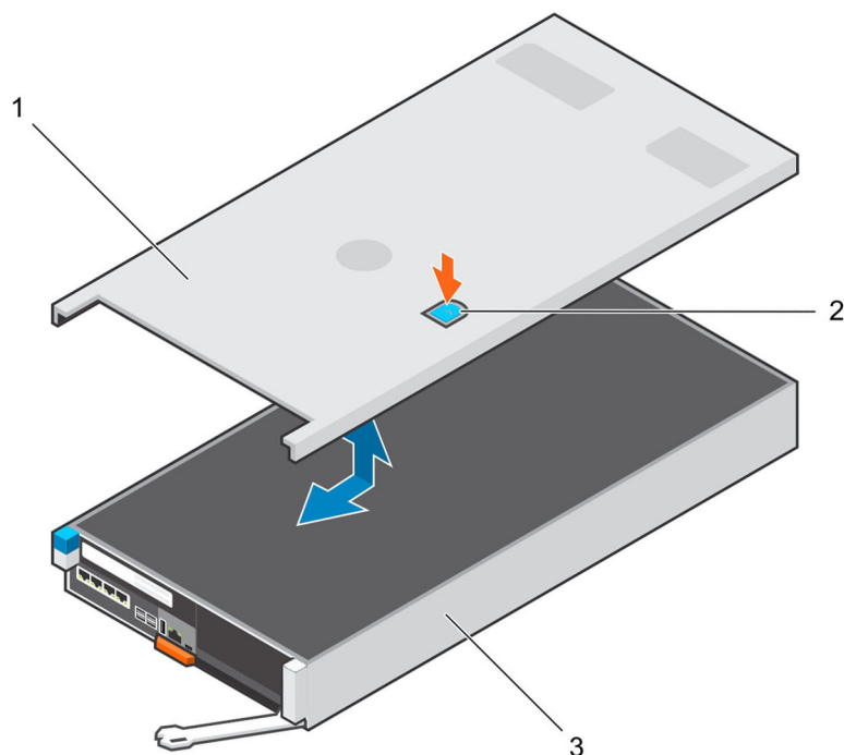
Figure 12. Retrait et installation du capot du Contrôleur de stockage
