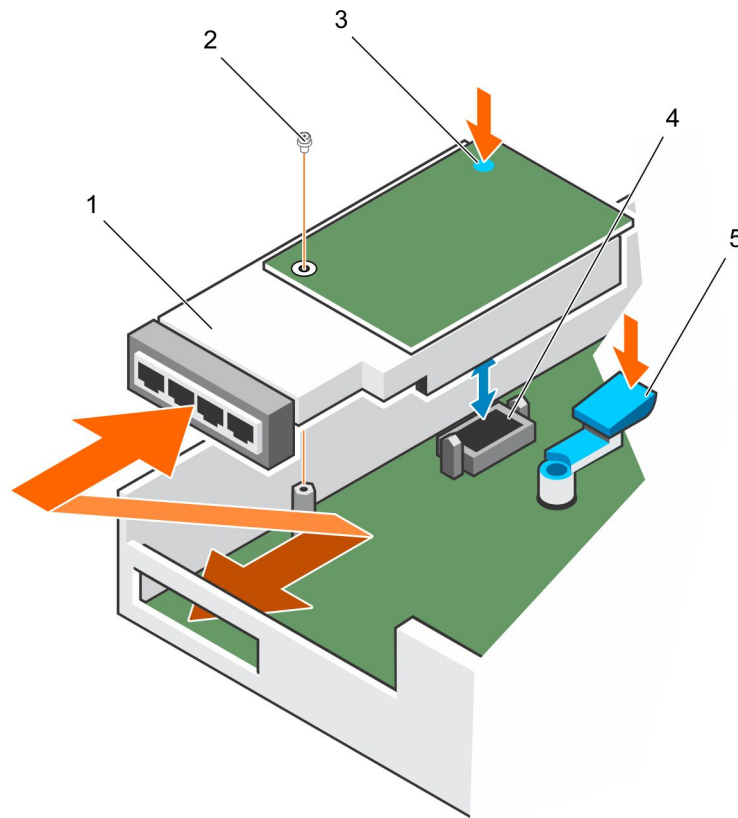
Figure 20. Installation de la carte mezzanine
