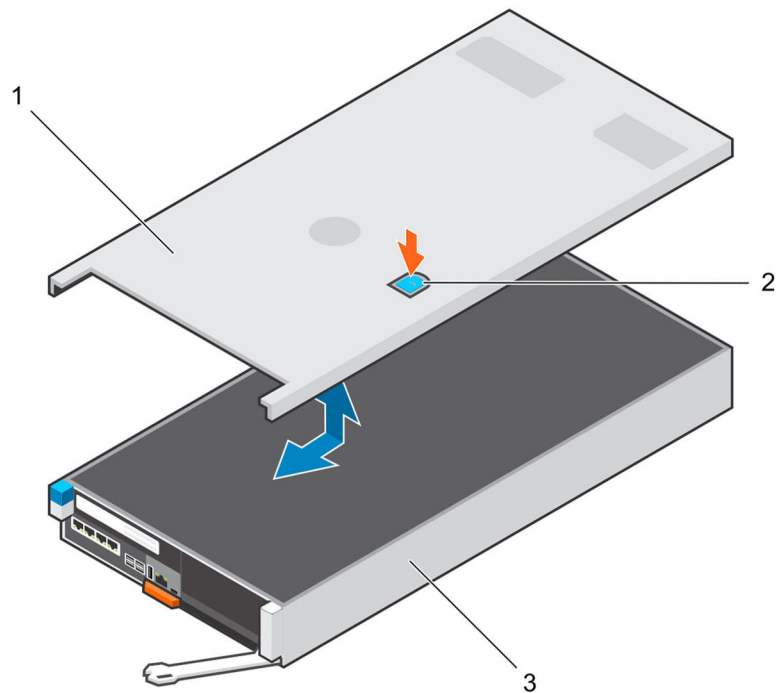
Figure 13. Retrait du capot du Contrôleur de stockage
