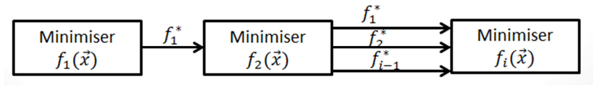
Figure IV-10 Méthode lexicographique
