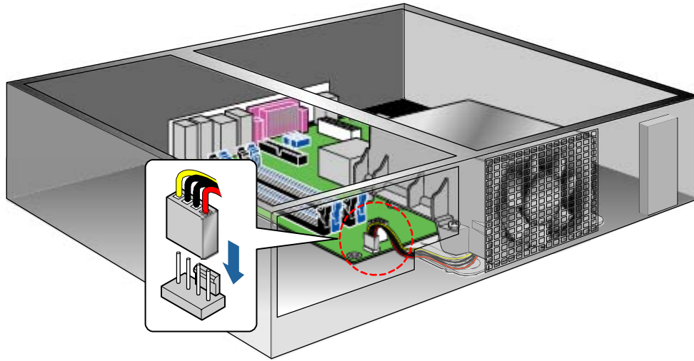
Figure 15. Connect the Thermal Module Fan Cable
