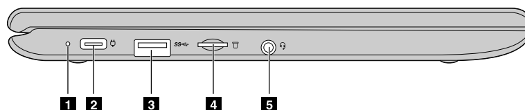
Figure 2. 500e Chromebook - vue du côté gauche
