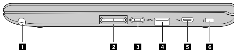
Figure 4. Chromebook 500e - vue du côté droit
