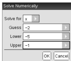
Numerisk OS
