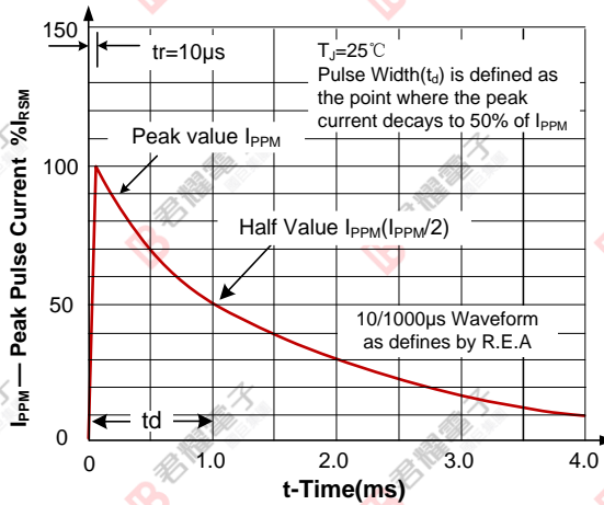
图 6 10/1000μs 电流波形
