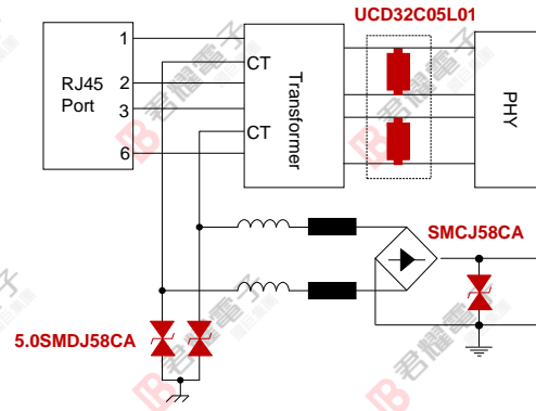
图 7 100M PoE 接口保护
