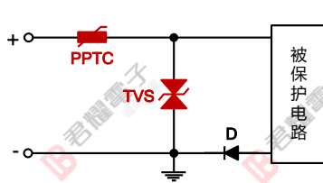
图 3 直流电源保护
