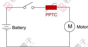
图 5 电机保护
