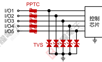
图 4 I/O 接口保护
