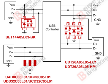
图 2 USB2.0 接口保护
