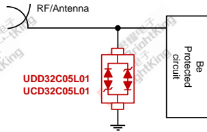
图 7 天线 (射频) 接口 ESD 保护
