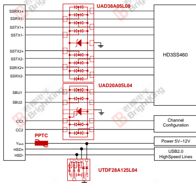
图 3 USB type-C 接口保护
