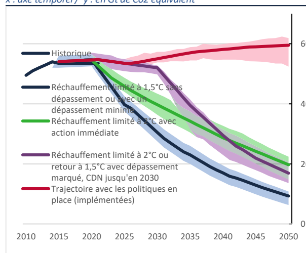
Graphique 1.62 : Évolutions des émissions de GES selon les trajectoires x : axe temporel / y : en Gt de CO2 équivalent
