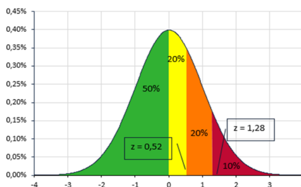
Graphique 4.4 : Densité de probabilité d'une loi normale centrée réduite autour de 0
