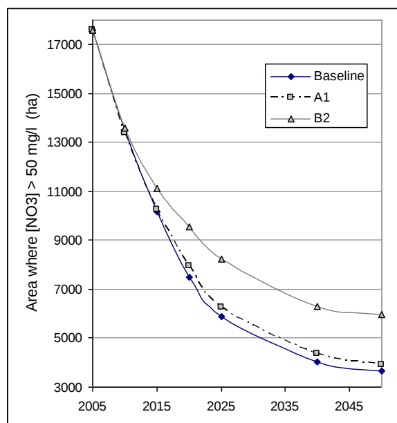
Figure 14 : Evolution des surfaces affectées par la pollution par les nitrates avec 3 scénarios.
