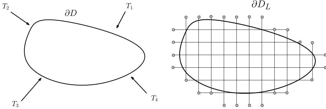
FIGURE 2.7 – Un domaine D \subset \mathbb{R}^2 avec différentes températures imposées sur son bord \partial D . Le maillage de D induit une frontière discrète \partial D_L représentée par les sites gris.
