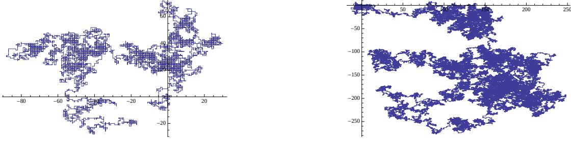
FIGURE 4.3 – Deux réalisations de la marche aléatoire dans \mathbb{Z}^2 pour 10^4 et 10^5 pas.
