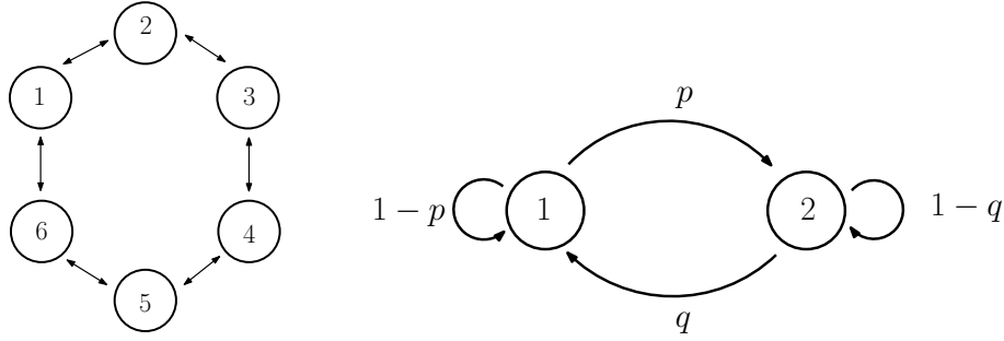
FIGURE 3.1 – À gauche, le graphe des transitions associé à la marche aléatoire symétrique sur le domaine périodique \{1, \dots, 6\} . Le graphe des transitions pour la chaîne à deux états est représenté à droite.
