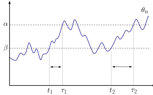
FIGURE 12.8 – La suite \{\theta_n\}_{n \geq 0} est représentée et les intervalles de temps [t_1, \tau_1] , [t_2, \tau_2] correspondent au dernier passage au dessus du niveau \beta avant d'atteindre le niveau \alpha .
