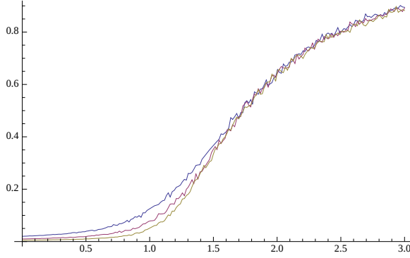
FIGURE 4.7 – Densité moyenne de la composante connexe maximale d'un graphe aléatoire d'Erdős-Rényi pour trois valeurs de N = 50, 100, 200 et \lambda variant entre 0 et 3.
