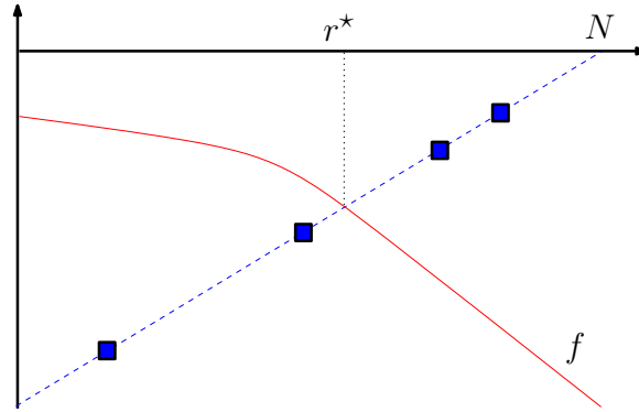
FIGURE 13.2 – Les graphes de n \rightarrow f(N - n) et de n \rightarrow -(N - n) sont représentés. Les carrés marquent les positions n des places disponibles ( \xi_n = 0 ) et le gain correspondant est -(N - n) . Le seuil r^* est le point où les deux graphes s'intersectent. La place choisie est la première place libre après r^* , i.e. le troisième carré sur le schéma.
