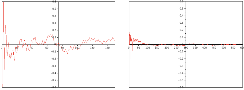
FIGURE 12.7 – L’algorithme de Robbins-Monro est utilisé dans ces 2 simulations pour résoudre la récurrence aléatoire \theta_{n+1} = \theta_n + \gamma_n(-\arctan(\theta_n) + X_n) où X_n sont des variables aléatoires uniformément distribuées sur [-1, 1] . La simulation représentée à gauche est réalisée avec \gamma_n = \frac{1}{n^{0.7}} pour 150 pas de temps. La série \theta_n s’approche de la solution \theta^* = 0 en oscillant. La convergence est améliorée sur la simulation de droite réalisée avec \gamma_n = \frac{1}{n} pour 600 pas de temps.
