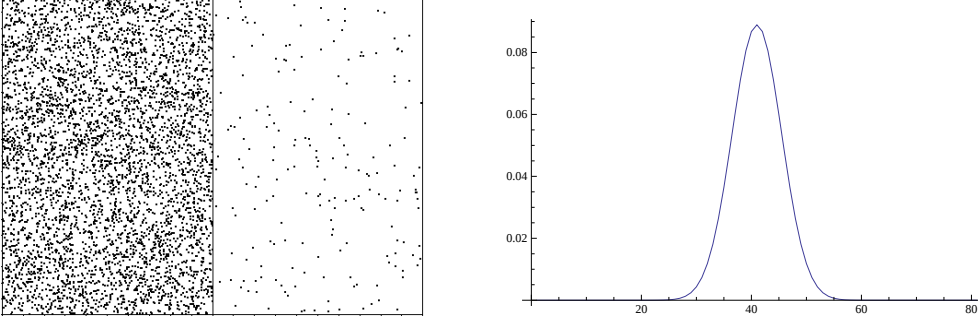
FIGURE 3.3 – Sur le schéma de gauche, le modèle d'Ehrenfest est représenté : le compartiment de gauche est rempli de molécules, celui de droite est presque vide. Un passage est ouvert entre les deux compartiments pour permettre le transfert des molécules. Le graphe de droite représente la distribution de \pi pour K = 80 . Cette distribution est symétrique autour de sa moyenne et elle décrit l'état d'équilibre du gaz.
