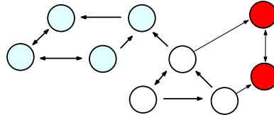
FIGURE 3.2 – Dans ce graphe de transition, on distingue 2 classes irréductibles fermées en rouge et en bleu clair. Aucun site de ces deux classes ne communique avec les sites blancs qui ne forment pas une classe fermée. La chaîne de Markov peut être restreinte à chacune des classes irréductibles.
