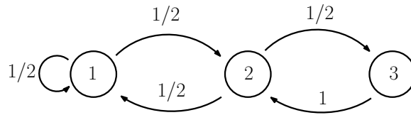
FIGURE 6.6 – Pour ce graphe de transition, l'équilibre ne peut pas correspondre au moment où les différentes trajectoires fusionnent. En effet, l'état 3 ne peut être atteint qu'en venant de l'état 2 et il n'est donc pas possible que les trajectoires se touchent pour la première fois à l'état 3.
