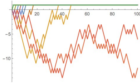
FIGURE 10.2 – Cette simulation représente 30 réalisations de marches aléatoires arrêtées au niveau 1. Après 100 pas, seules 2 marches n'ont pas atteint le niveau 1 mais leurs valeurs sont très négatives. Ces rares fluctuations permettent d'expliquer le comportement asymptotique (10.11).
