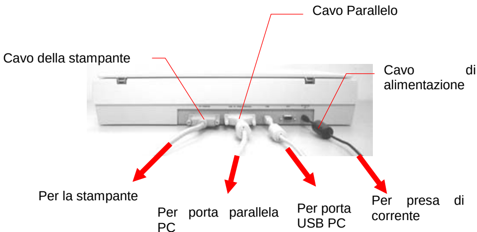
Figura 5.1 SC-215 Collegamento dei Cavi
