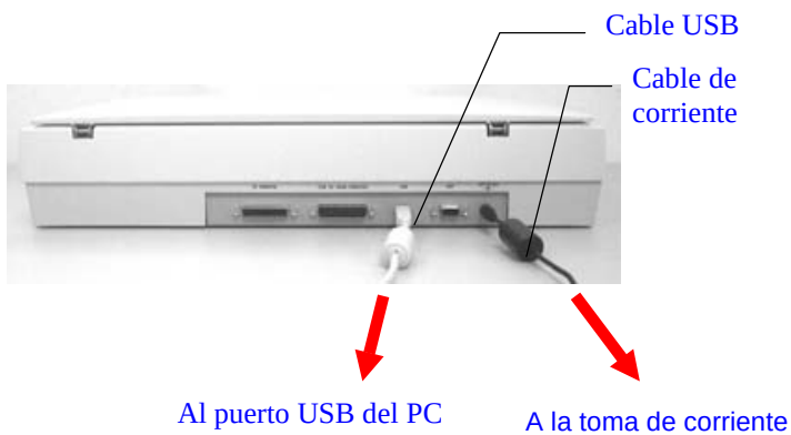
Figura 2-3 SC-215 conexión de cables
