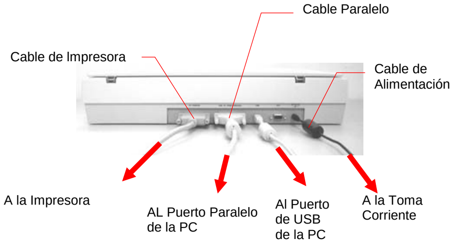
Figura 5.1 Conexión del Cable de SC-215
