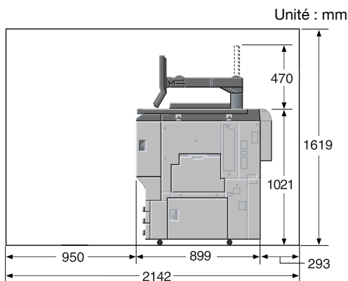
Machine + OC-506 + OT-502 (vue latérale)
