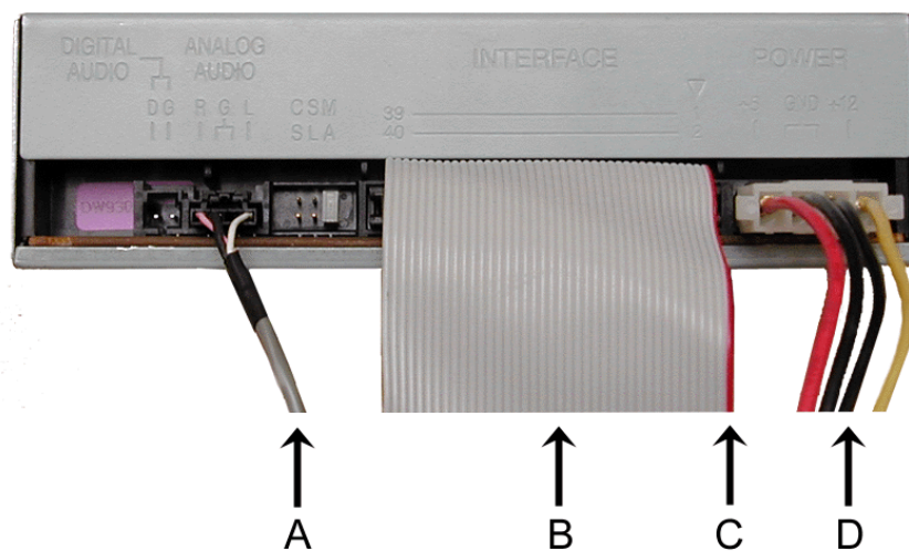
Figure 99: Câblage d'un périphérique optique IDE
