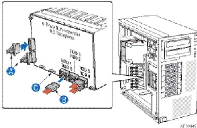
Figure 80: Branchement du panier de six disques durs 'hot-swap' SAS/S-ATA Fond de panier sans expenseur
