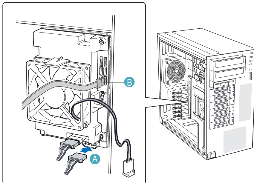
Figure 78: Câblage du panier de disque dur 'hot-swap' SAS/S-ATA
