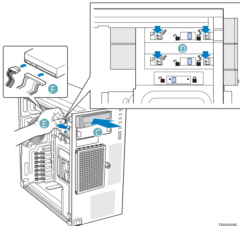
Figure 50: Installation d'un lecteur de disque optique
