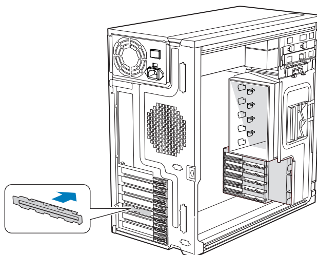
Figure 96: Remettre le cache d'emplacement PCI
