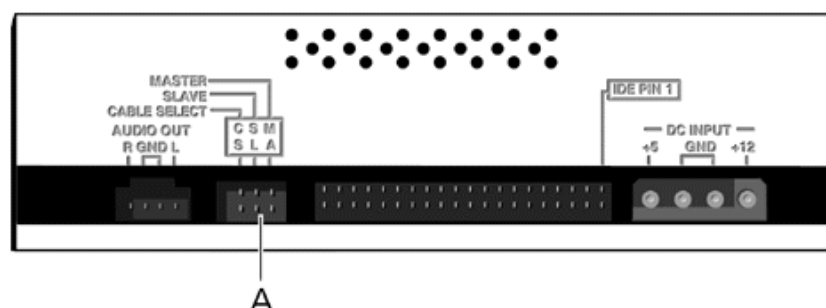
Figure 107: Connecteurs situés au dos d'un lecteur optique (exemple)
