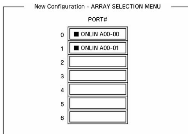
Illustration 38: Écran New Configuration - Array Selection Menu
