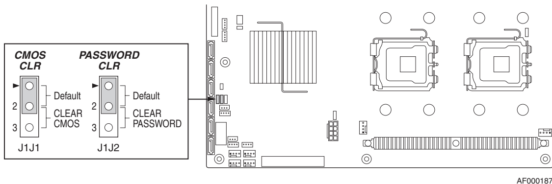
Figure 9: Cavalier de suppression des mots de passe
