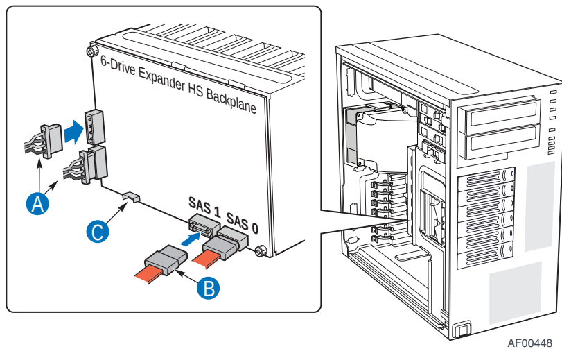
Figure 81: Branchement du fond de panier de six disques durs 'hot-swap' avec expasseur (support de ventilateur non représenté pour plus de clarté)
