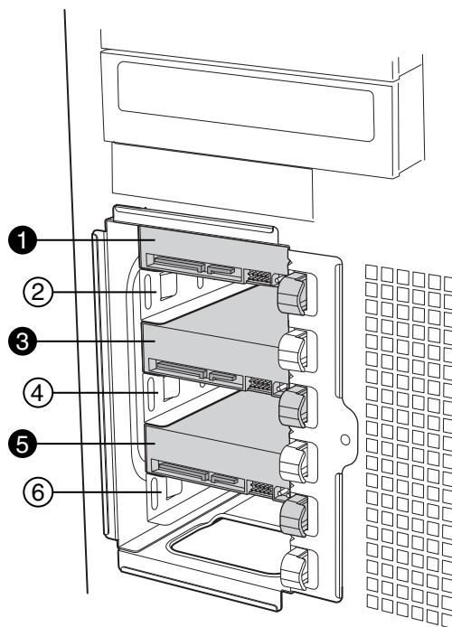
Figure 53: Ordre des emplacements de la baie (disques SAS/S-ATA représentés)
