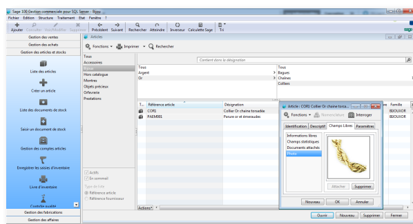
Sage 100 Gestion Commerciale i7 : Gestion de la base article
